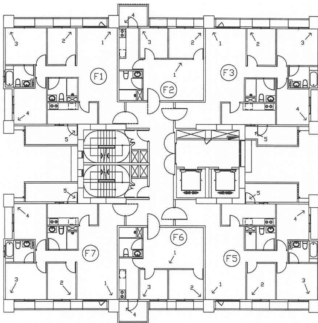
(A6區)F棟 8層平面圖
