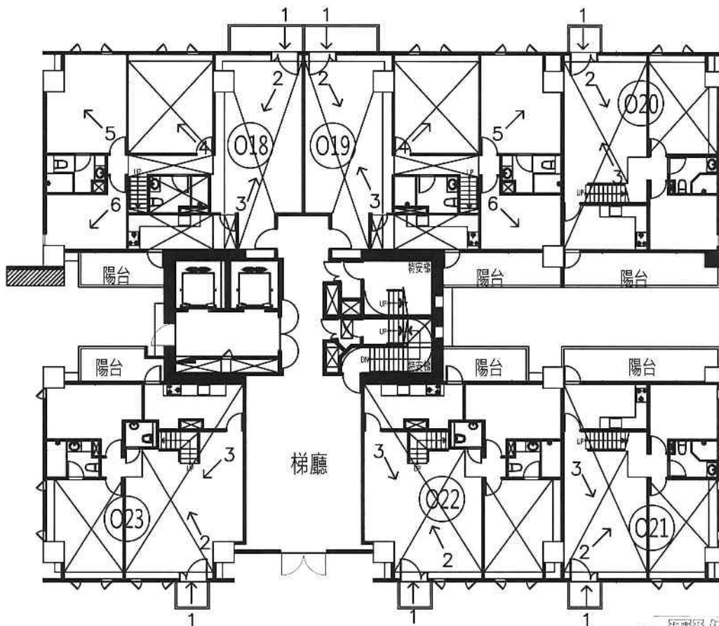
A6區E棟1層照片平面位置示意圖
