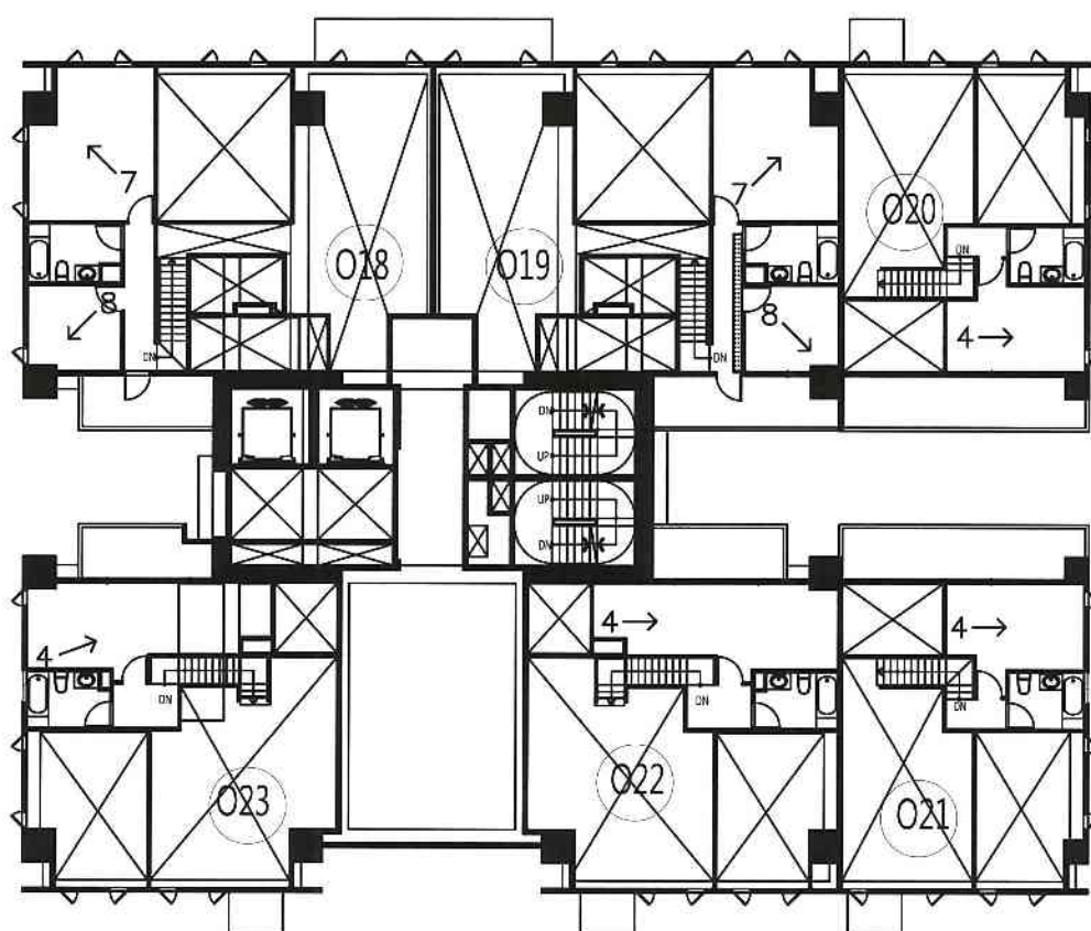
A6區E棟1夾層照片平面位置示意圖
