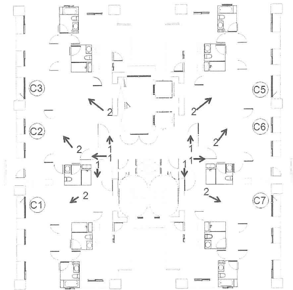
A6 區 C 棟 21 層照片平面位置示意圖
