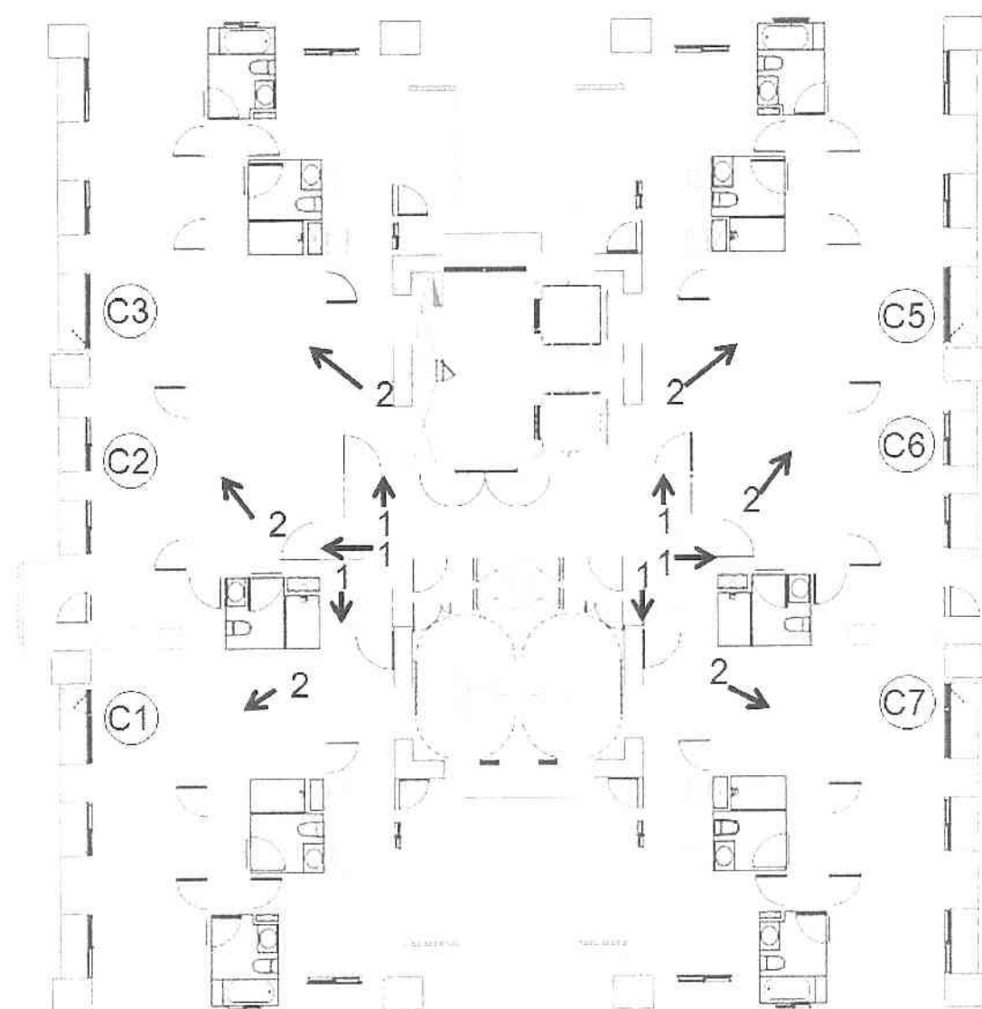
A6 區 C 棟 23 層照片平面位置示意圖
