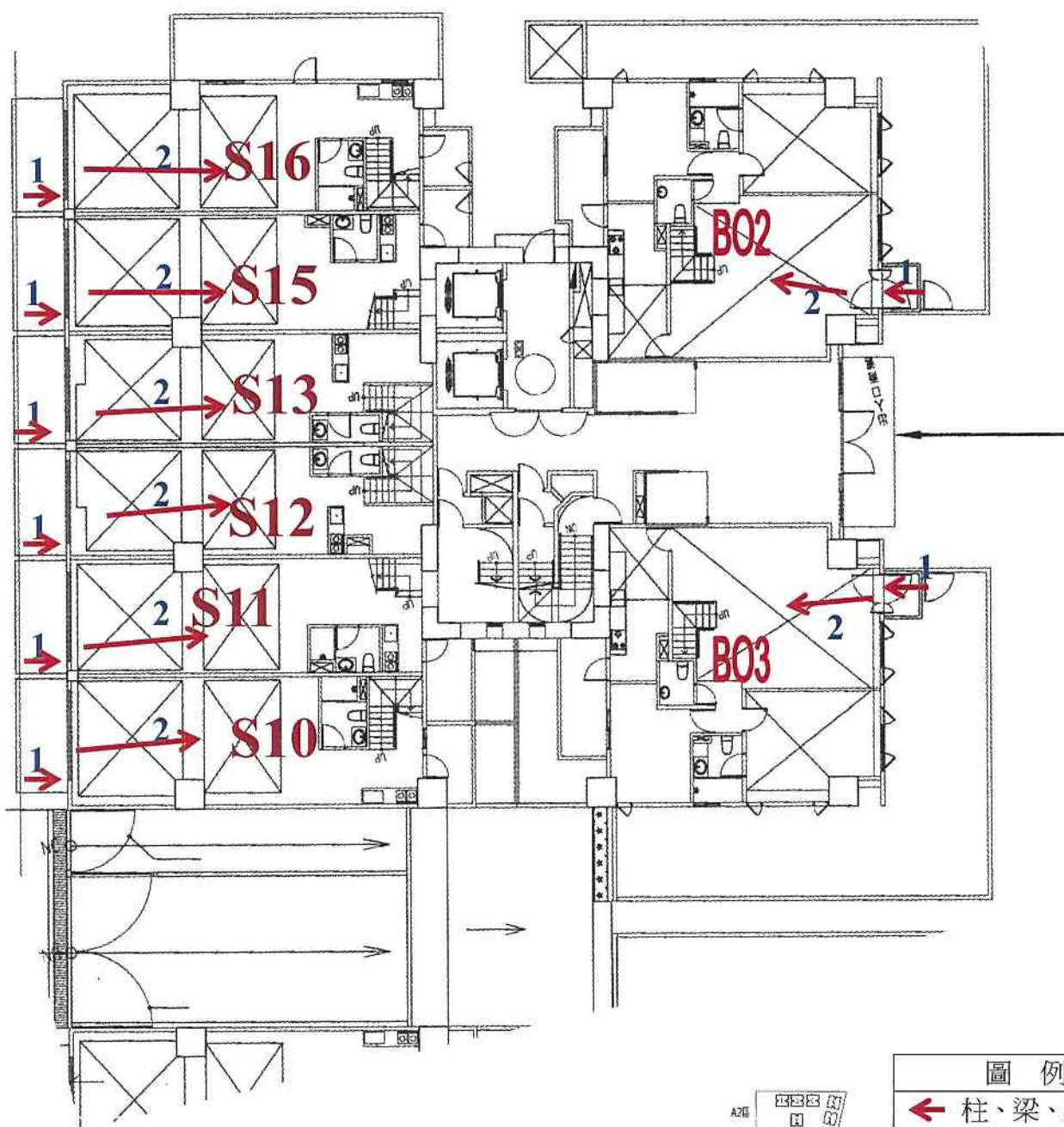
A6 區 B 棟 1 層照片平面位置示意圖
