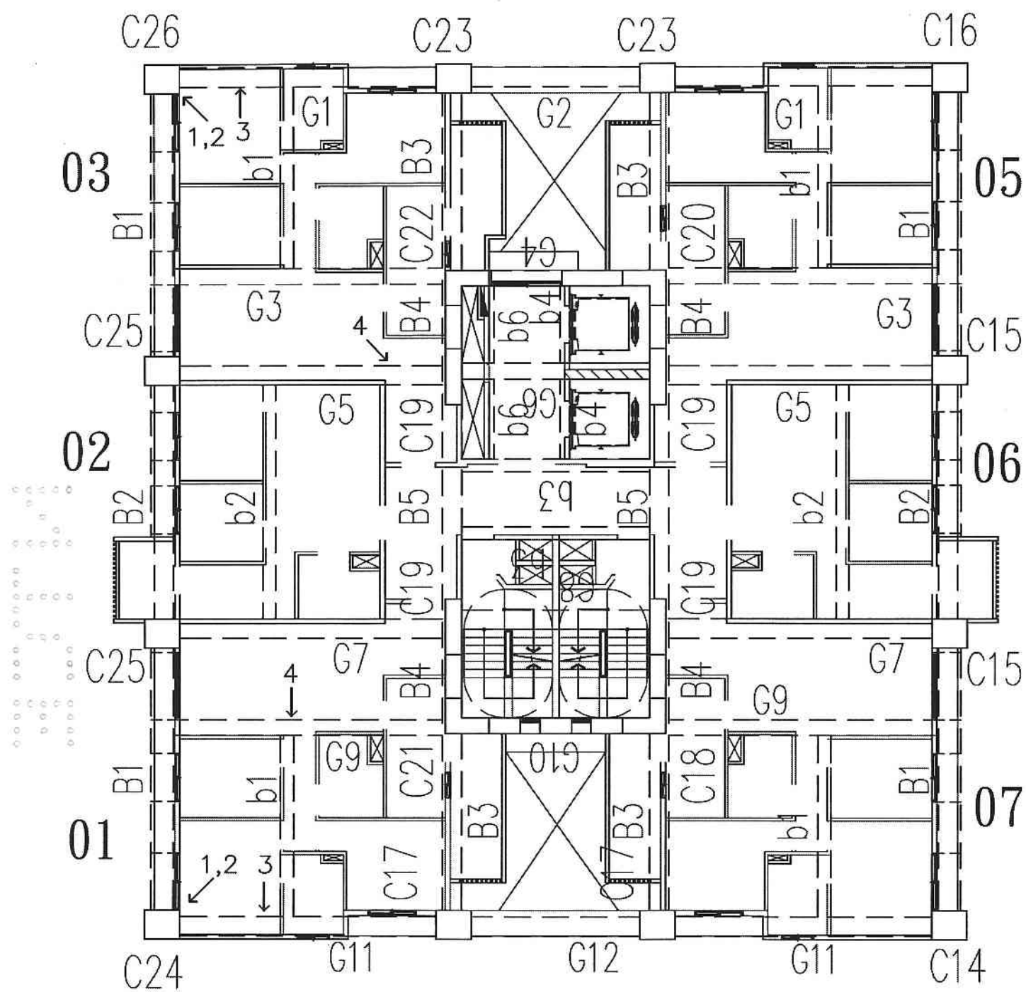
A6區T棟17層照片平面位置示意圖
