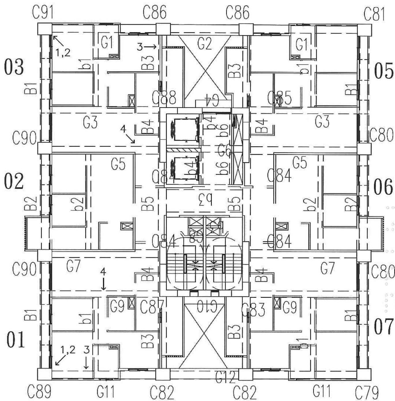
A6區S棟21層照片平面位置示意圖
