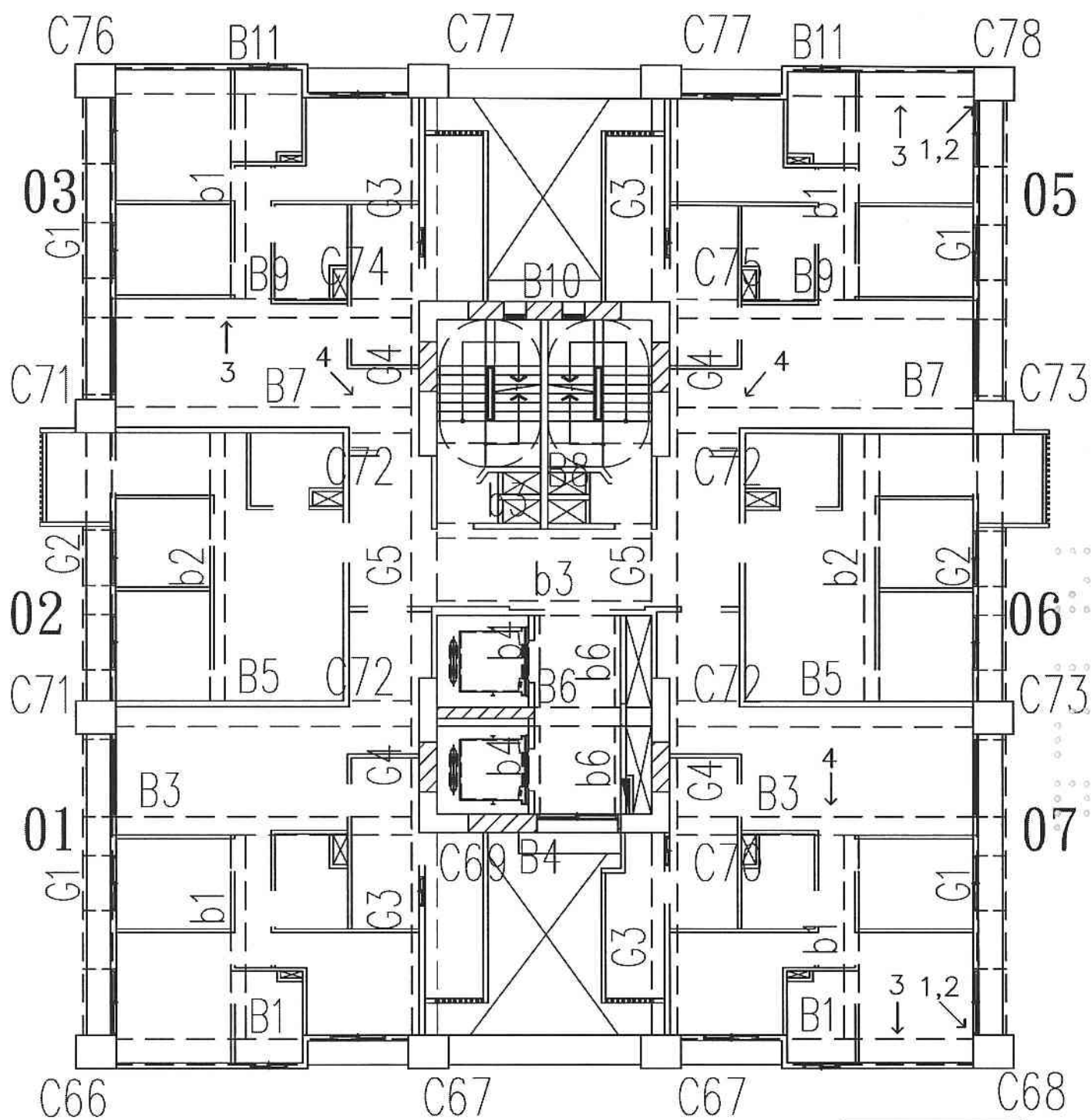
A6區U棟9層照片平面位置示意圖
