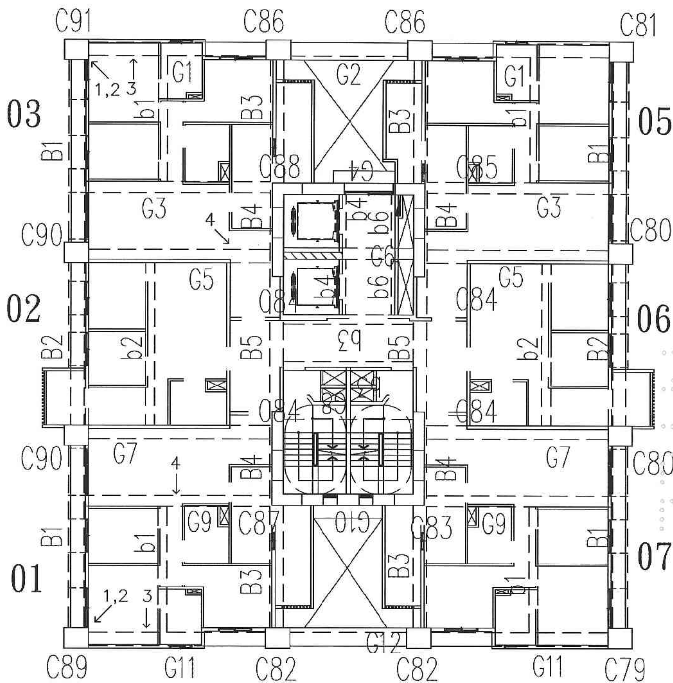
A6區S棟11層照片平面位置示意圖
