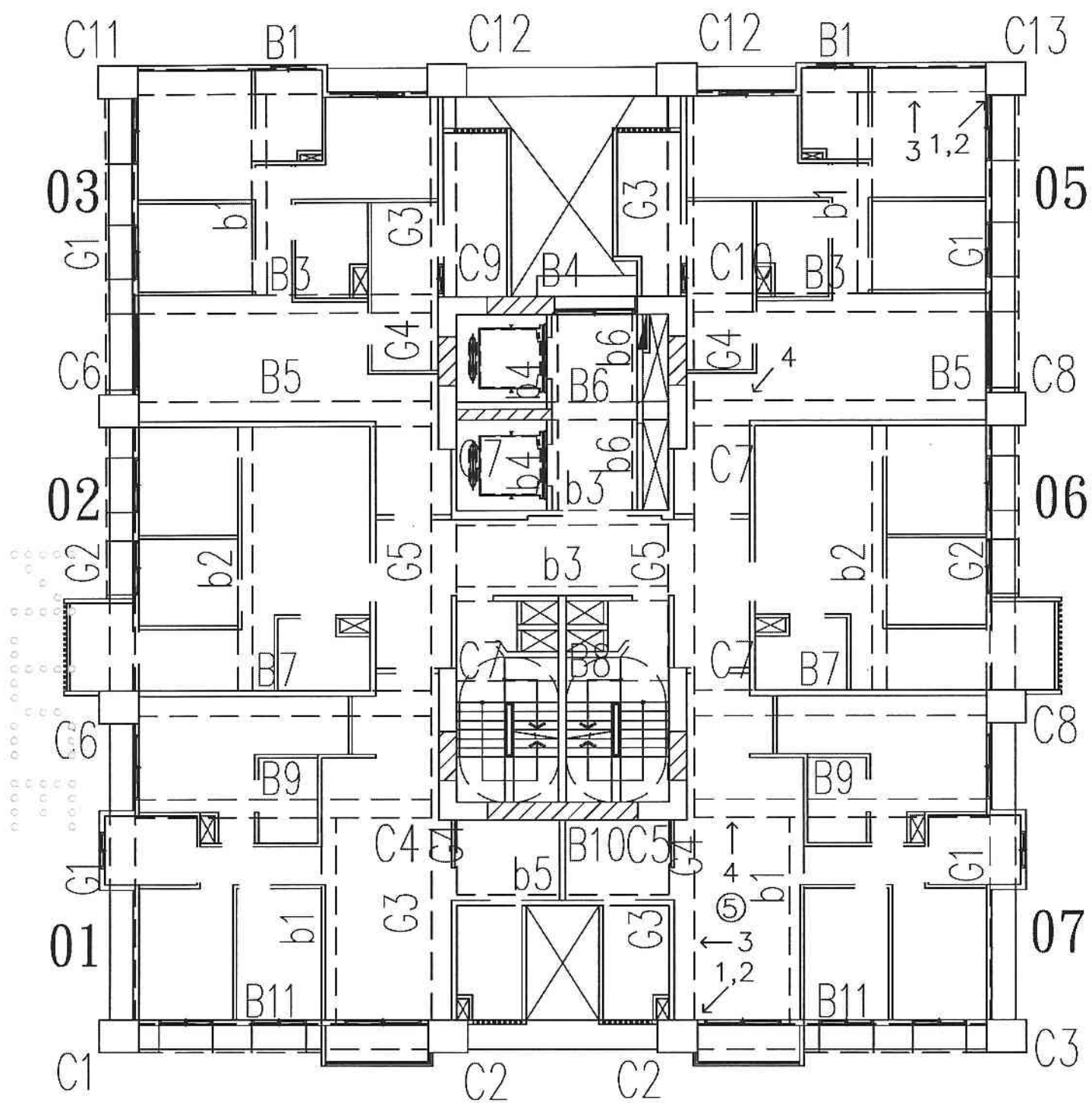
A6區V棟8層照片平面位置示意圖
