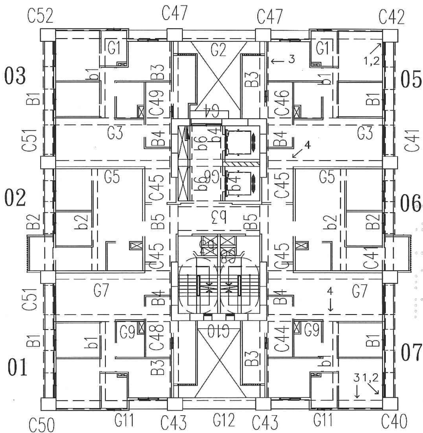
A6區R棟19層照片平面位置示意圖
