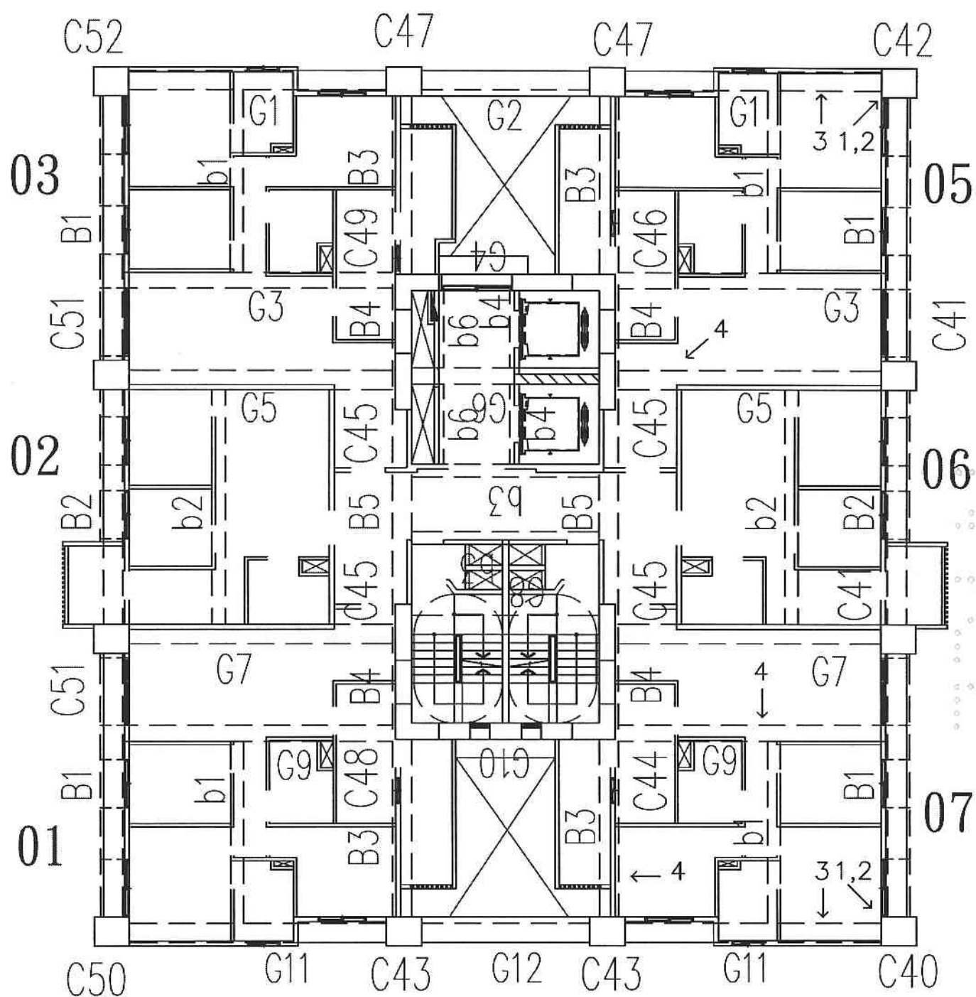
A6區R棟23層照片平面位置示意圖
