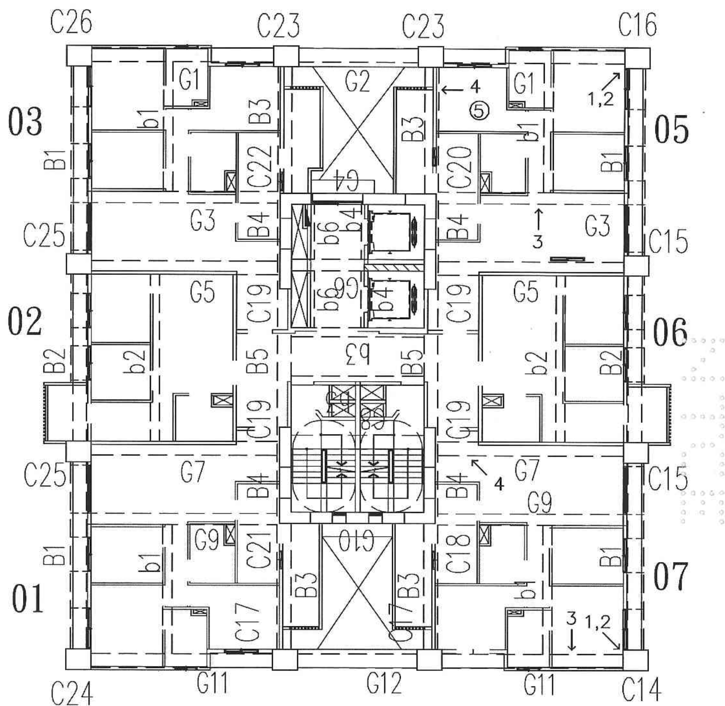
A6區T棟16層照片平面位置示意圖
