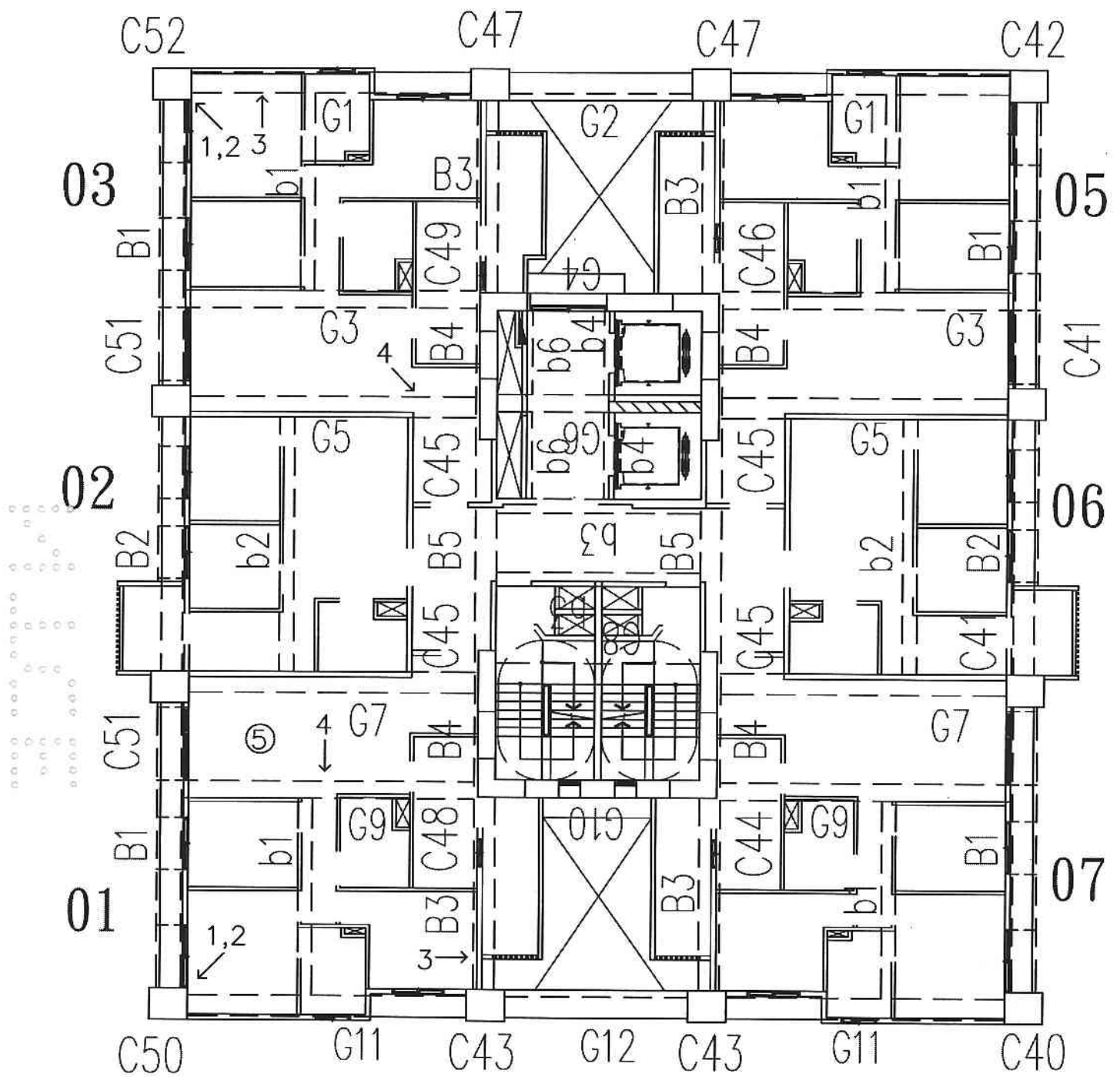
A6區R棟10層照片平面位置示意圖
