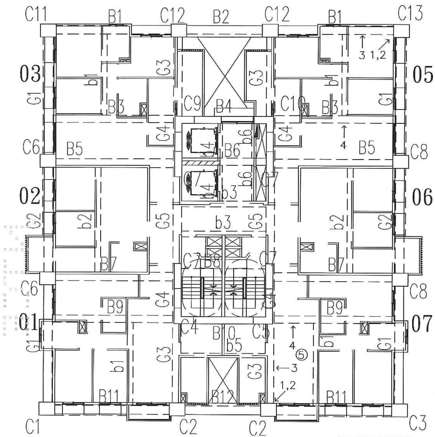
A6區J棟16層照片平面位置示意圖
