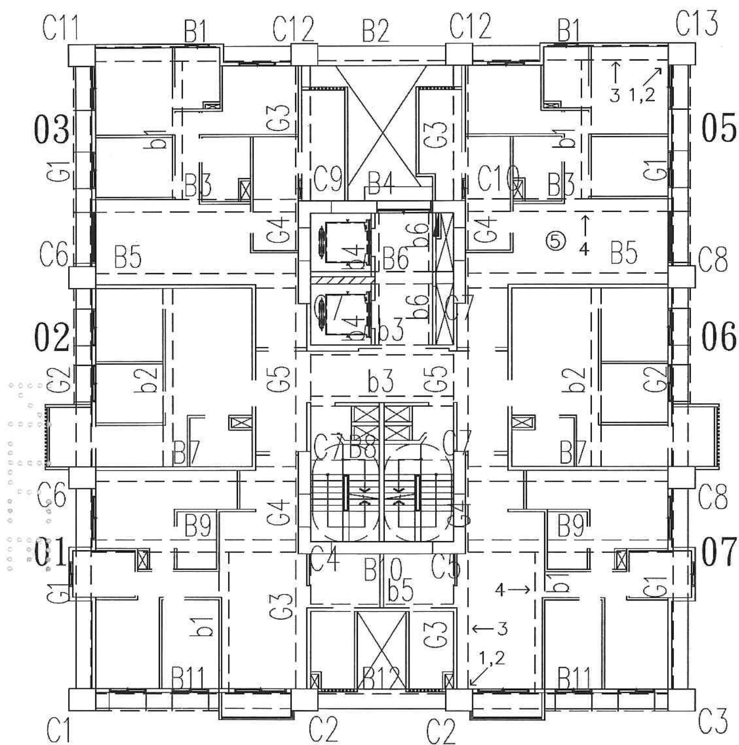
A6區J棟18層照片平面位置示意圖
