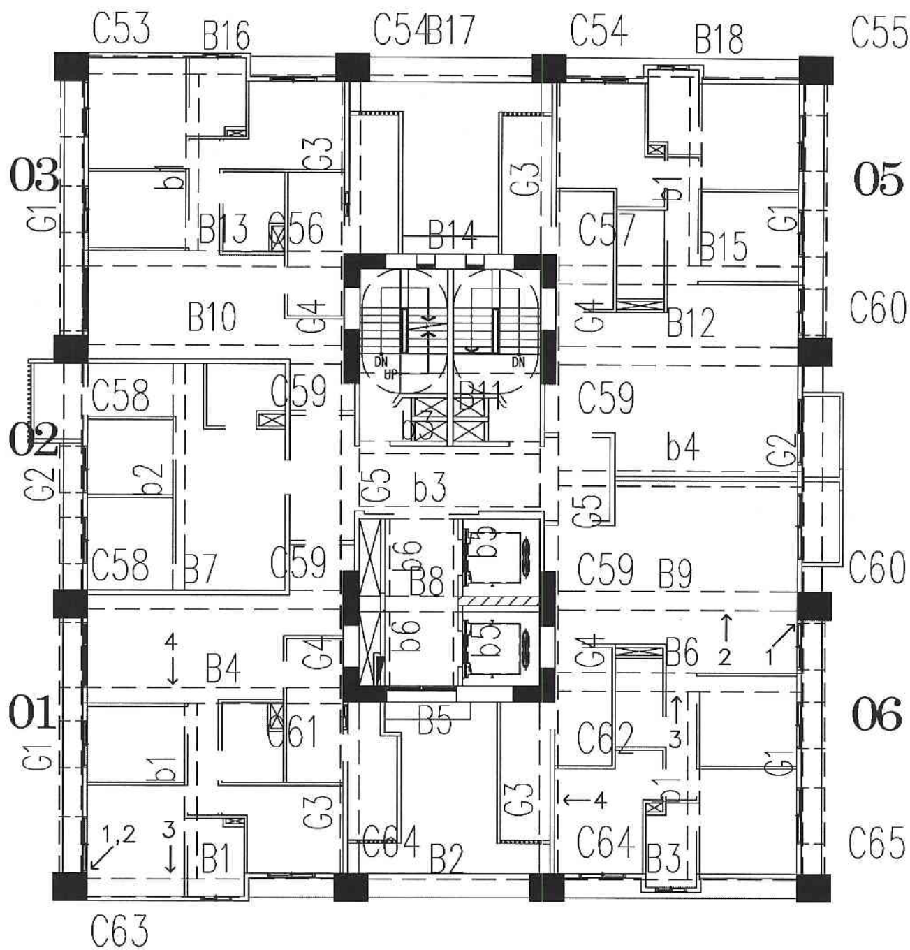
A6區L棟17層照片平面位置示意圖
