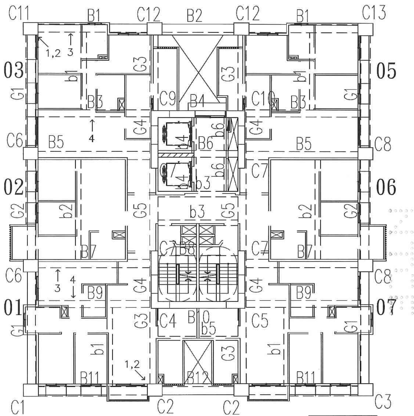
A6區J棟19層照片平面位置示意圖
