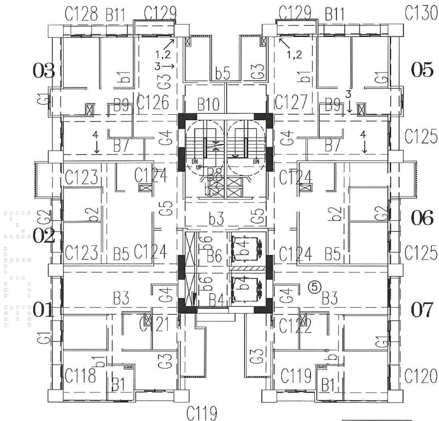
A6區K棟16層照片平面位置示意圖
