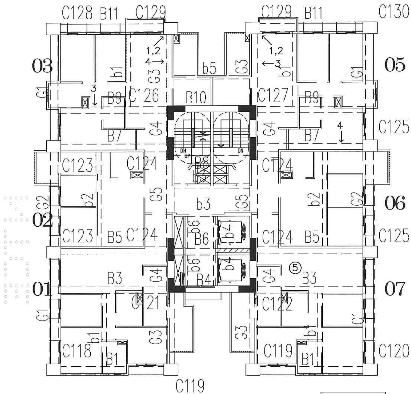
A6區K棟12層照片平面位置示意圖
