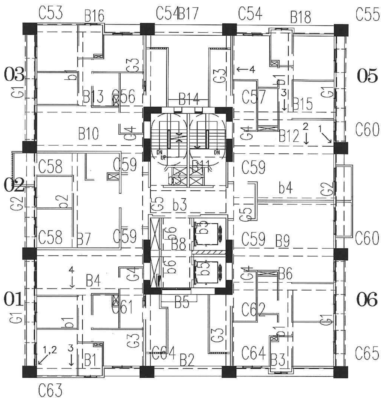
A6區L棟9層照片平面位置示意圖
