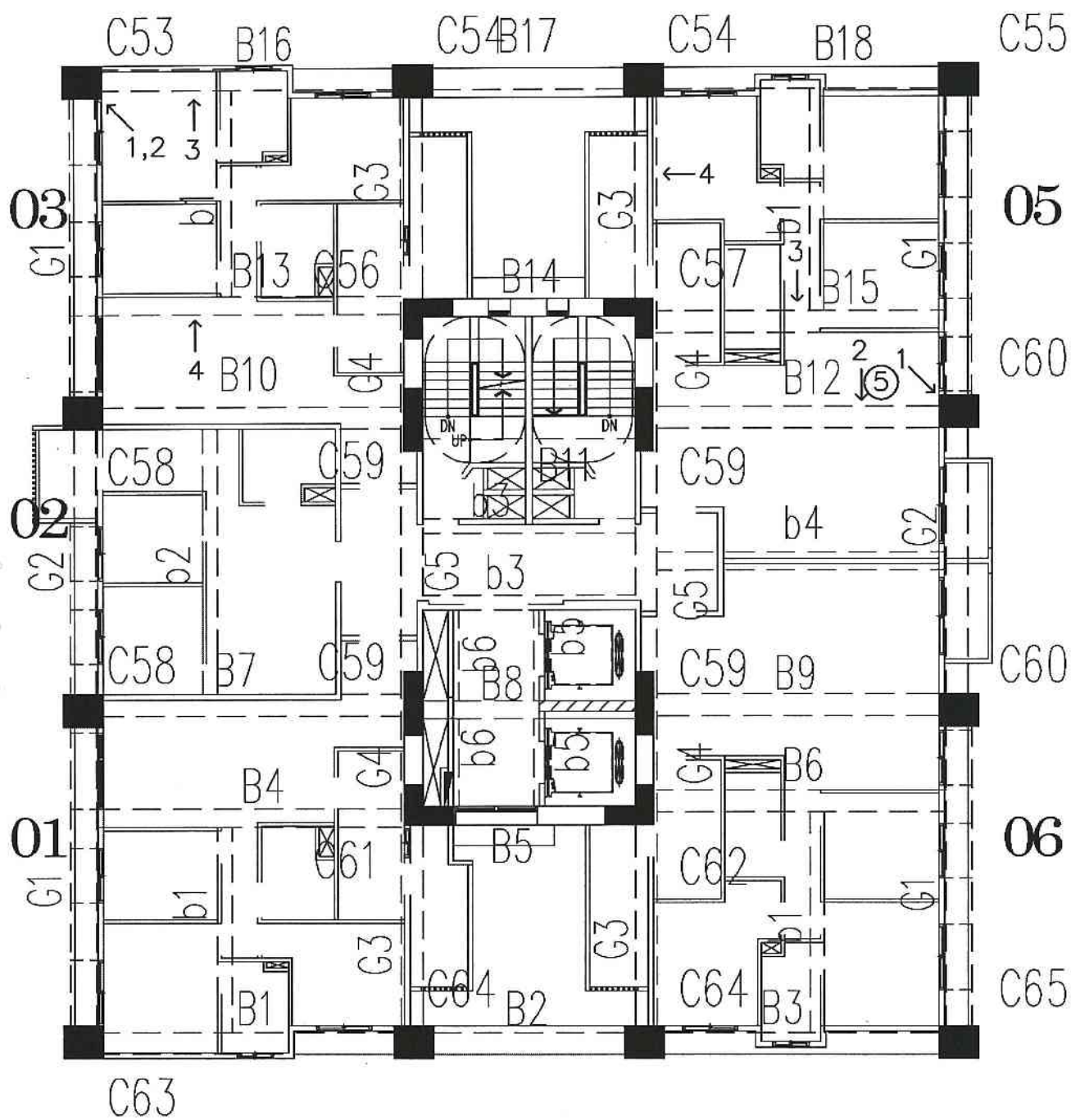
A6區L棟8層照片平面位置示意圖
