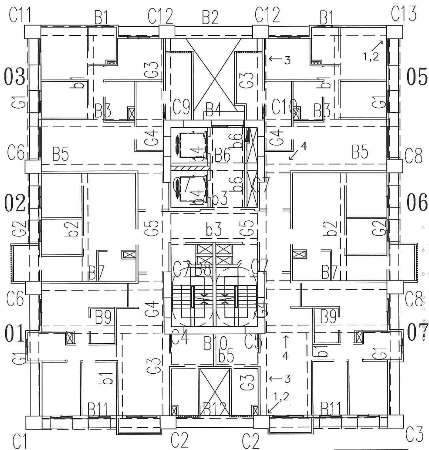
A6區J棟9層照片平面位置示意圖
