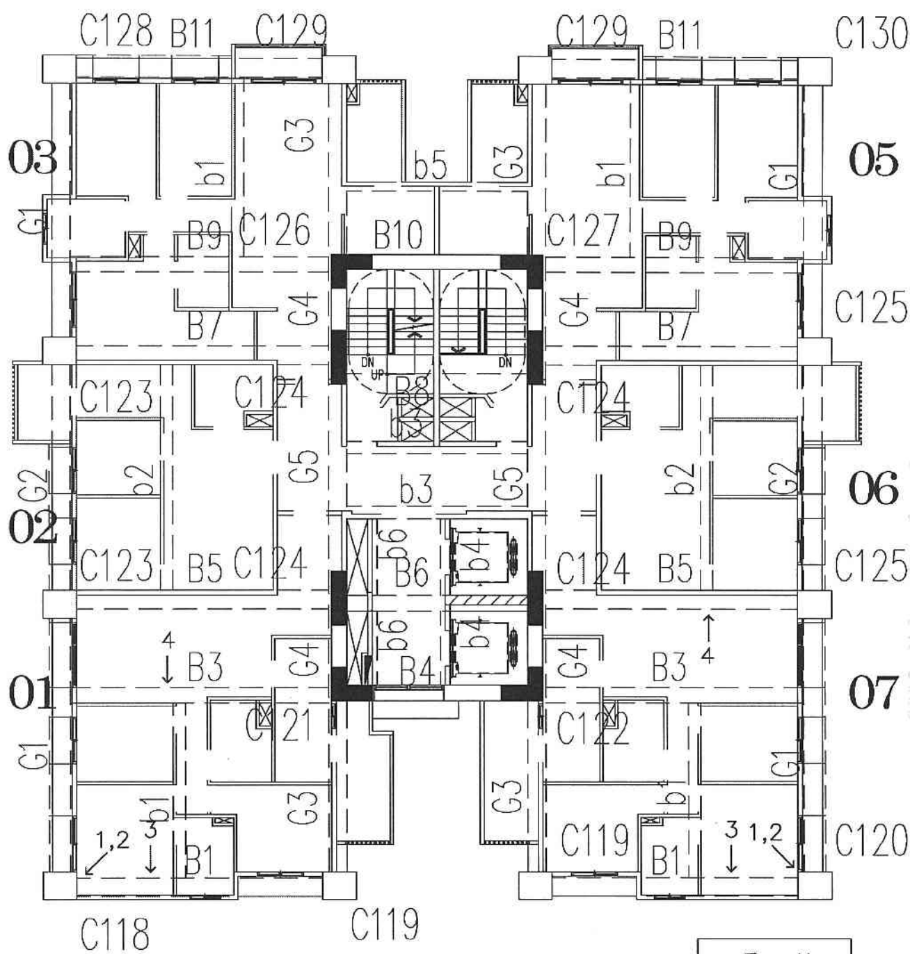
A6區K棟17層照片平面位置示意圖
