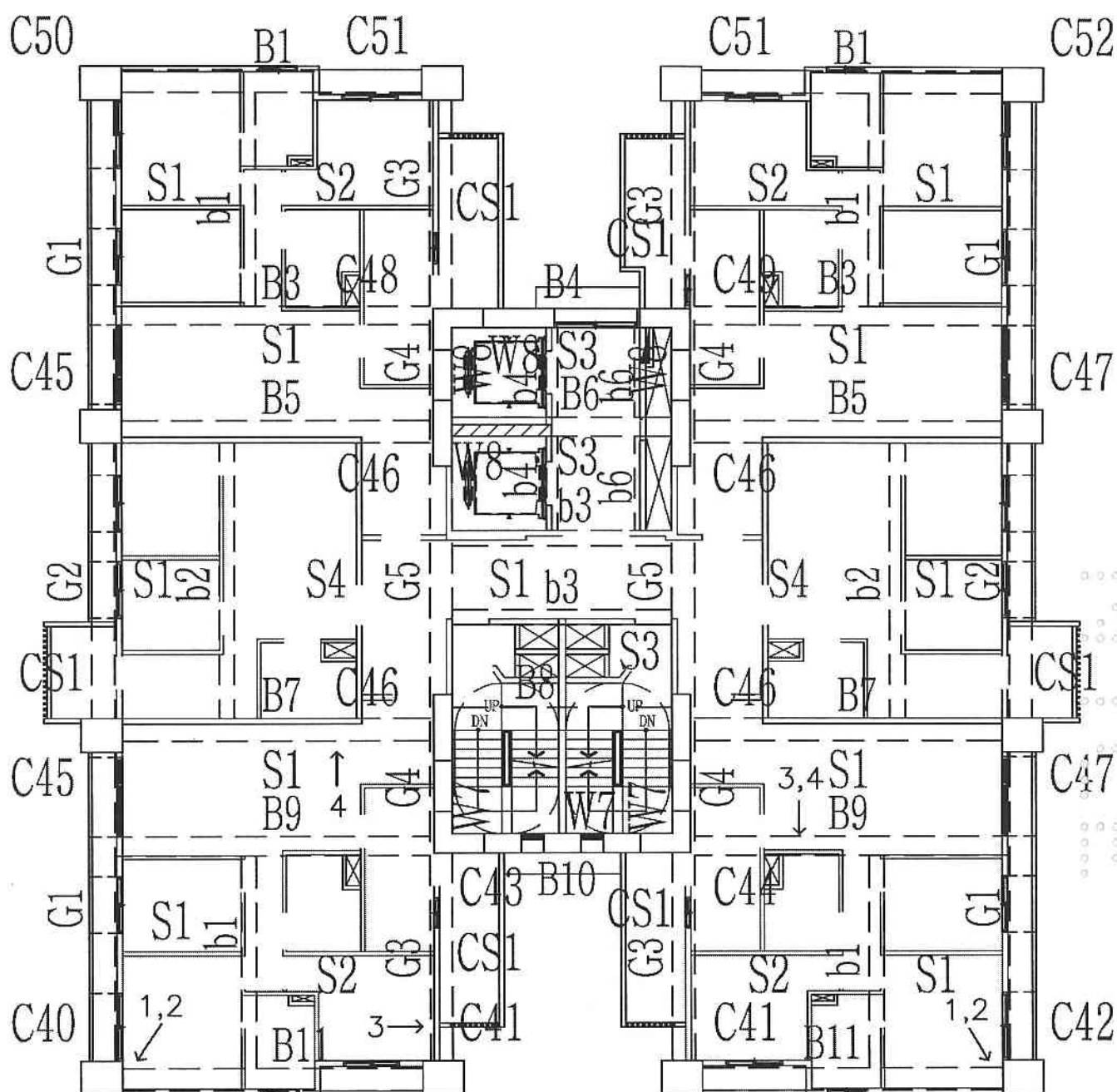
A6區I棟9層照片平面位置示意圖
