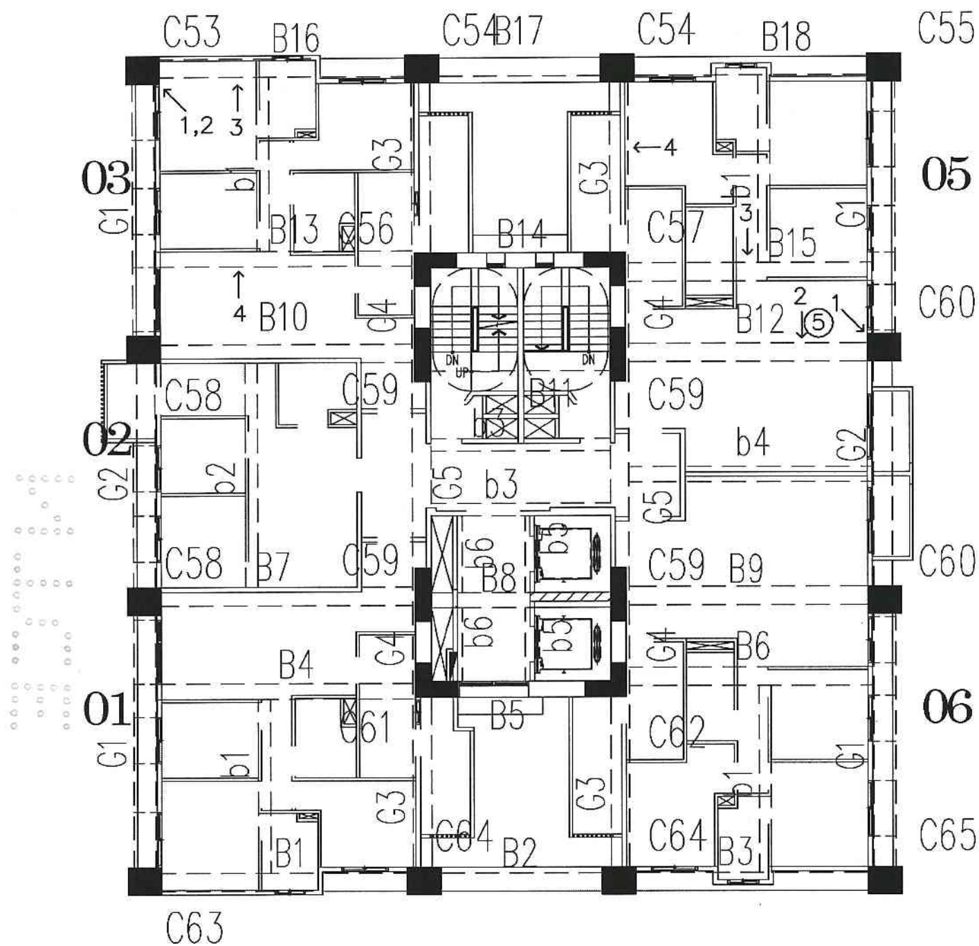
A6區L棟22層照片平面位置示意圖
