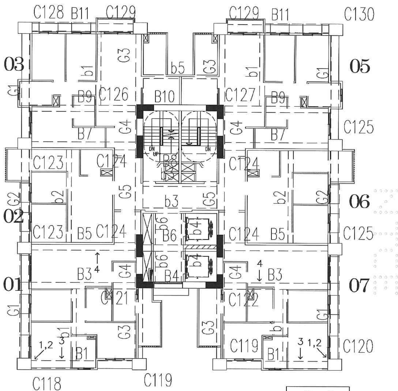
A6區K棟7層照片平面位置示意圖
