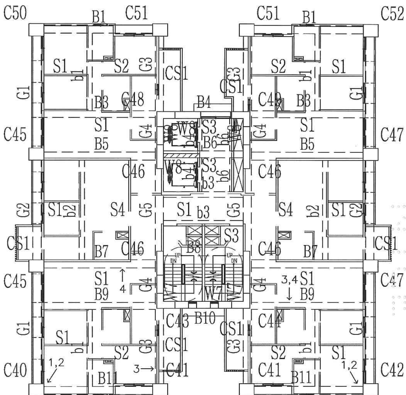
A6區I棟21層照片平面位置示意圖
