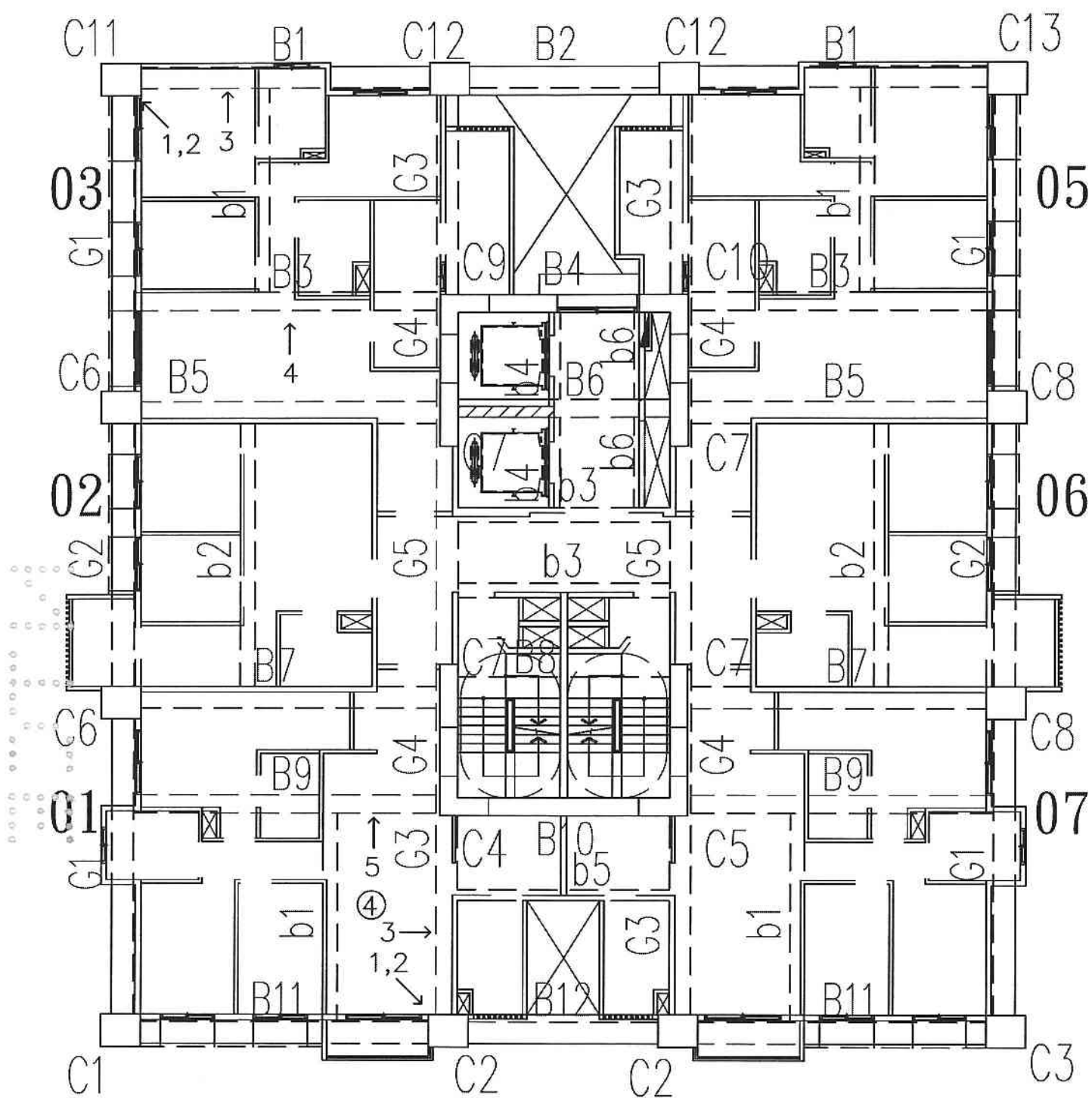
A6區J棟14層照片平面位置示意圖
