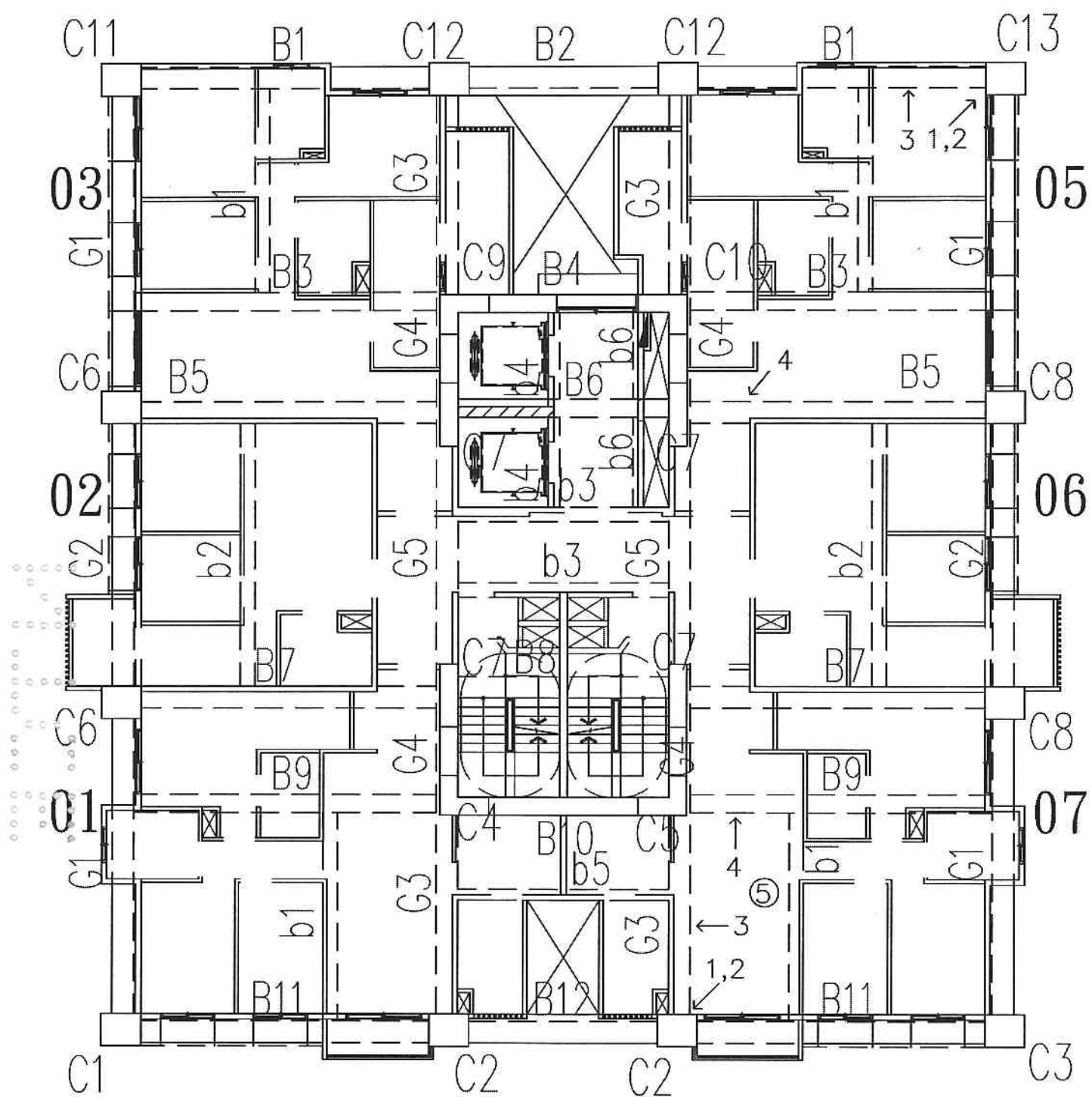
A6區J棟20層照片平面位置示意圖
