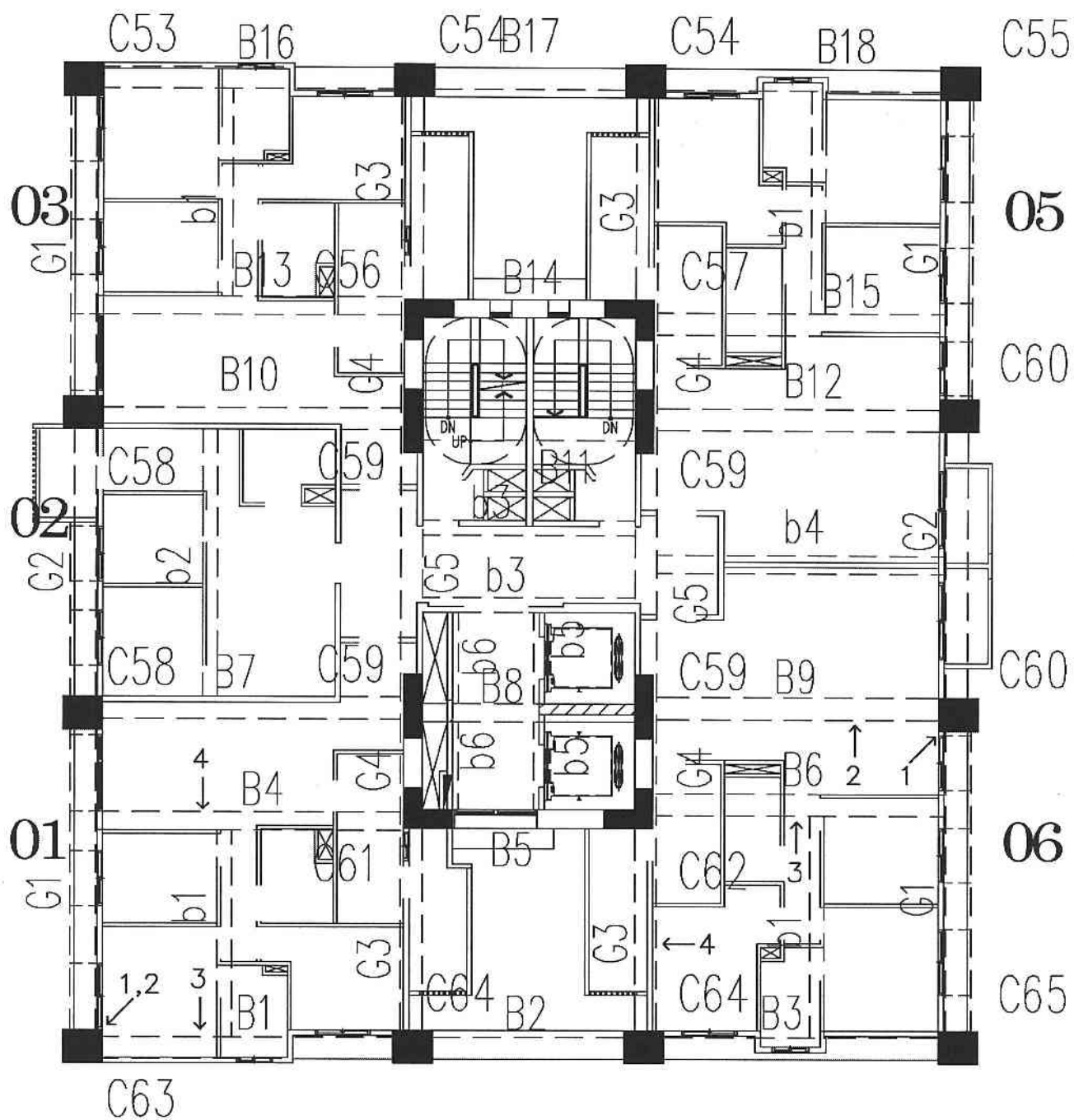
A6區L棟11層照片平面位置示意圖
