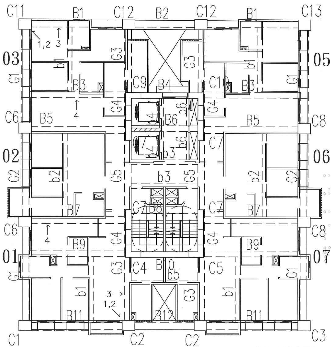
A6區J棟21層照片平面位置示意圖
