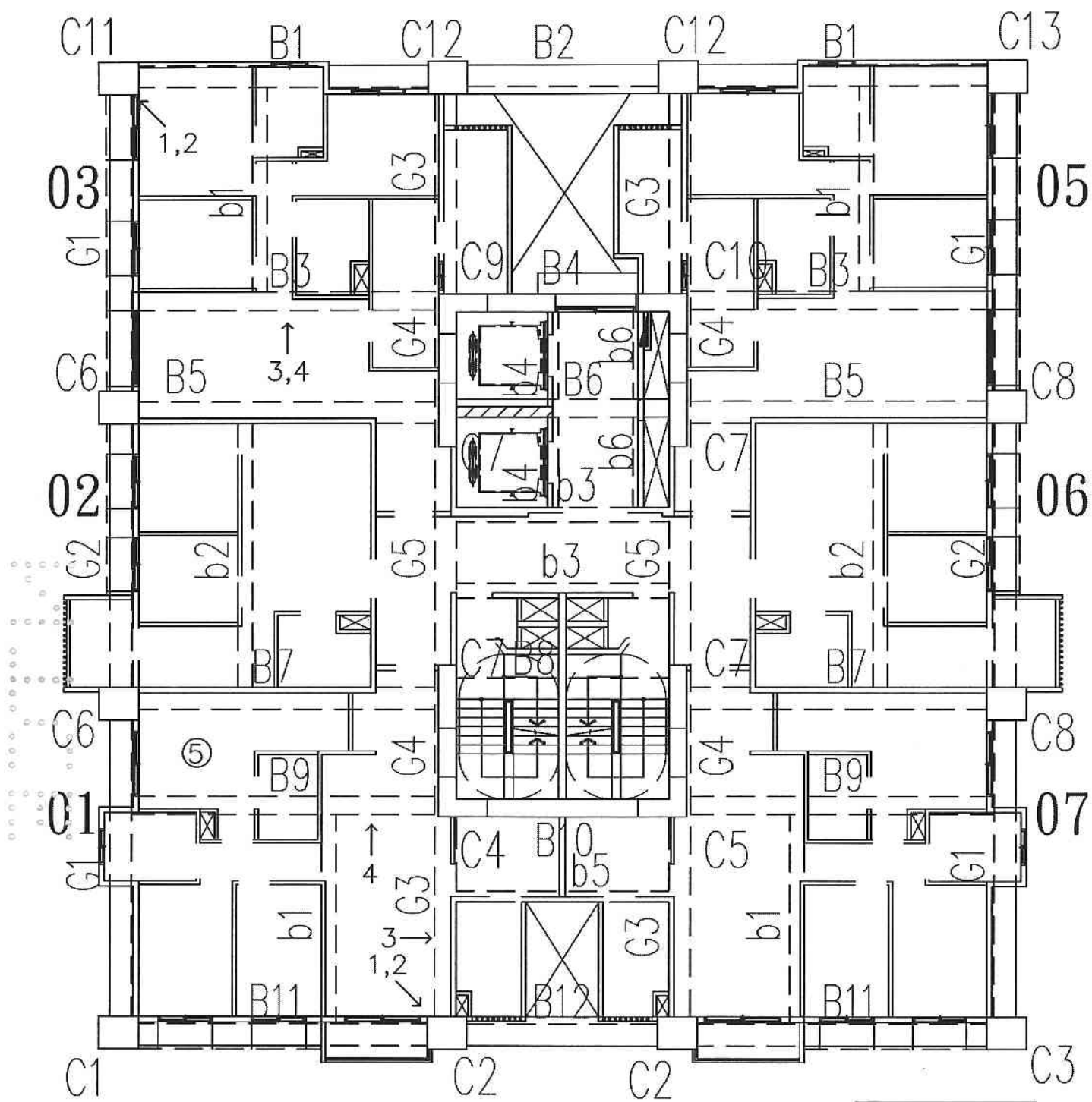
A6區J棟2層照片平面位置示意圖
