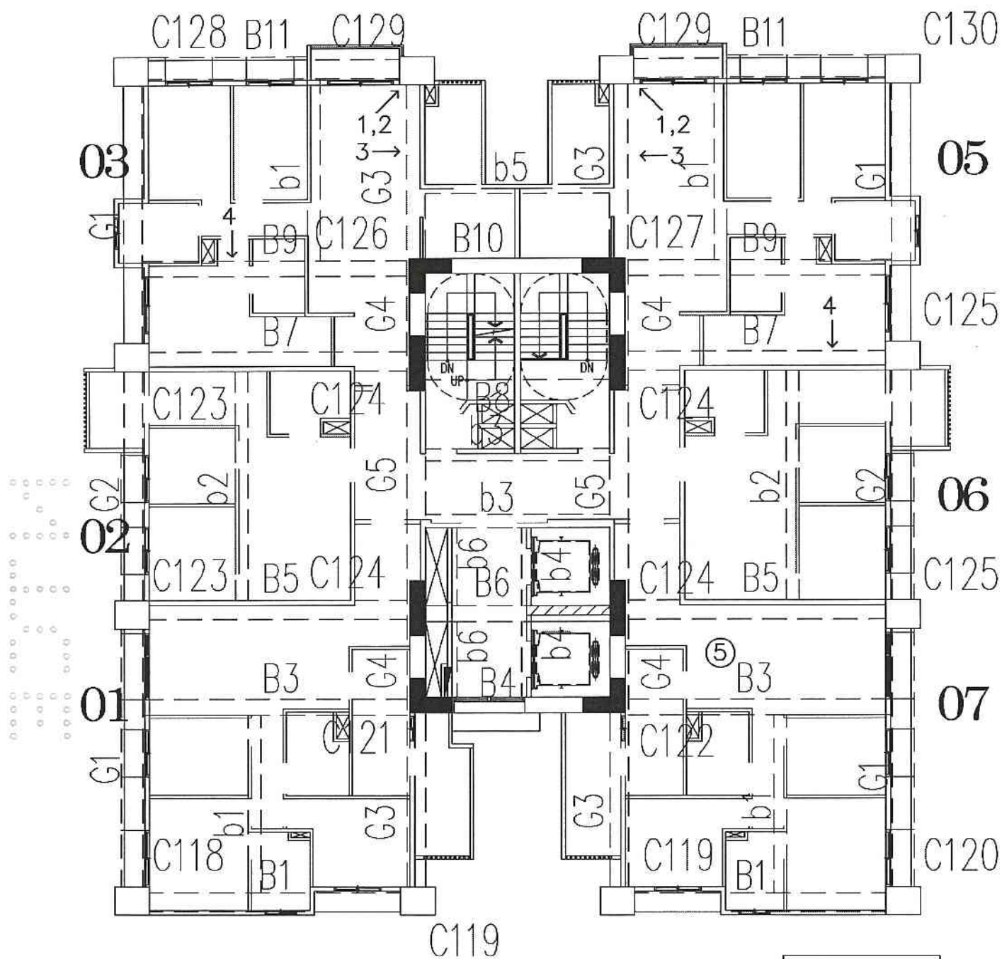
A6區K棟8層照片平面位置示意圖
