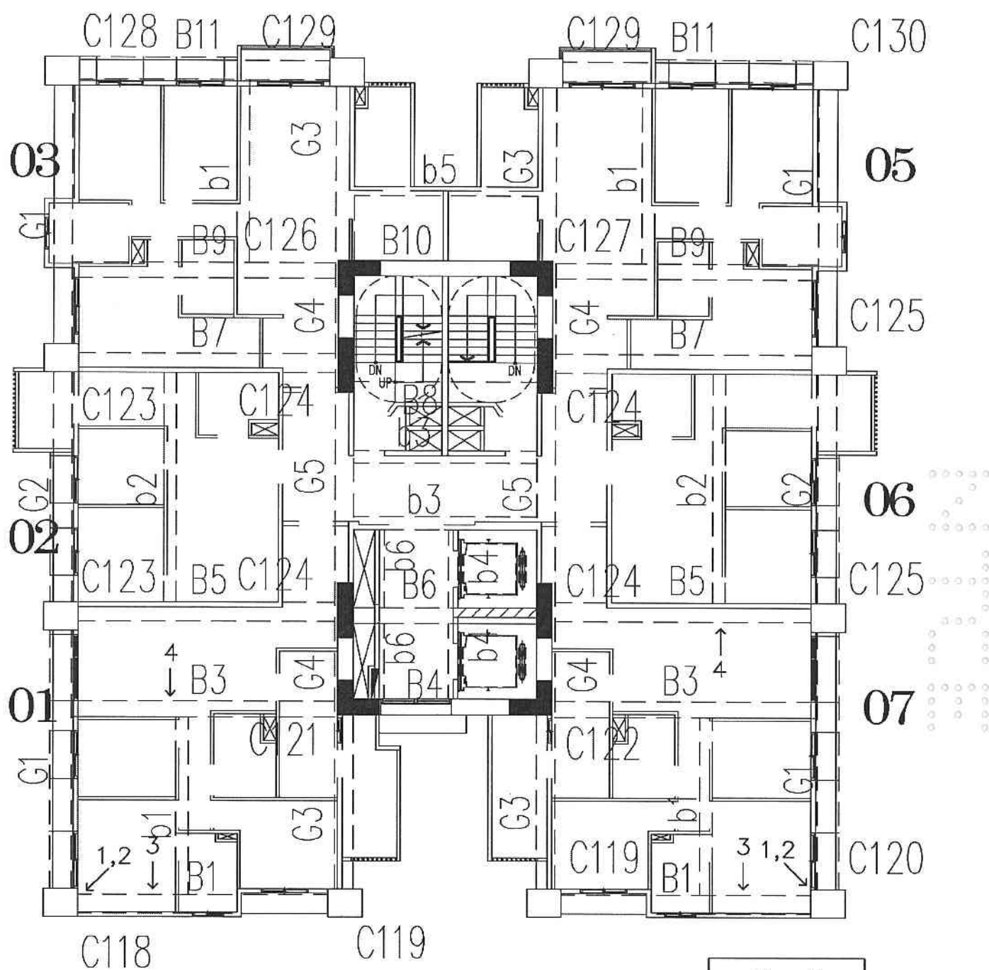
A6區K棟11層照片平面位置示意圖
