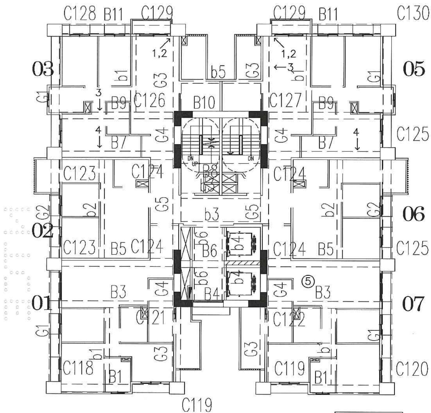
A6區K棟14層照片平面位置示意圖
