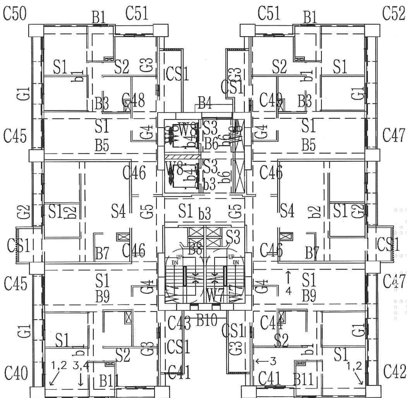
A6區I棟11層照片平面位置示意圖
