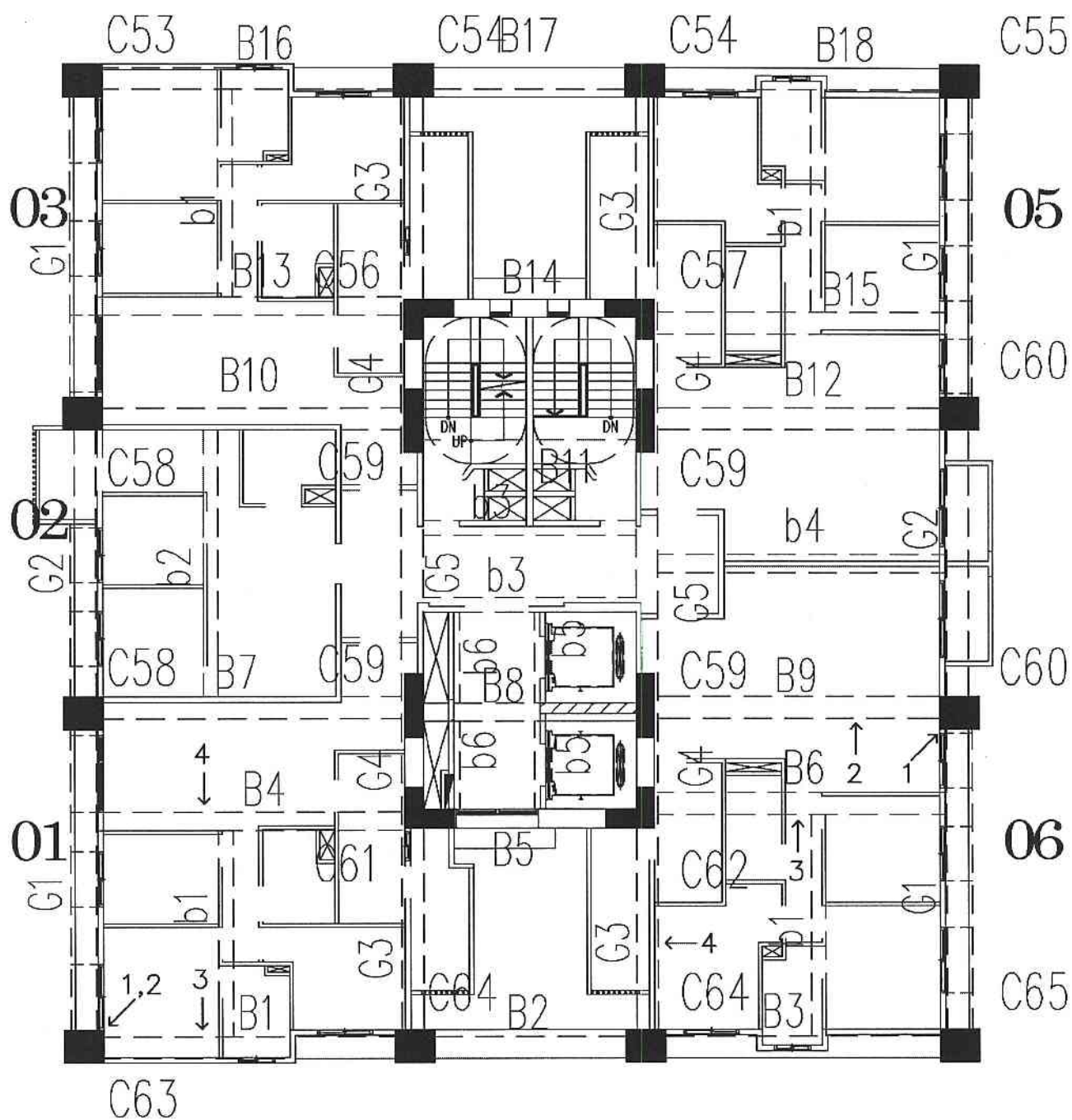
A6區L棟19層照片平面位置示意圖
