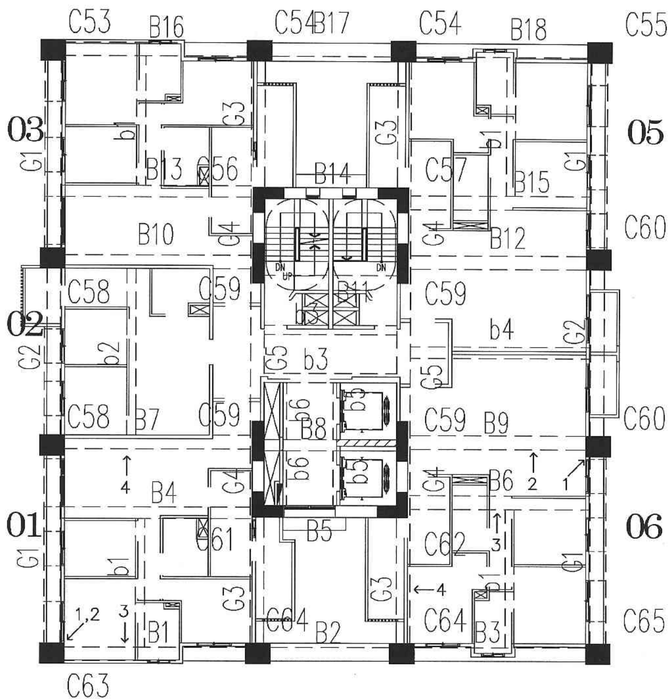
A6區L棟21層照片平面位置示意圖
