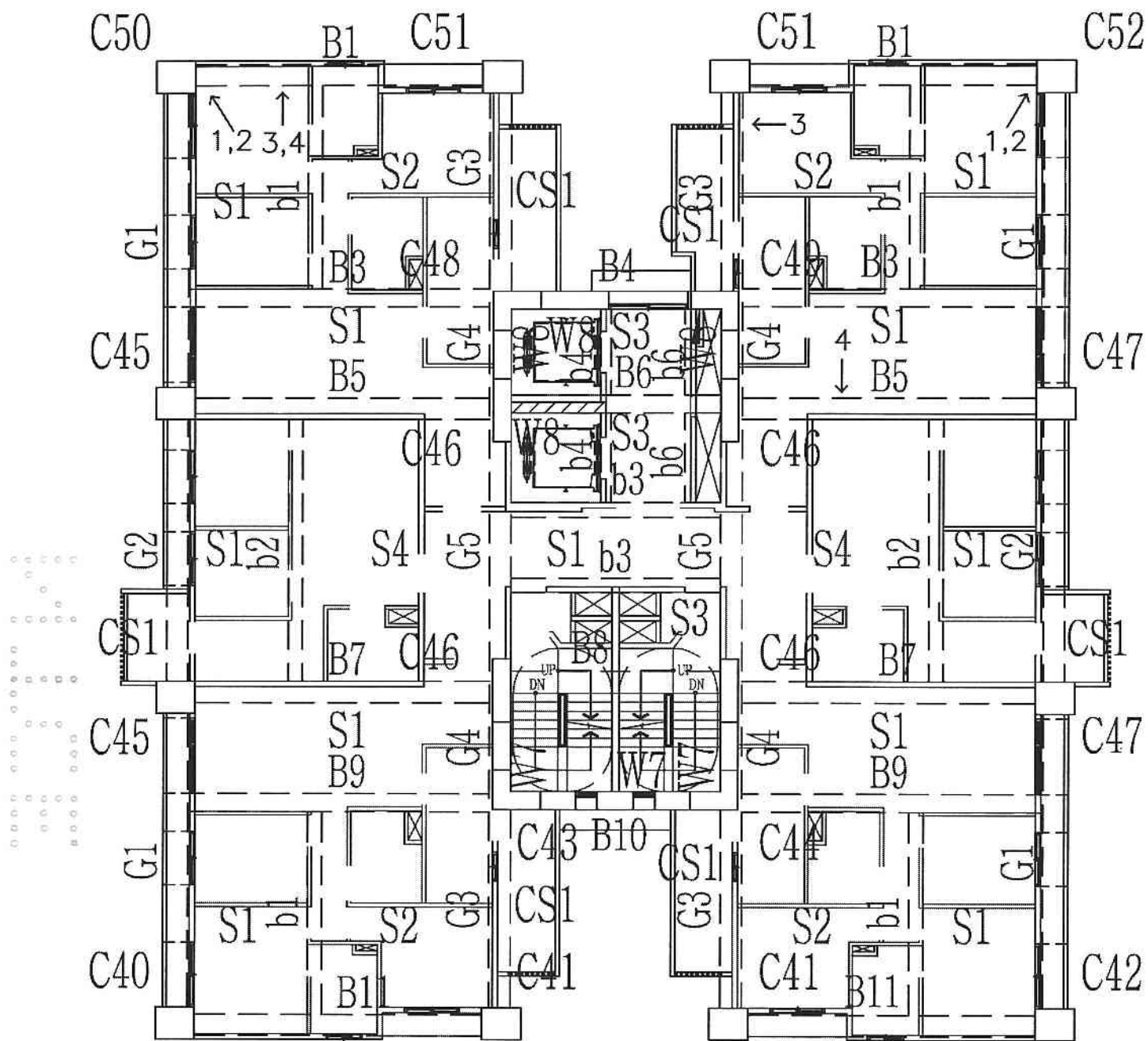
A6區I棟2層照片平面位置示意圖
