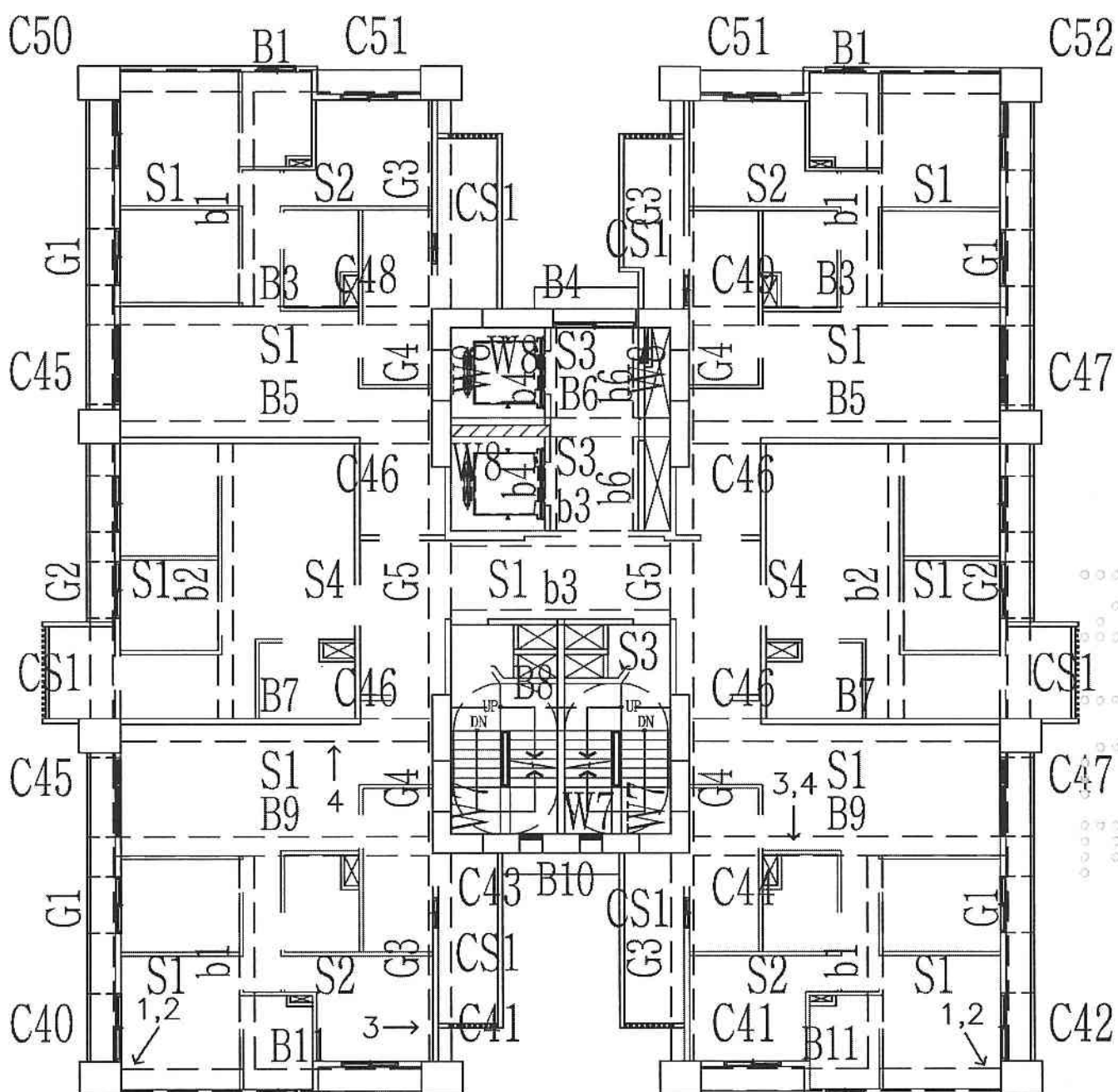
A6區I棟15層照片平面位置示意圖
