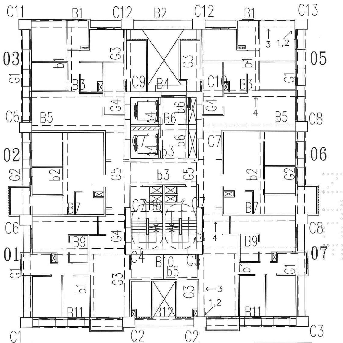
A6區J棟7層照片平面位置示意圖
