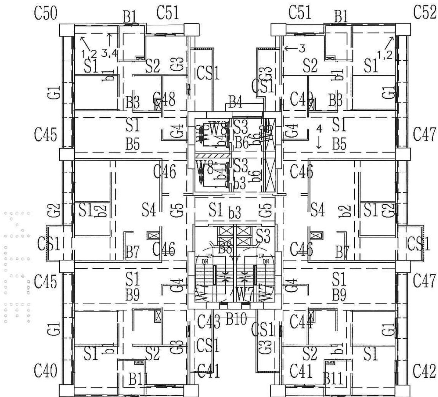
A6區I棟8層照片平面位置示意圖
