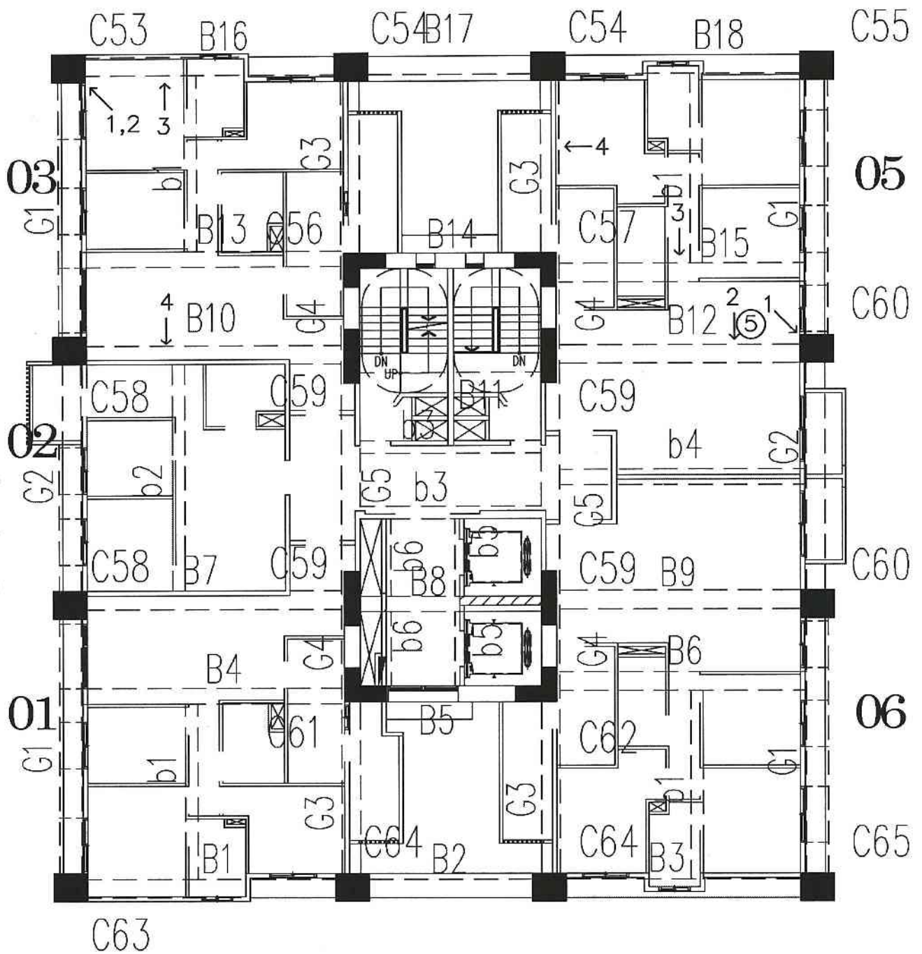
A6區L棟10層照片平面位置示意圖
