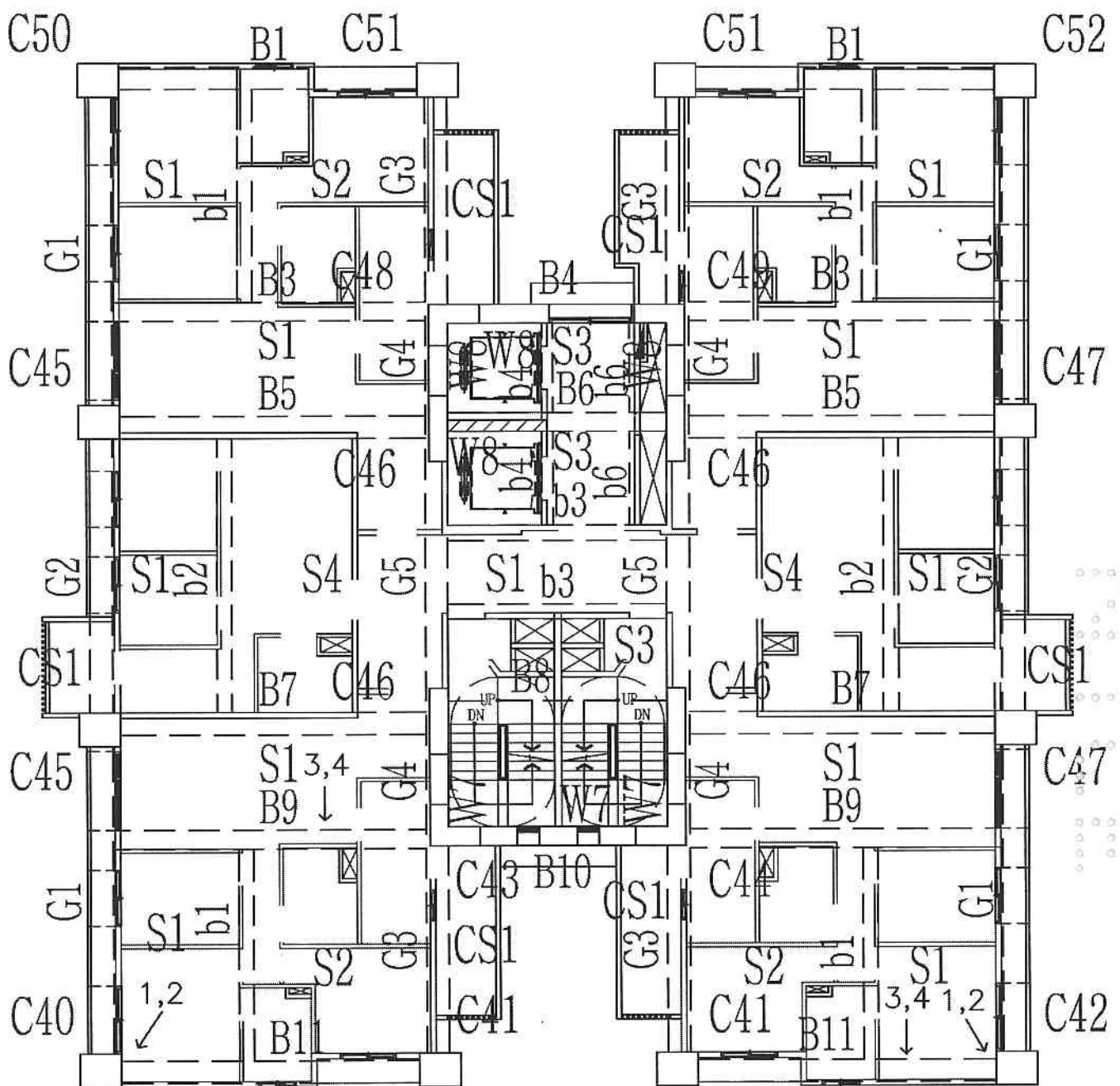
A6區I棟7層照片平面位置示意圖
