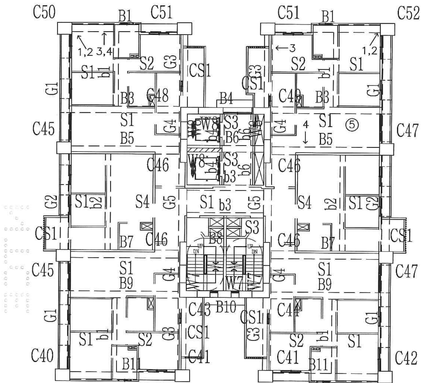
A6區I棟14層照片平面位置示意圖
