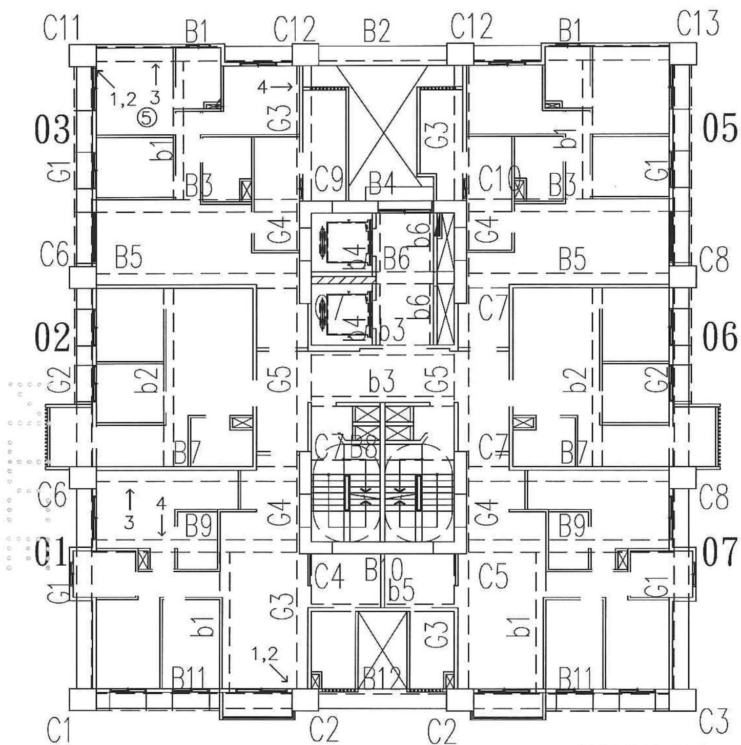
A6區J棟4層照片平面位置示意圖
