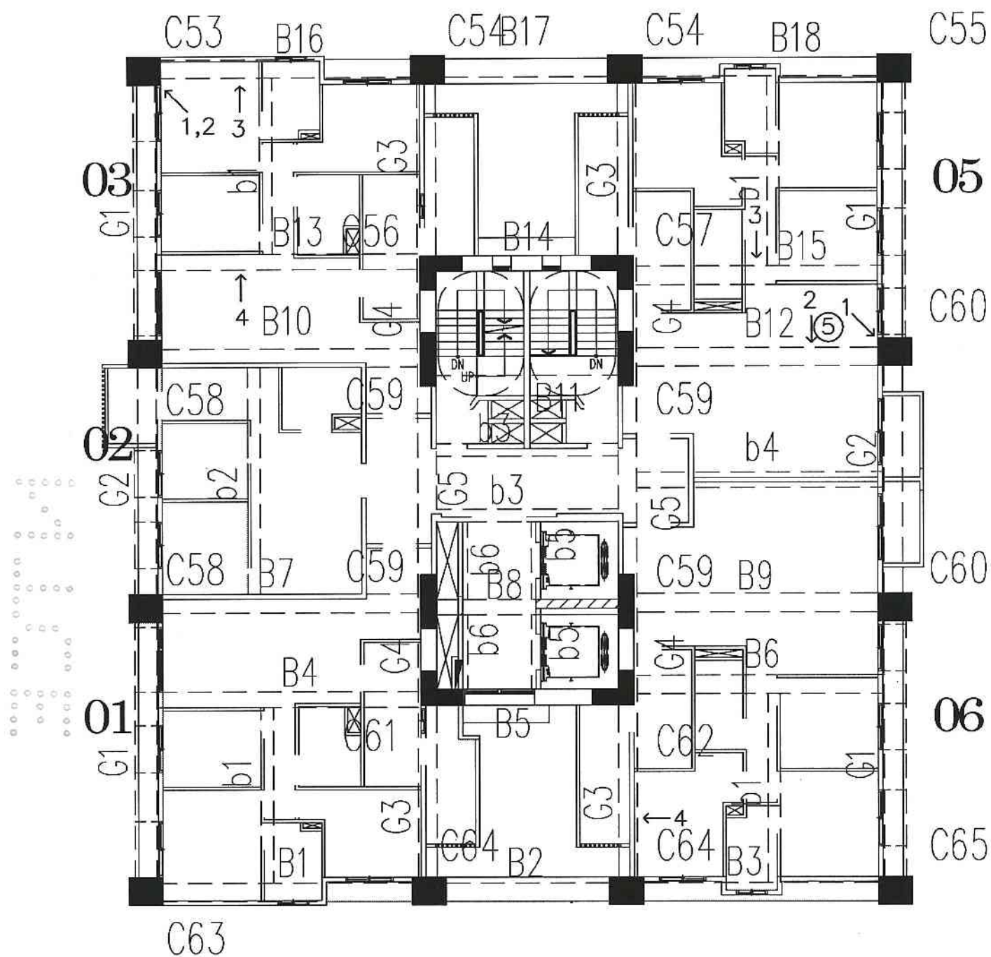
A6區L棟20層照片平面位置示意圖
