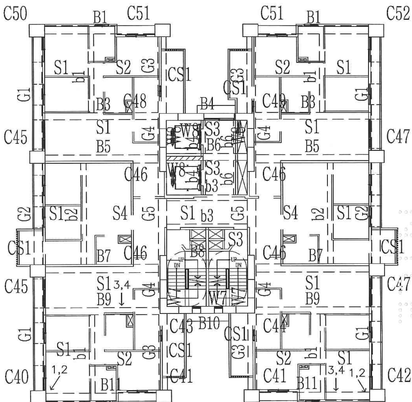
A6區I棟13層照片平面位置示意圖
