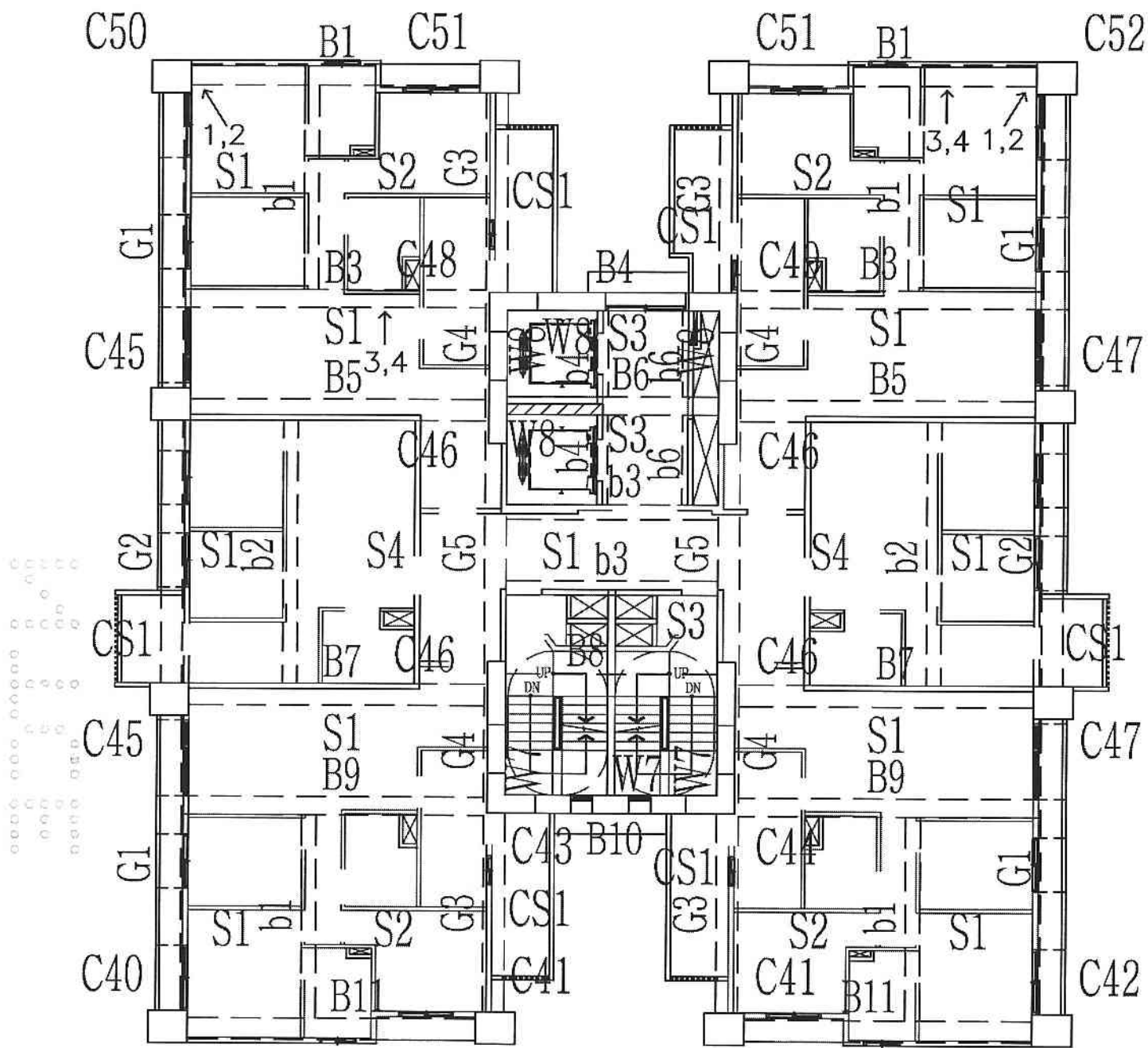
A6區I棟16層照片平面位置示意圖
