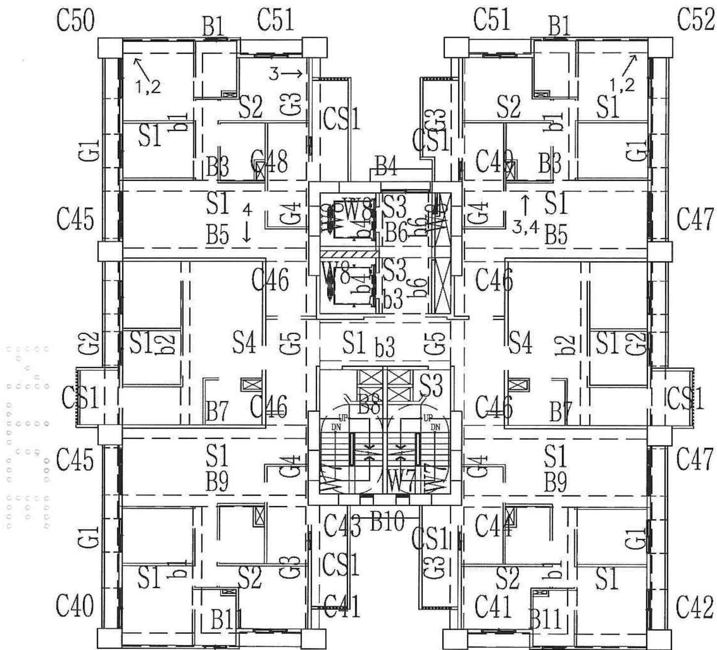
A6區I棟12層照片平面位置示意圖
