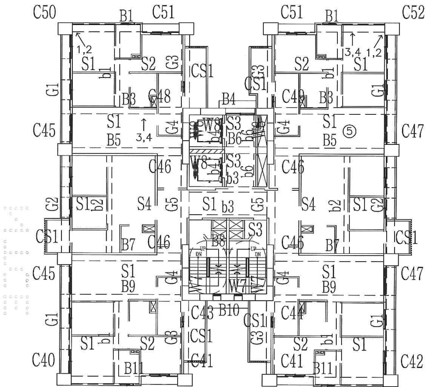
A6區I棟10層照片平面位置示意圖
