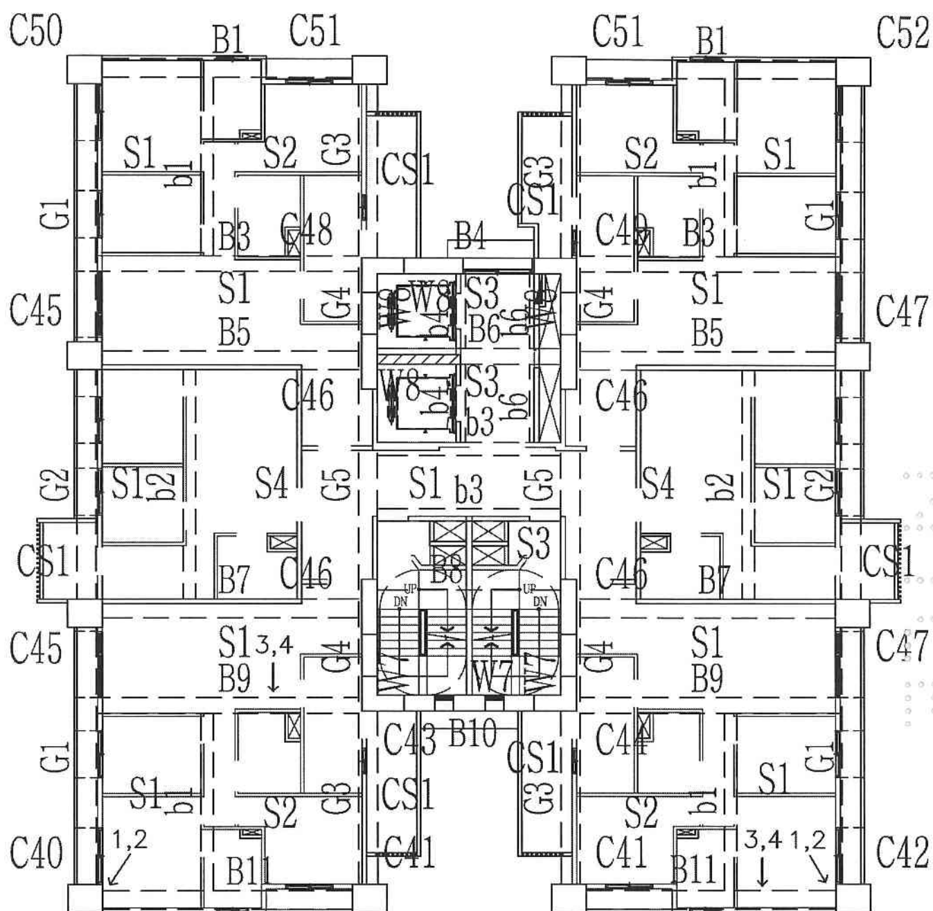
A6區I棟19層照片平面位置示意圖
