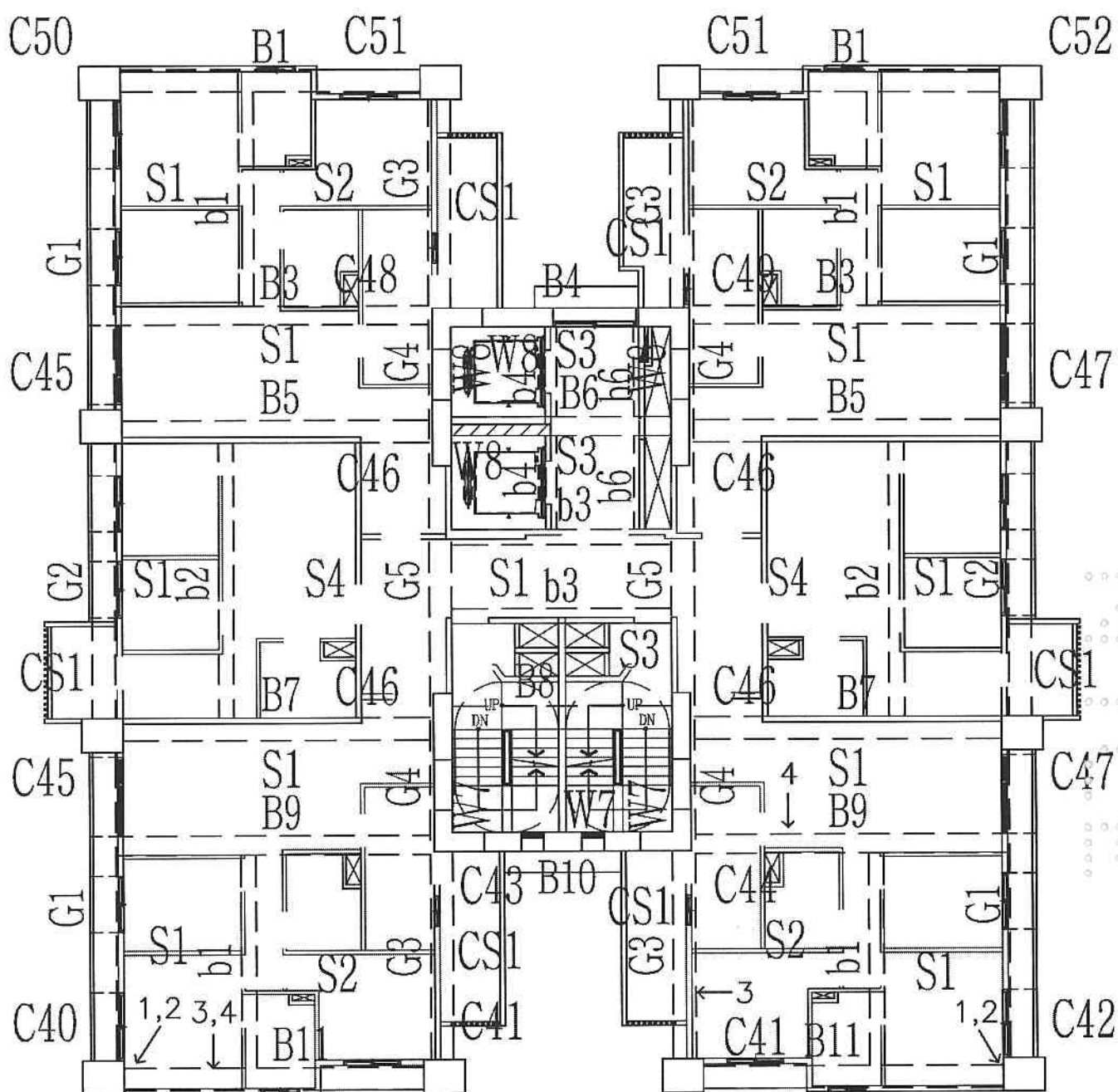
A6區I棟5層照片平面位置示意圖
