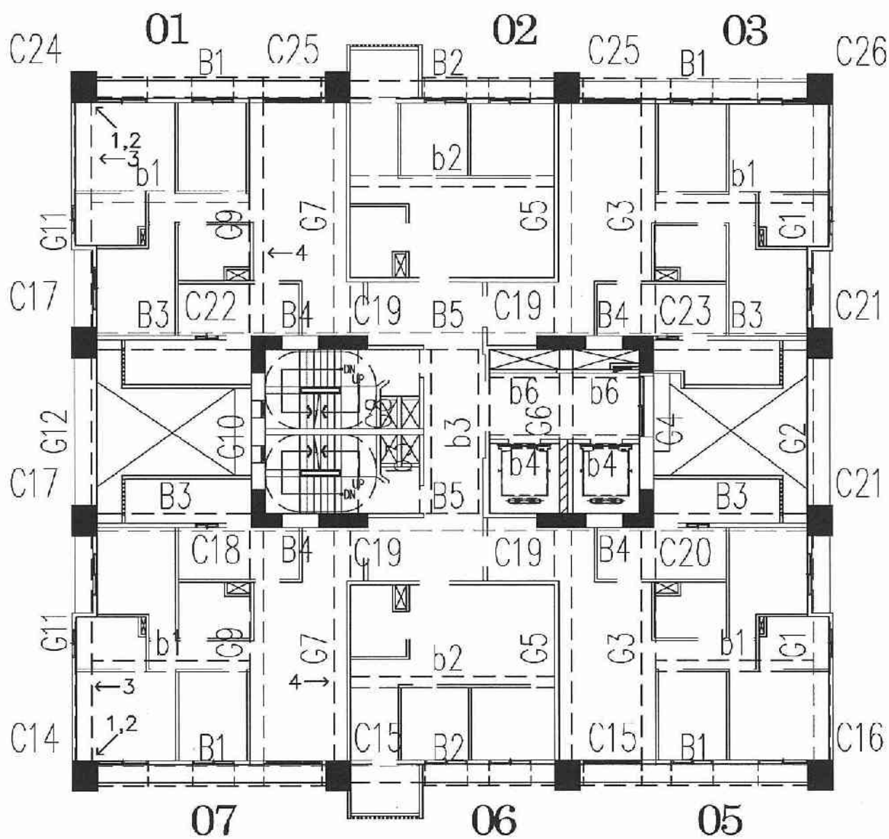
A6區F棟17層照片平面位置示意圖
