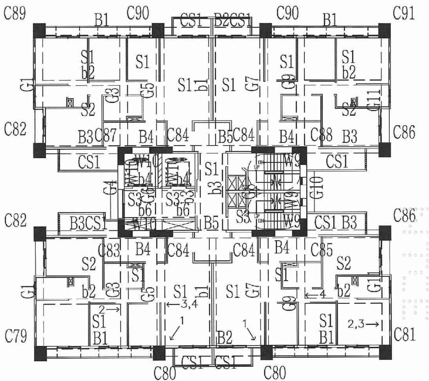
A6區E棟7層照片平面位置示意圖
