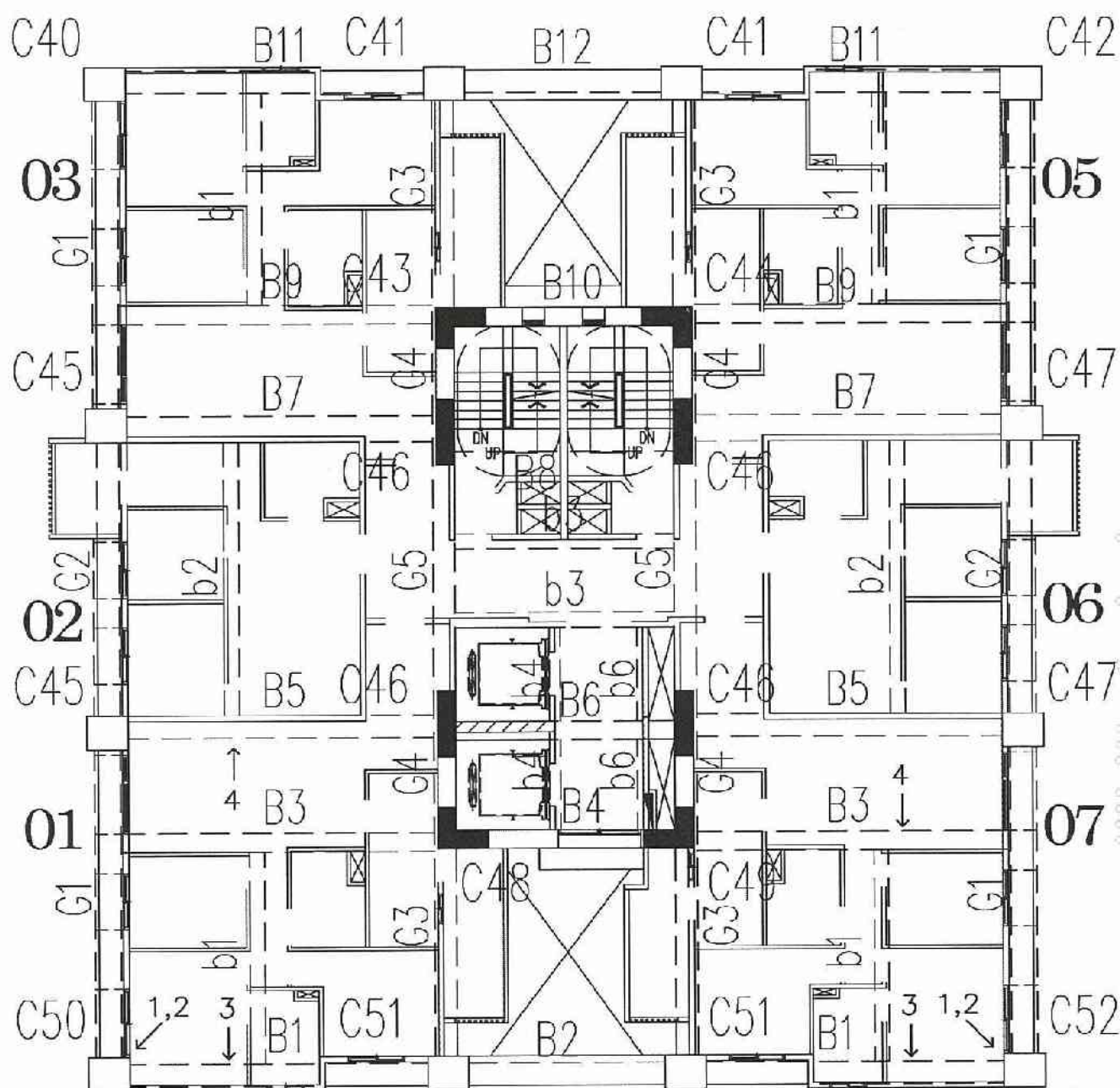
A6區H棟9層照片平面位置示意圖
