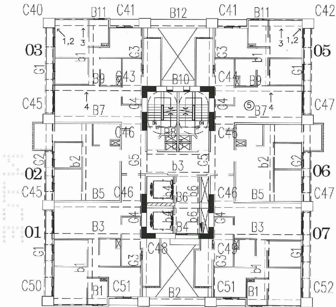
A6區H棟12層照片平面位置示意圖
