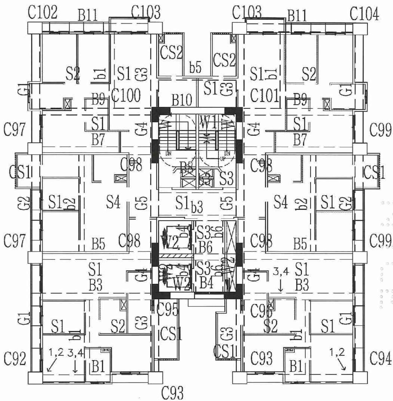
A6區G棟5層照片平面位置示意圖
