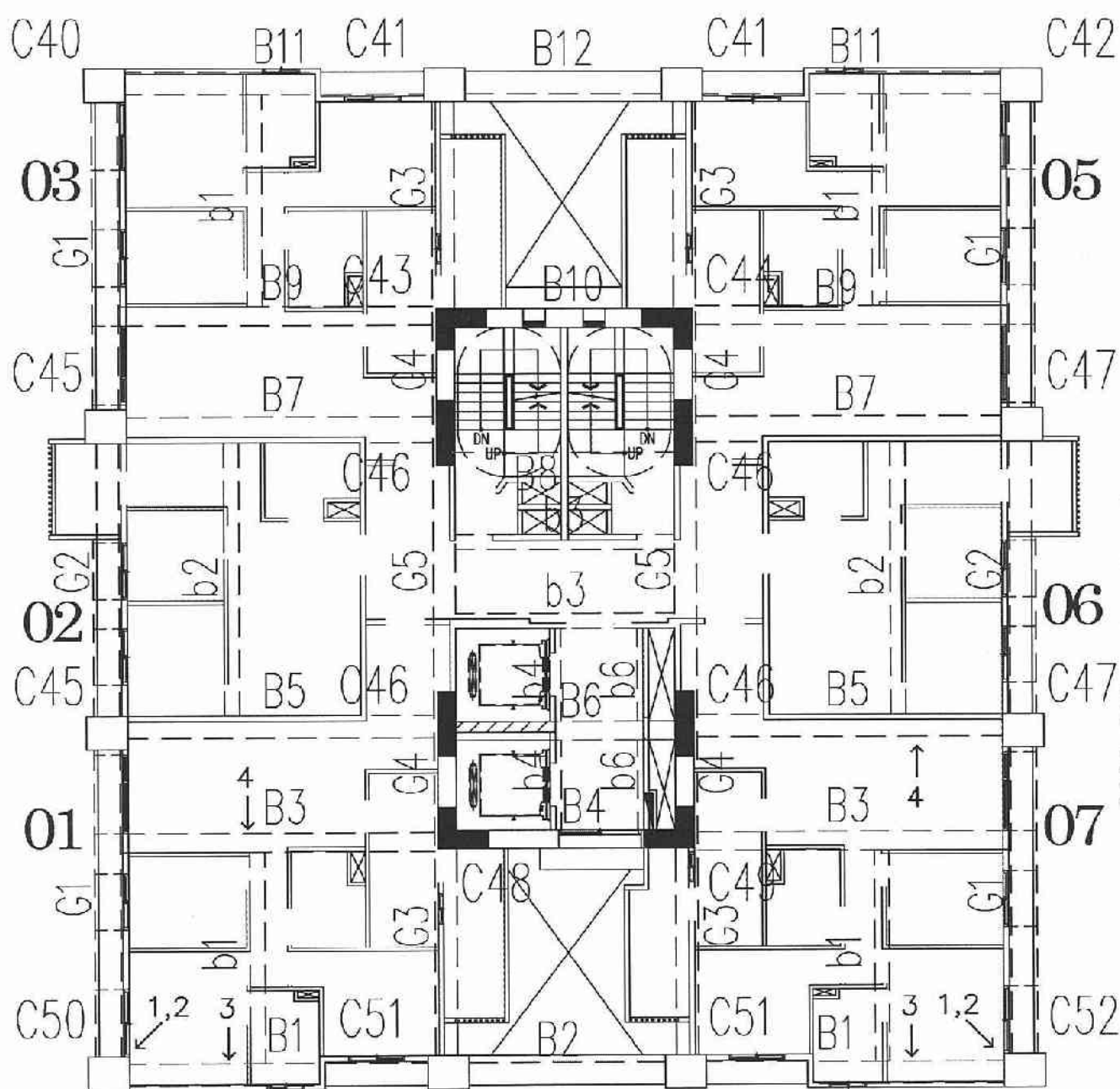
A6區H棟21層照片平面位置示意圖
