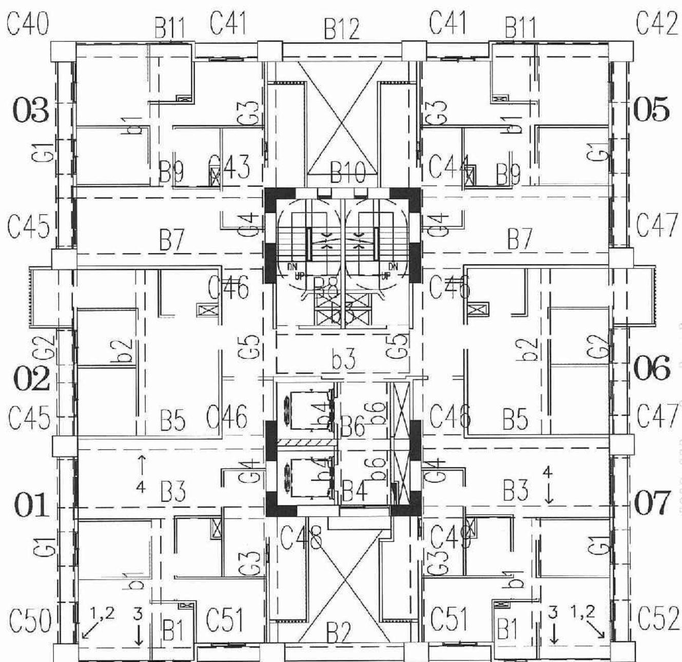
A6區H棟19層照片平面位置示意圖
