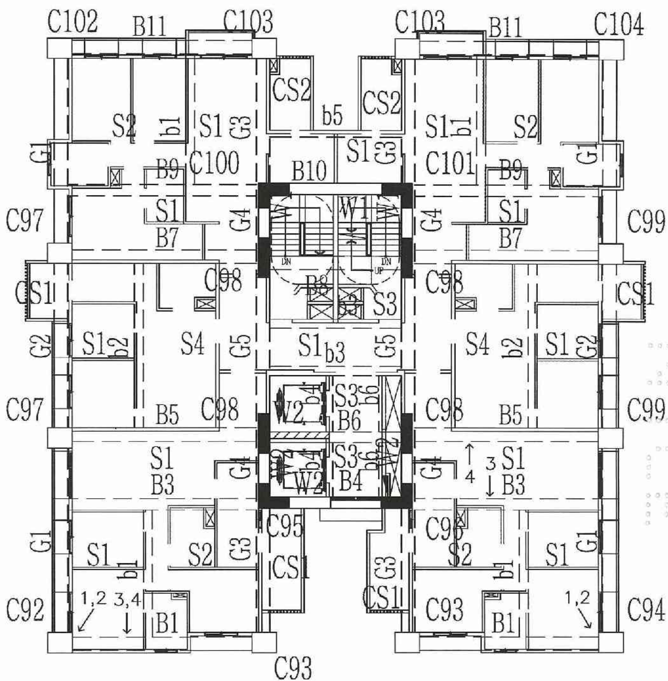
A6區G棟3層照片平面位置示意圖
