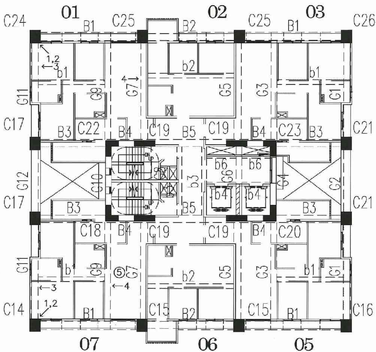
A6區F棟8層照片平面位置示意圖
