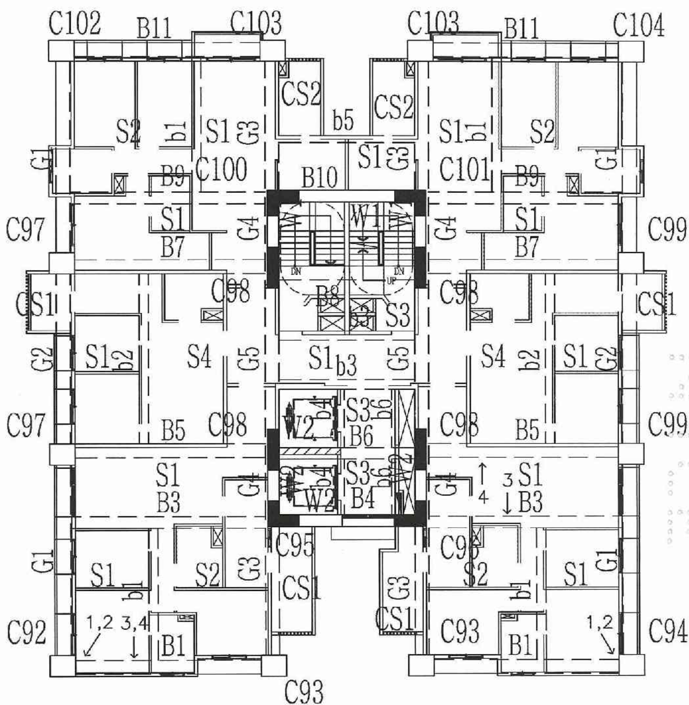
A6區G棟9層照片平面位置示意圖
