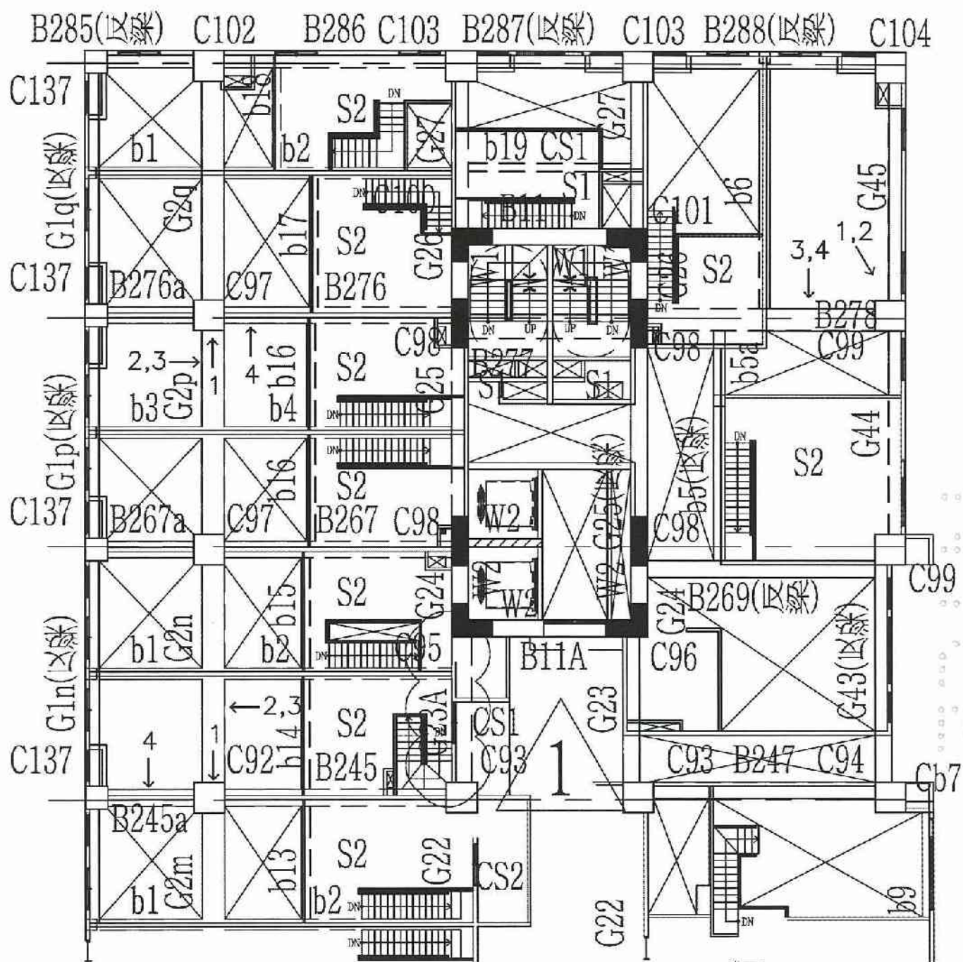
A6區G棟1照片平面位置示意圖
