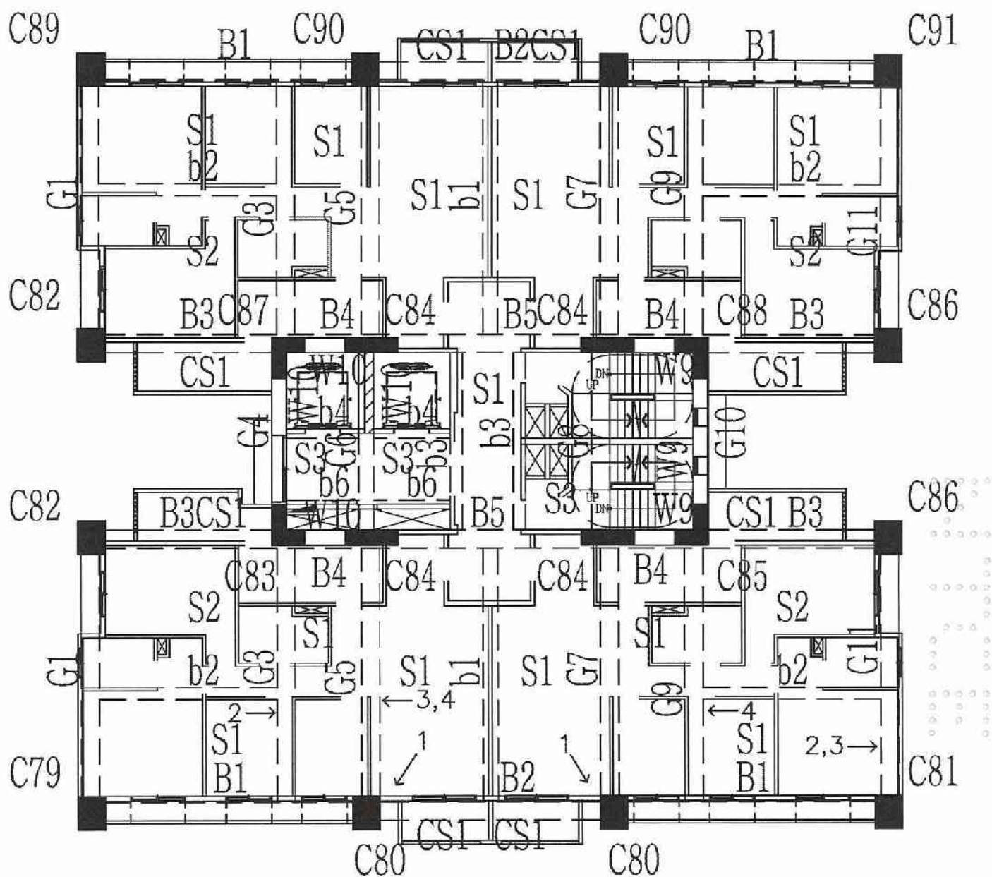
A6區E棟5層照片平面位置示意圖
