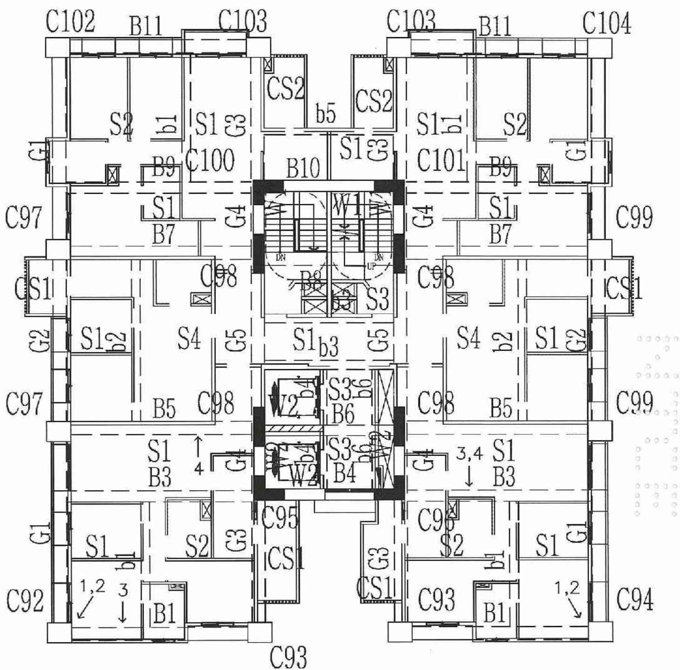
A6區G棟17層照片平面位置示意圖
