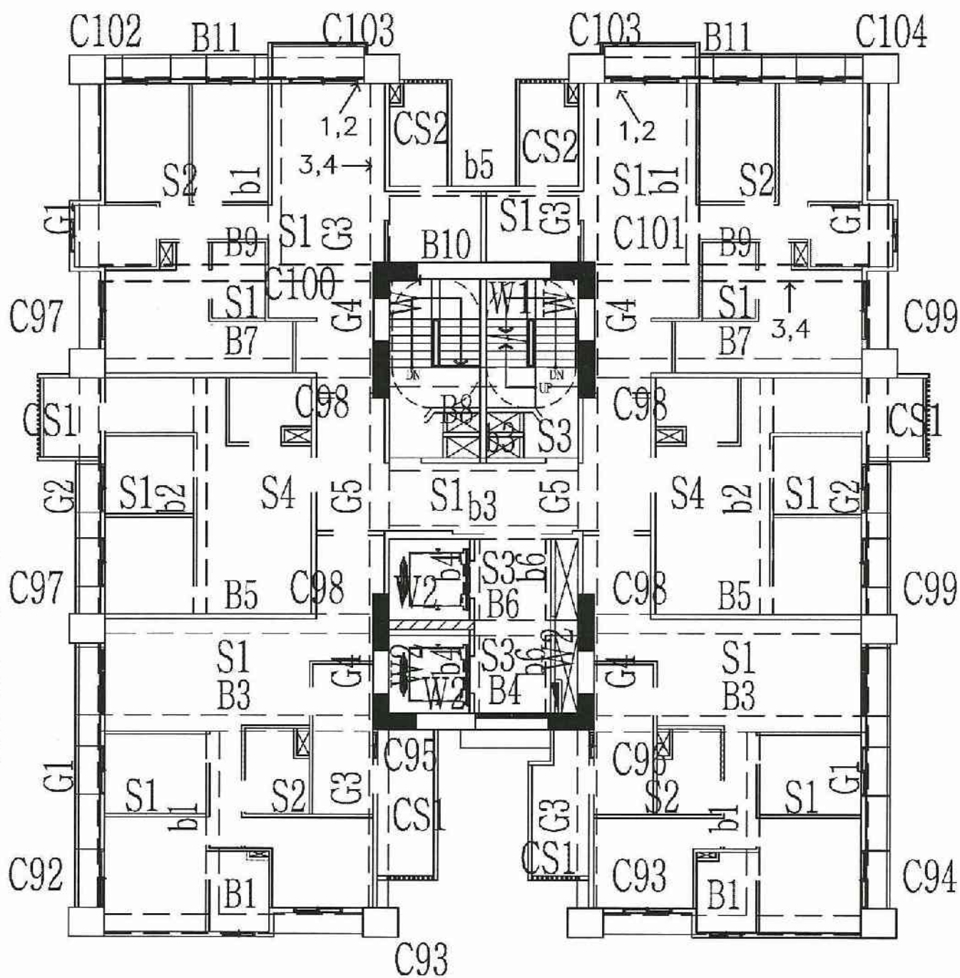
A6區G棟6層照片平面位置示意圖
