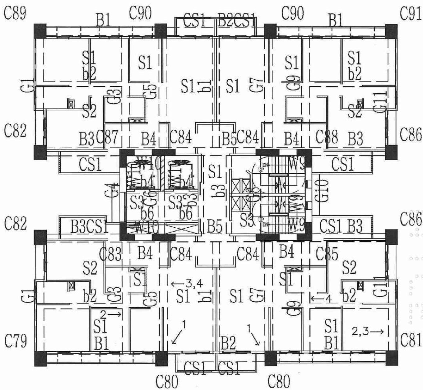
A6區E棟15層照片平面位置示意圖
