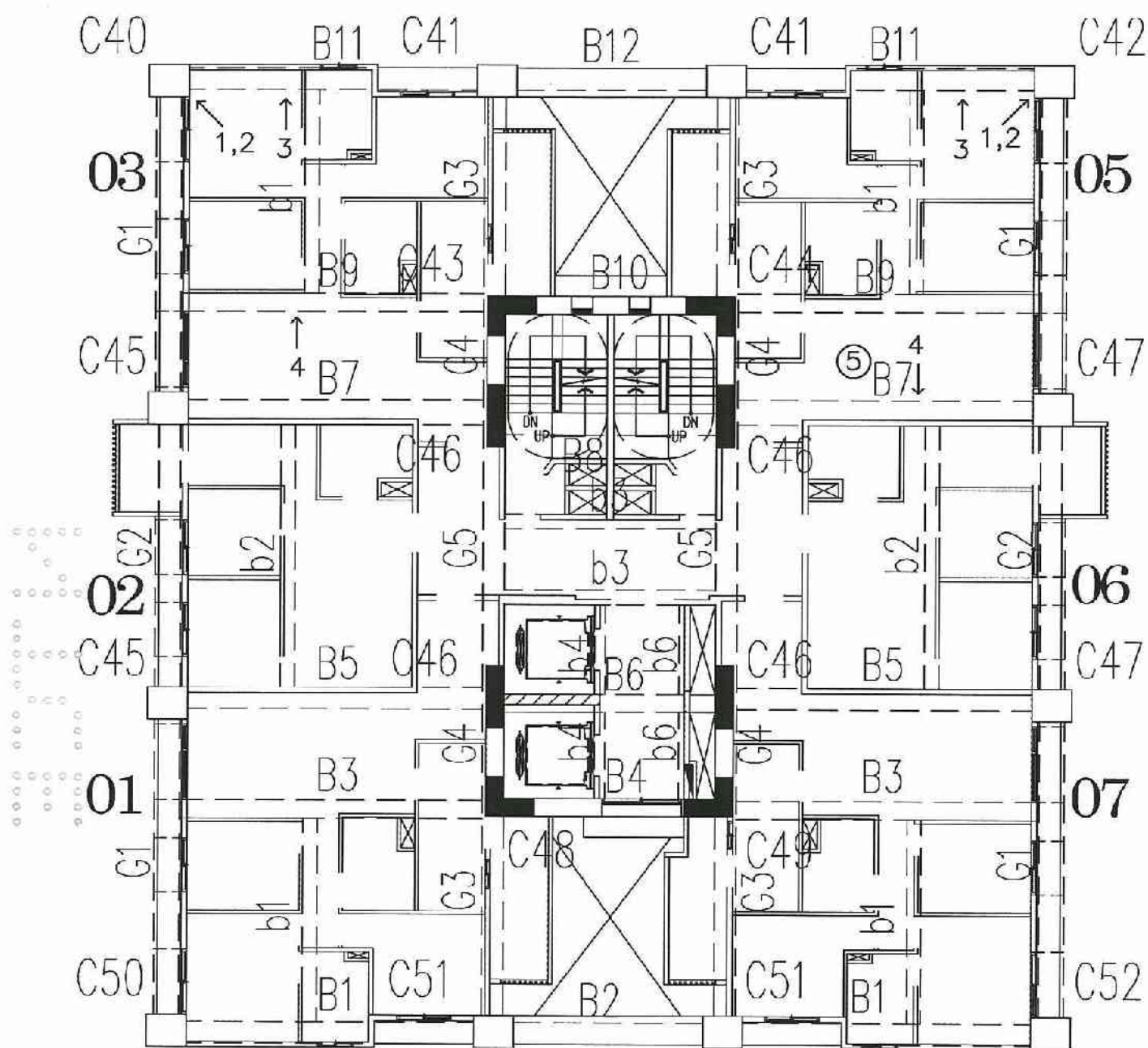
A6區H棟10層照片平面位置示意圖
