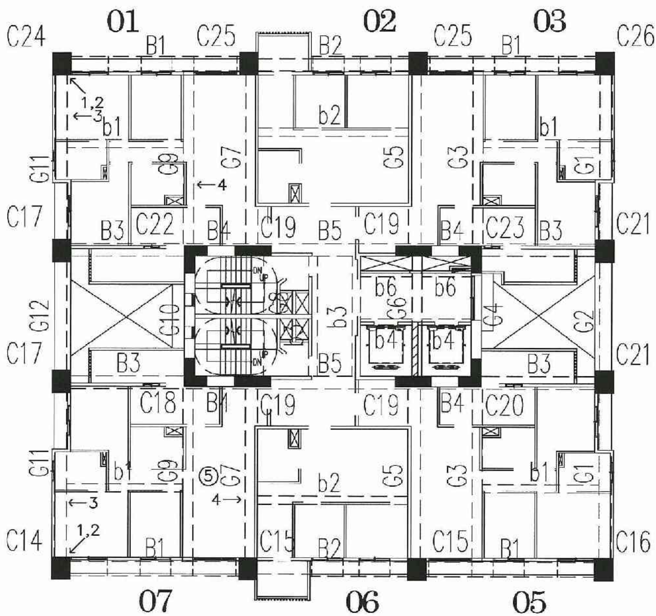
A6區F棟24層照片平面位置示意圖
