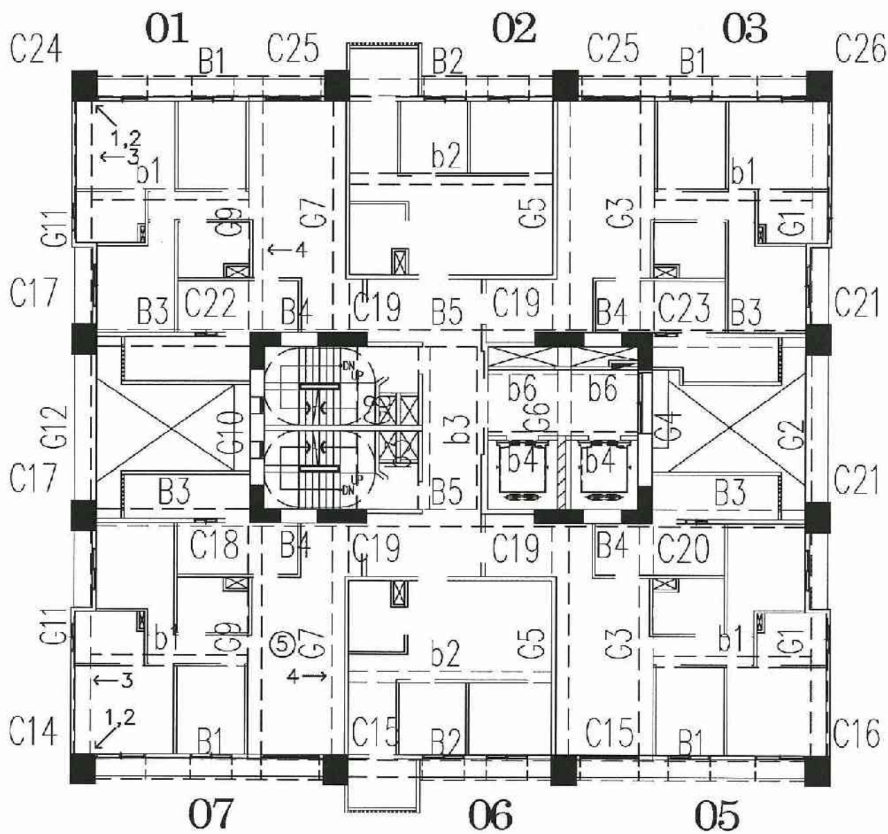
A6區F棟22層照片平面位置示意圖
