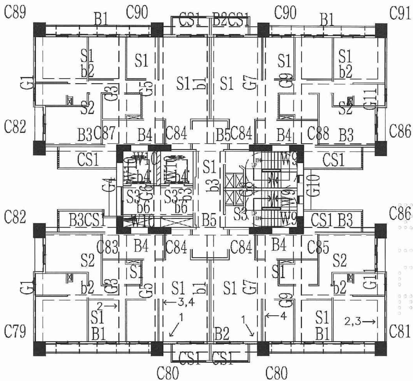
A6區E棟17層照片平面位置示意圖
