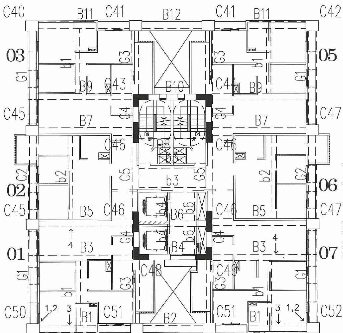
A6區H棟17層照片平面位置示意圖
