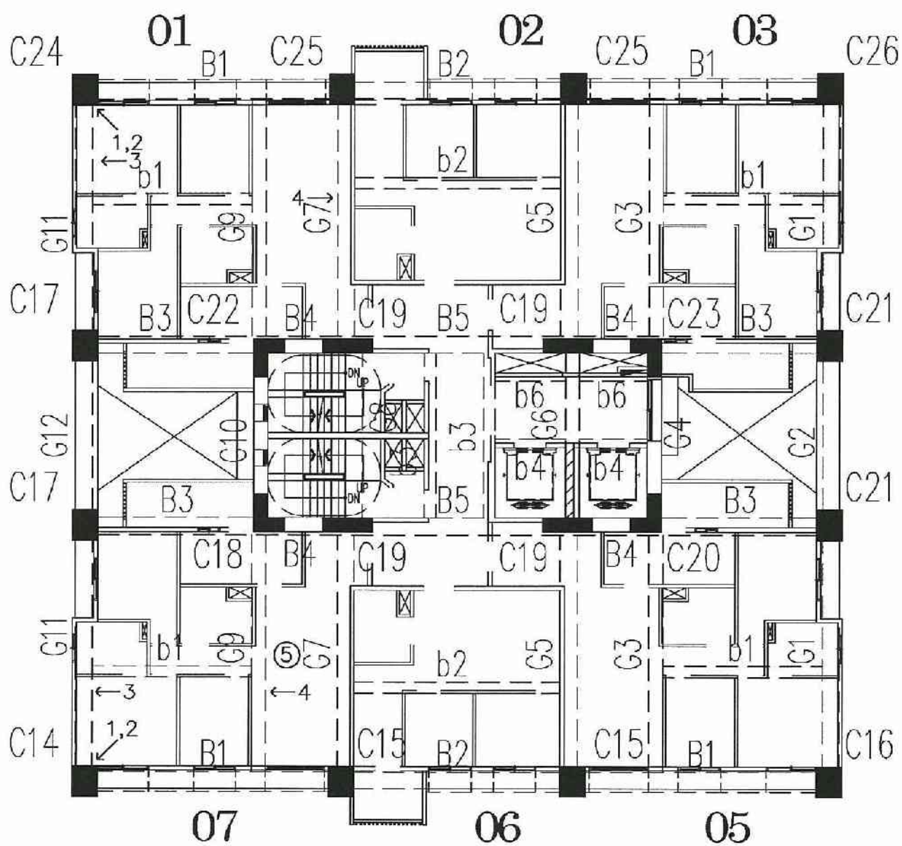
A6區F棟2層照片平面位置示意圖
