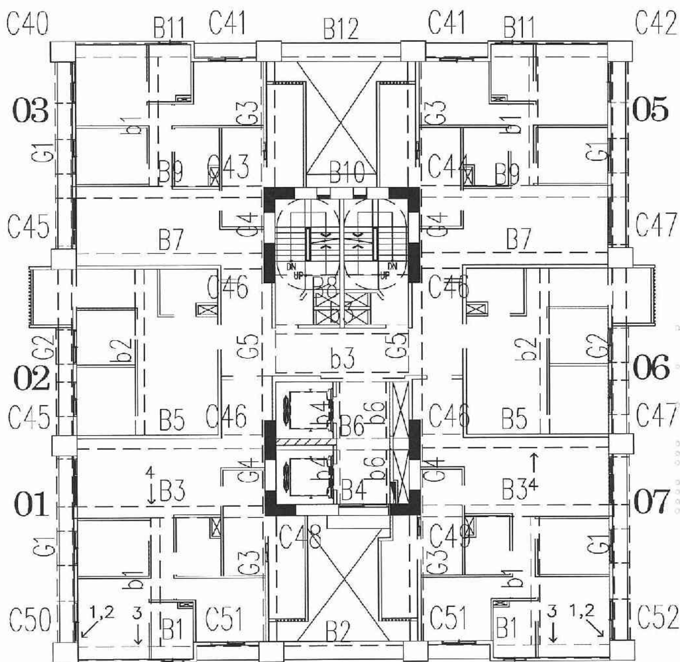
A6區H棟7層照片平面位置示意圖
