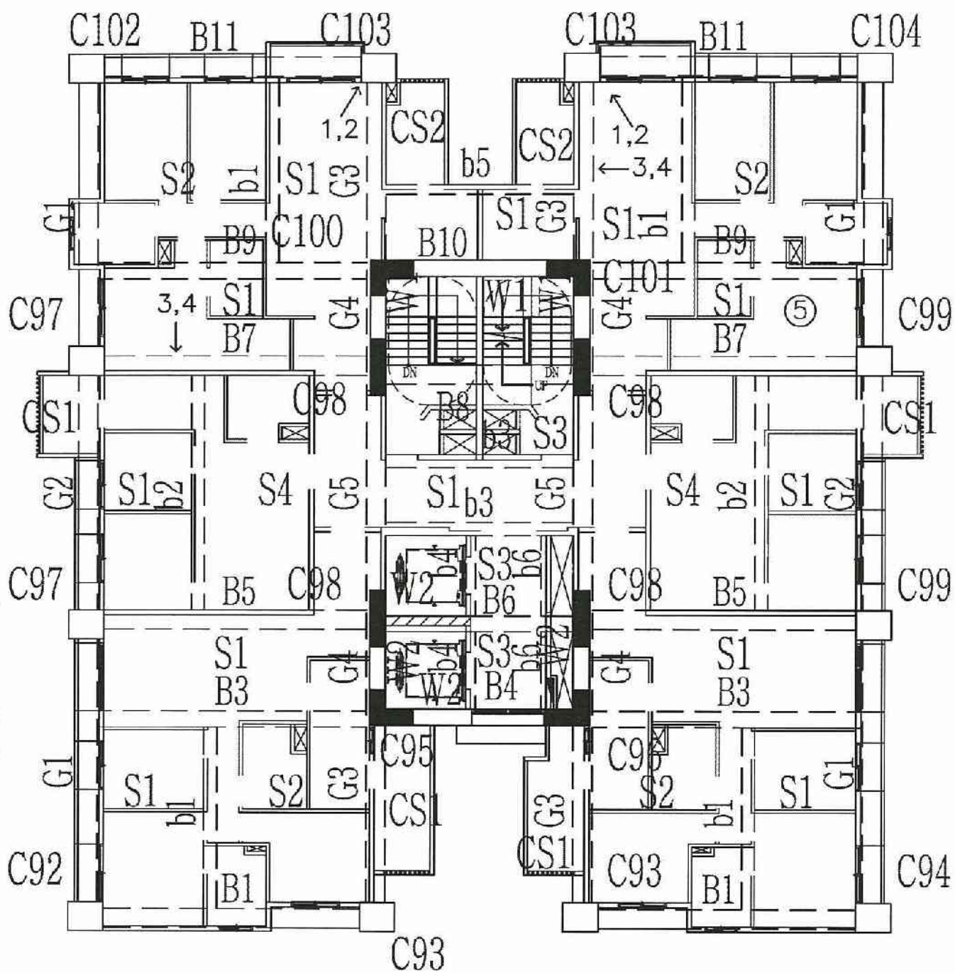
A6區G棟12層照片平面位置示意圖
