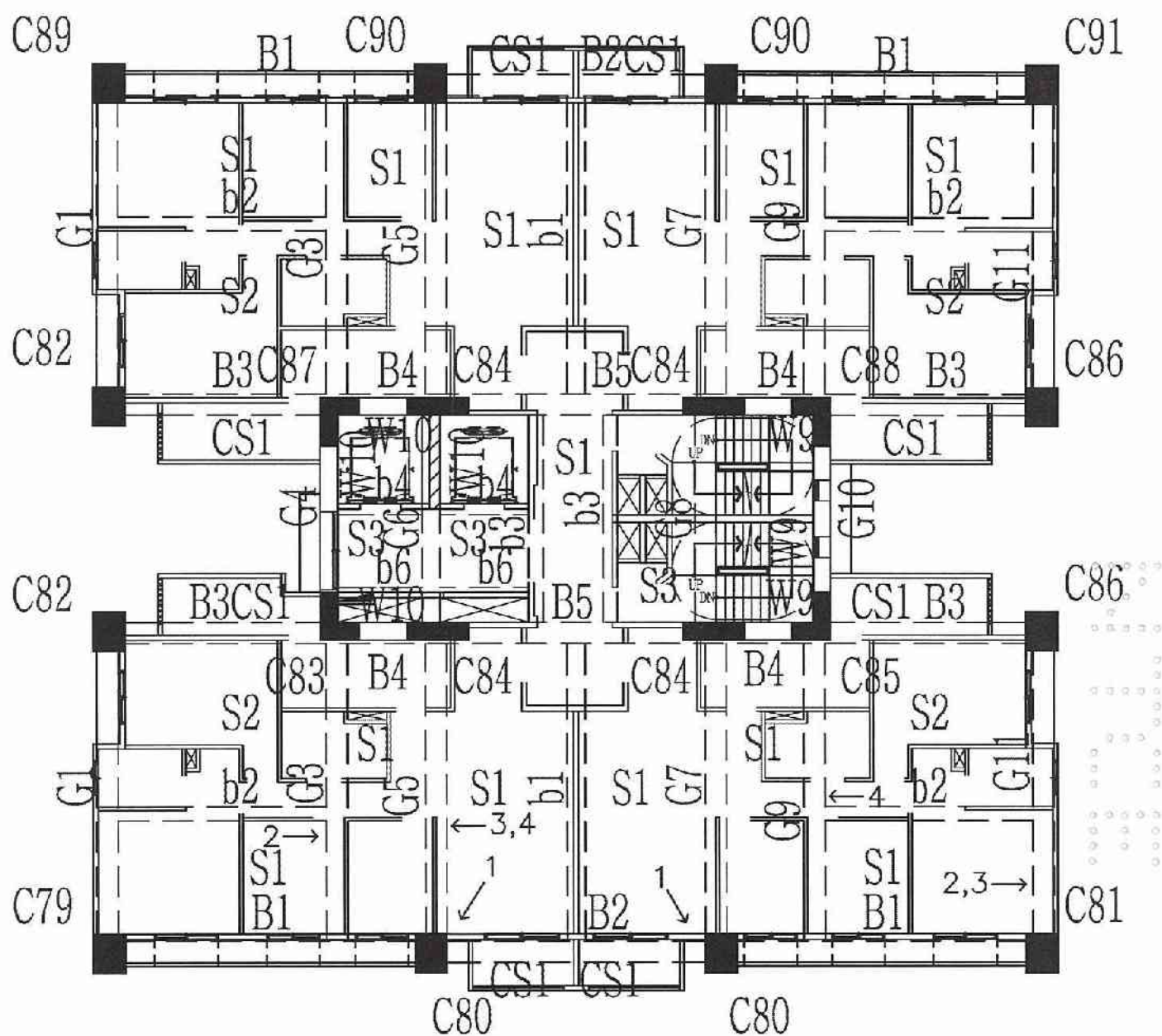
A6區E棟3層照片平面位置示意圖
