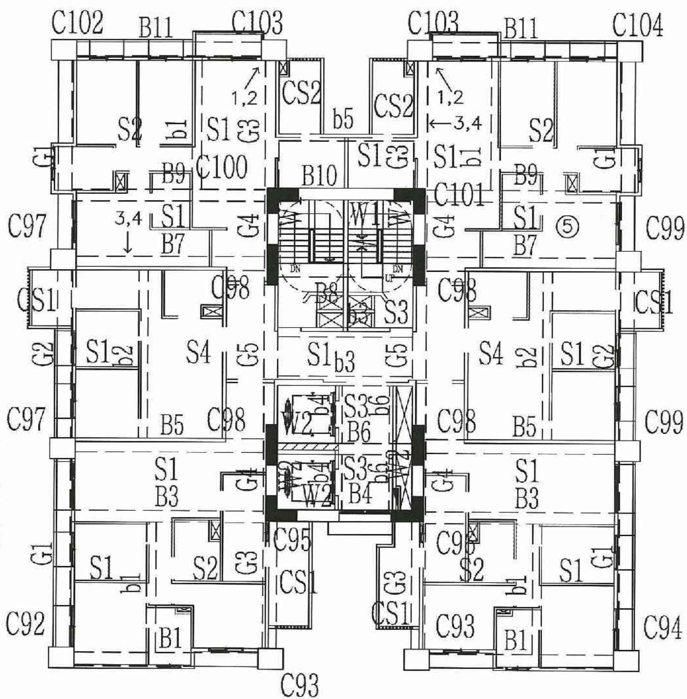
A6區G棟20層照片平面位置示意圖
