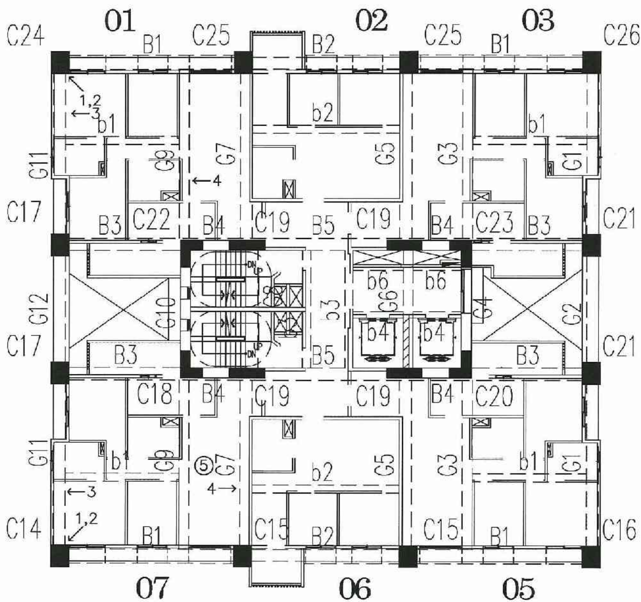
A6區F棟16層照片平面位置示意圖
