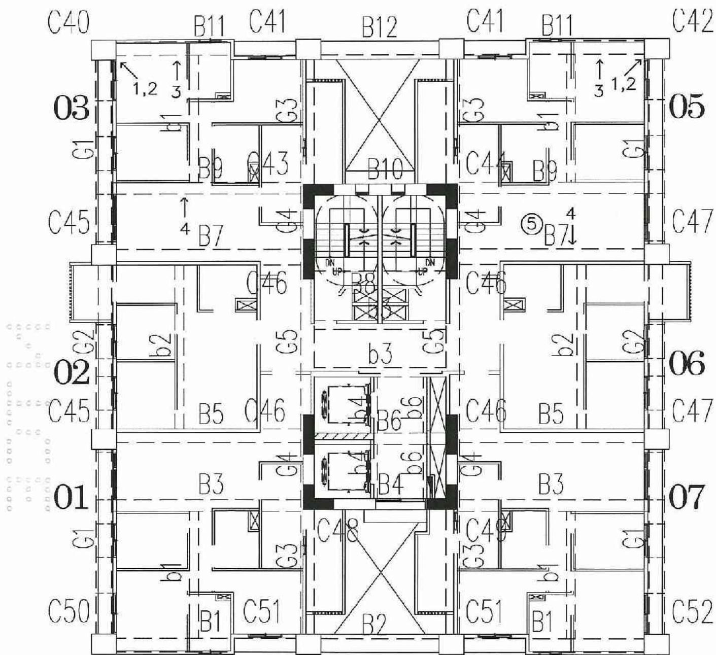
A6區H棟14層照片平面位置示意圖
