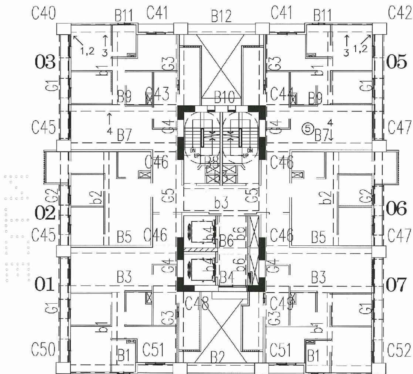
A6區H棟22層照片平面位置示意圖
