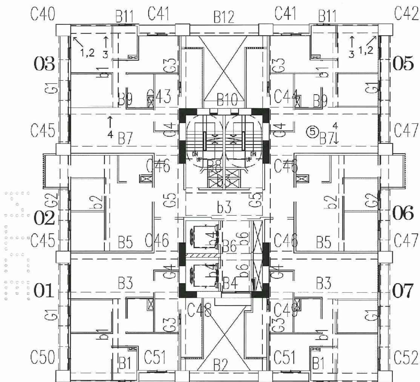
A6區H棟4層照片平面位置示意圖
