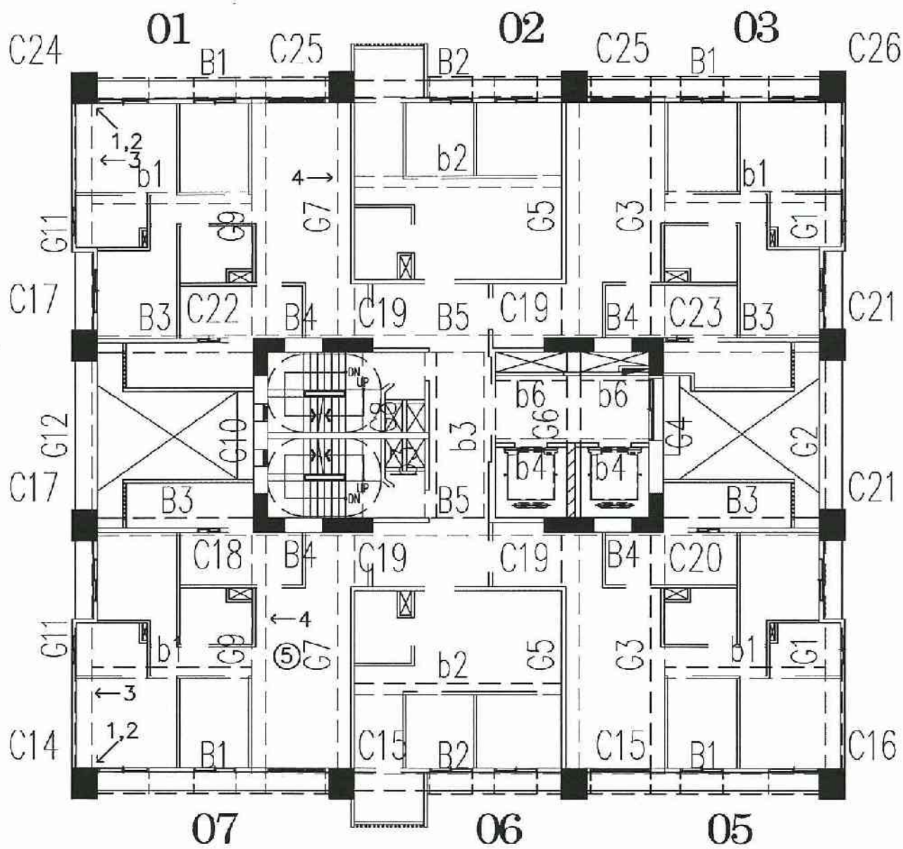
A6區F棟20層照片平面位置示意圖
