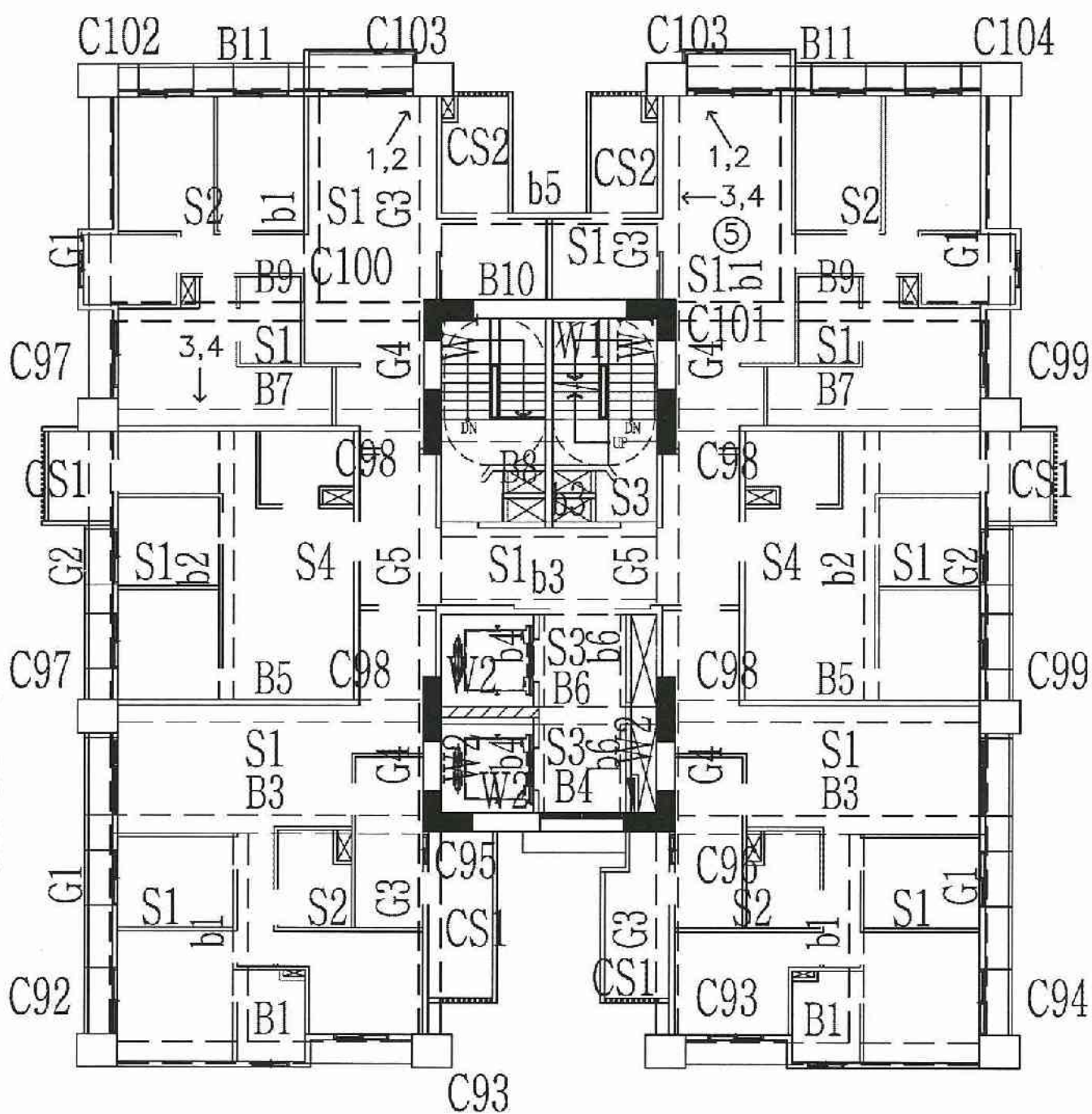
A6區G棟4層照片平面位置示意圖
