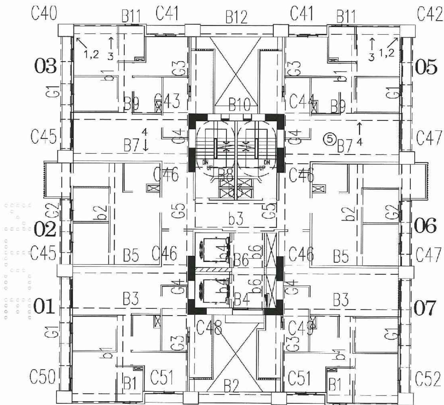
A6區H棟16層照片平面位置示意圖
