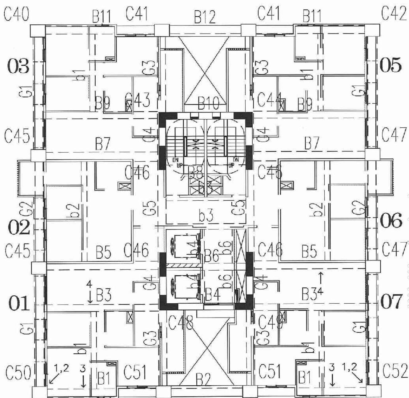
A6區H棟11層照片平面位置示意圖
