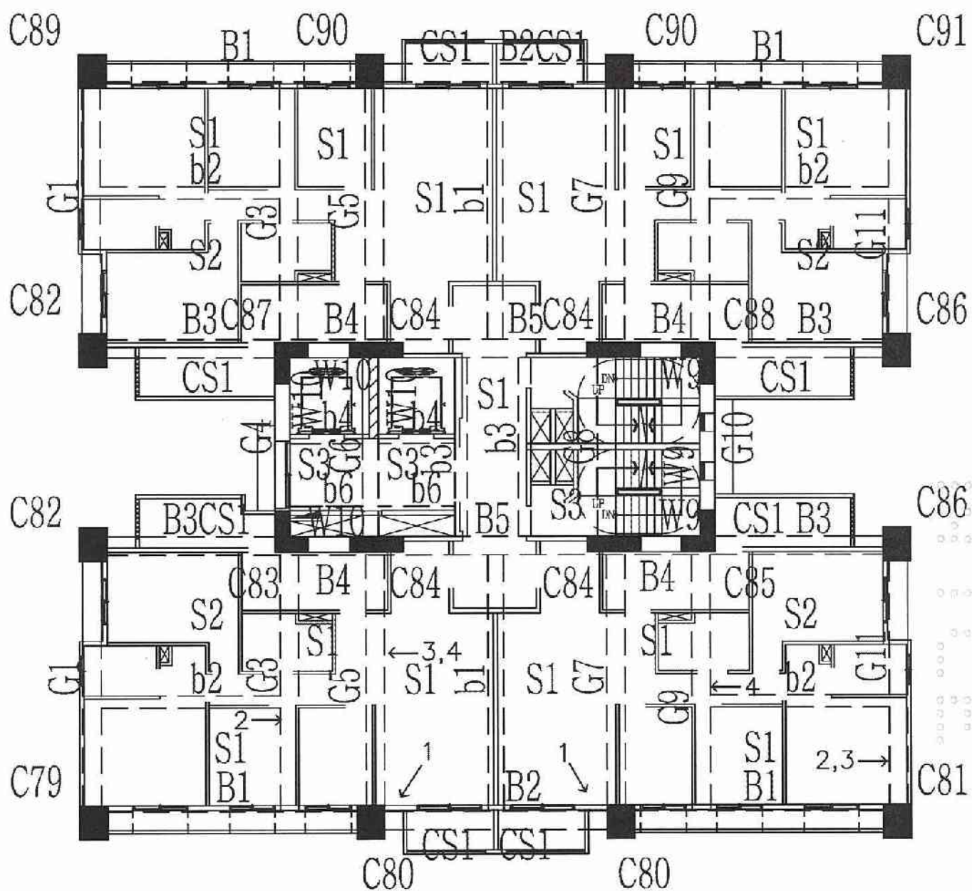
A6區E棟19層照片平面位置示意圖
