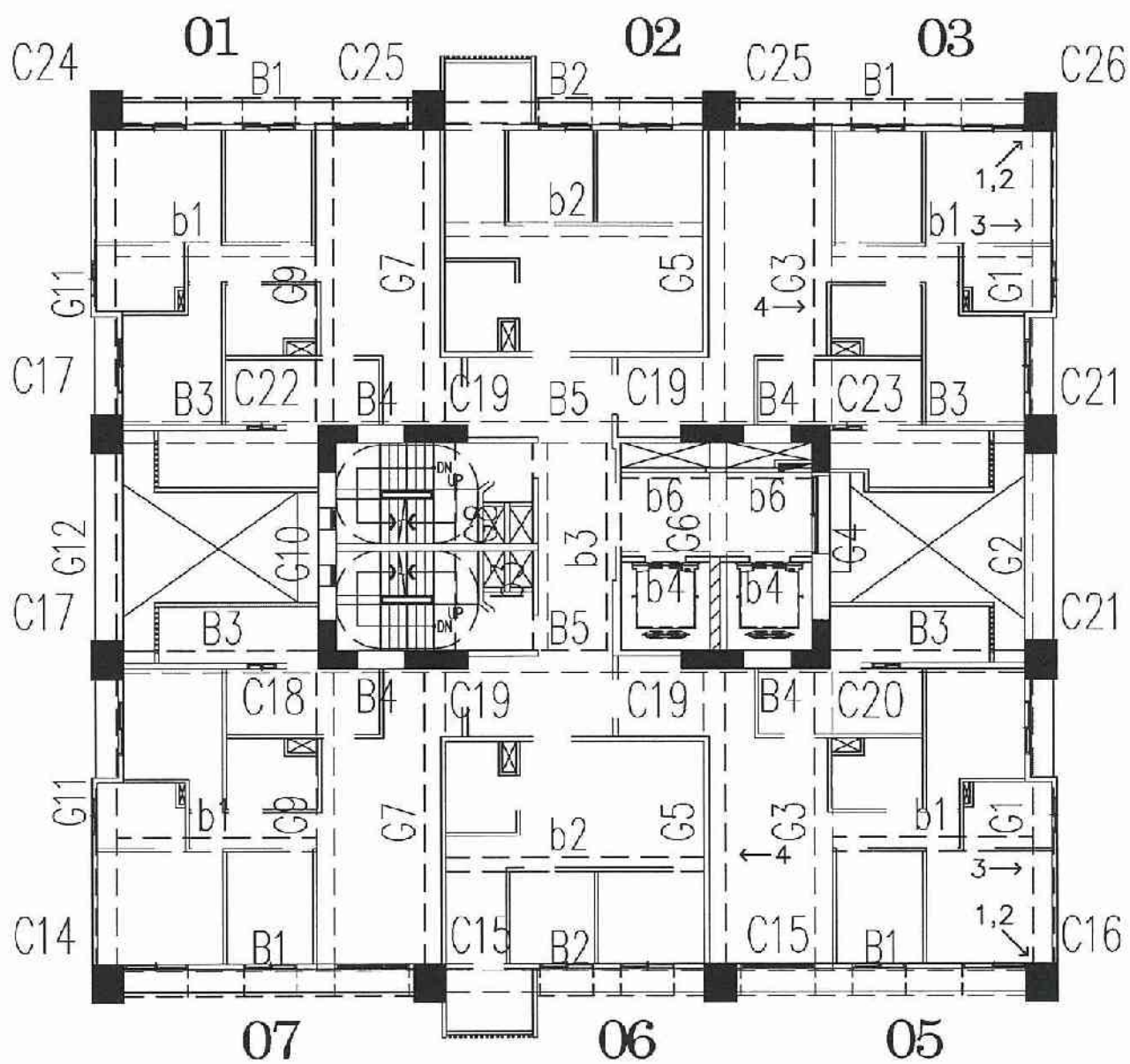
A6區F棟7層照片平面位置示意圖
