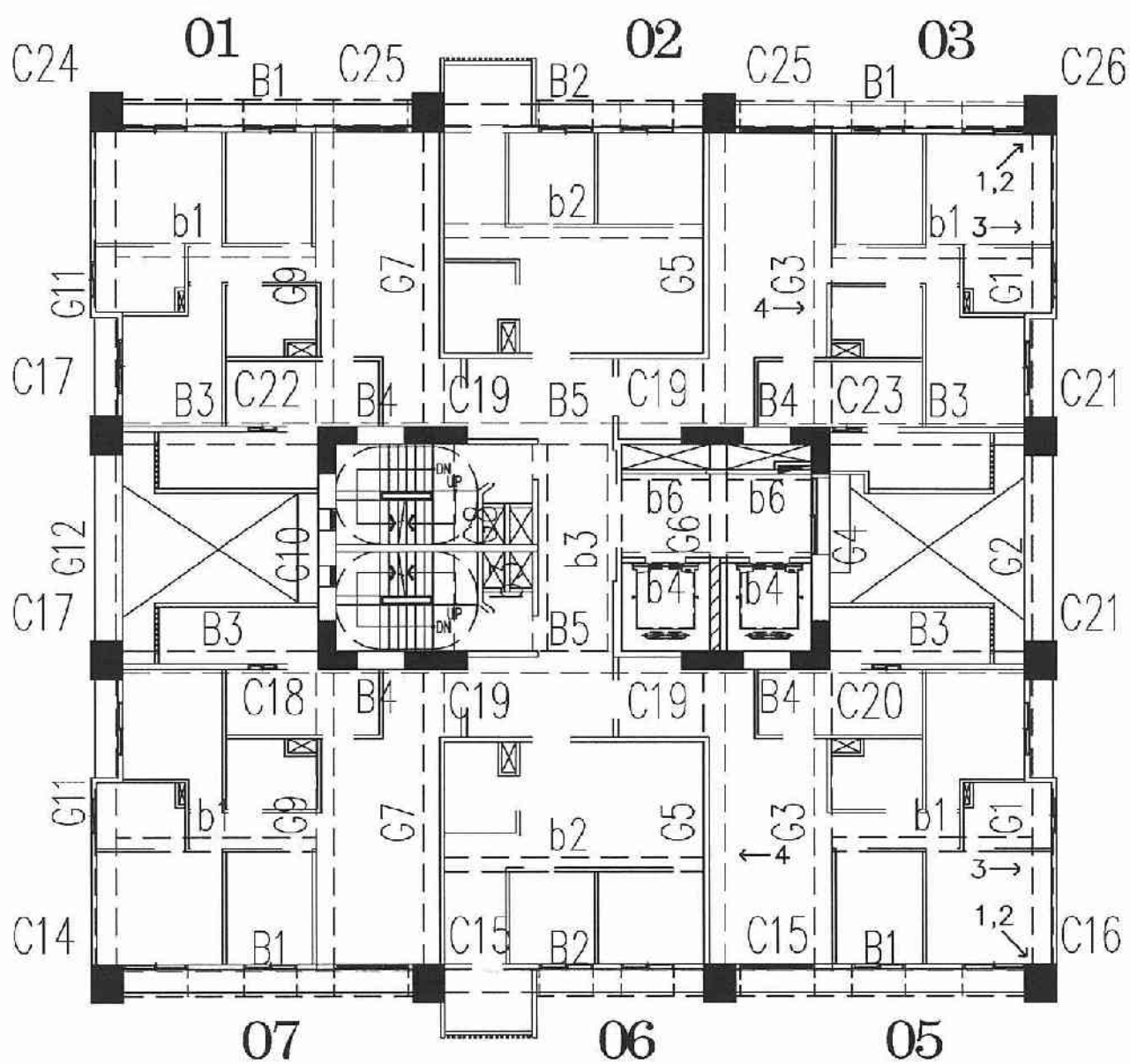
A6區F棟3層照片平面位置示意圖
