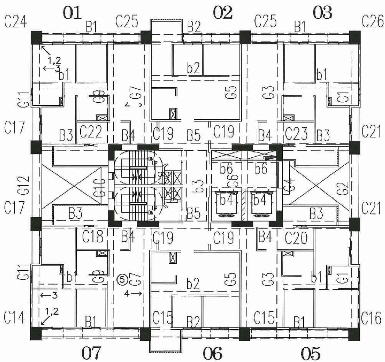
A6區F棟4層照片平面位置示意圖
