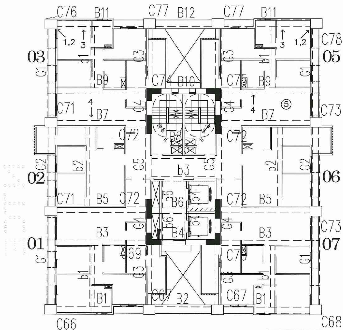
A6區B棟20層照片平面位置示意圖
