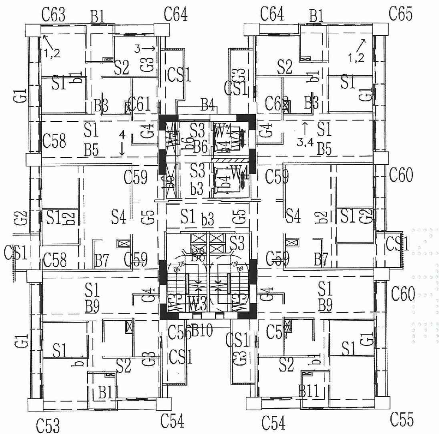
A6區C棟13層照片平面位置示意圖
