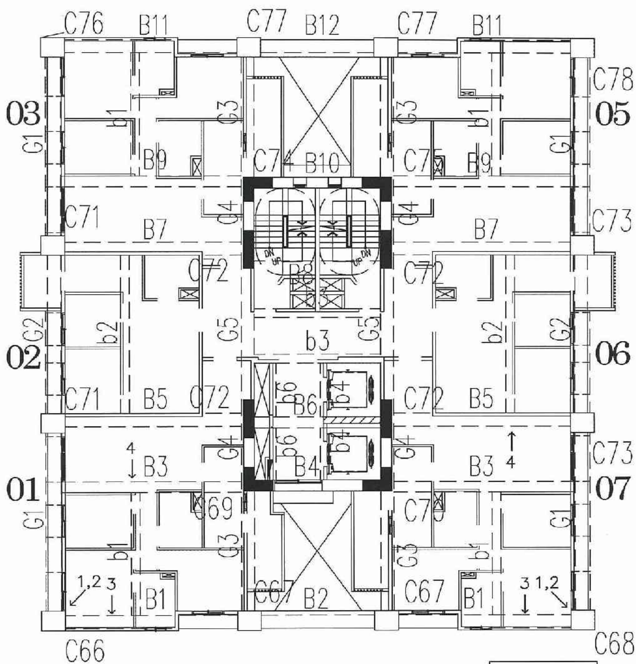
A6區B棟21層照片平面位置示意圖
