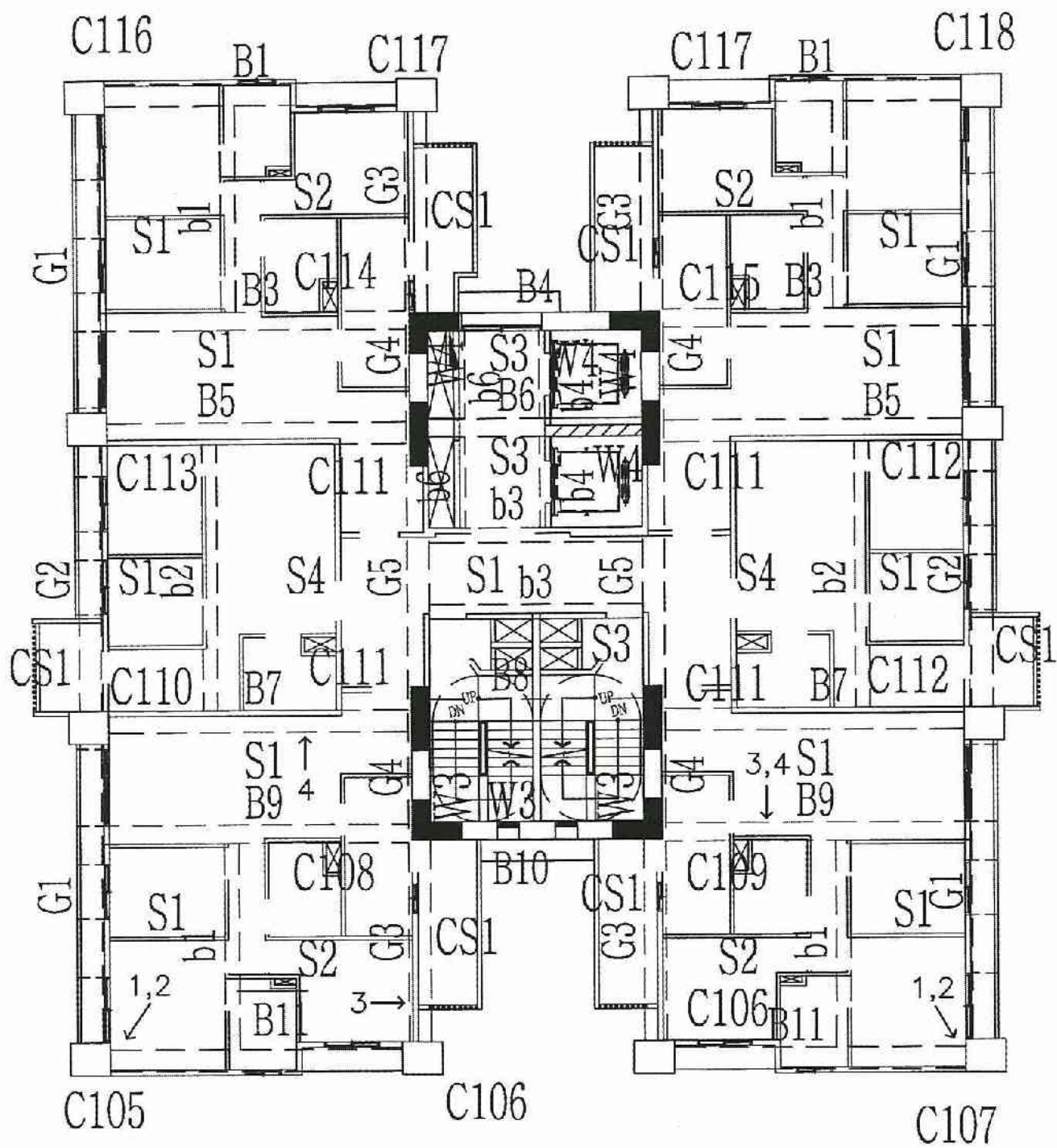
A6區A棟4層照片平面位置示意圖
