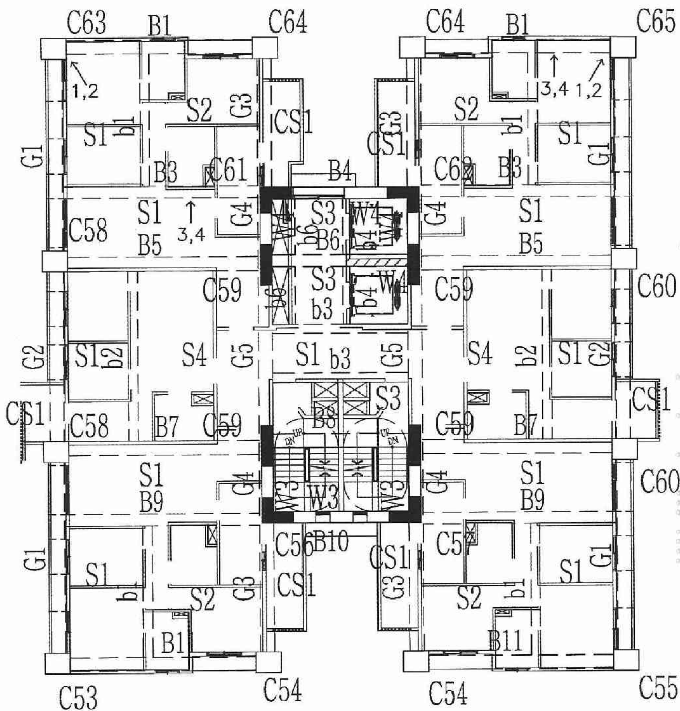
A6區C棟11層照片平面位置示意圖
