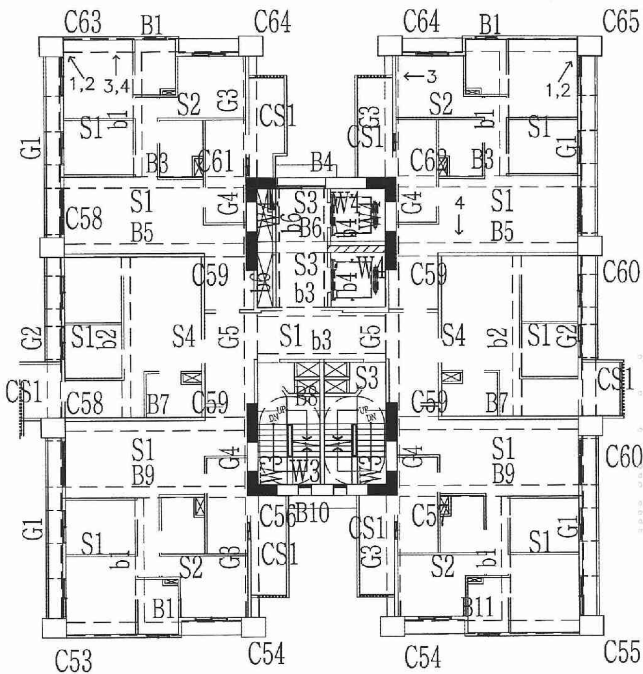
A6區C棟9層照片平面位置示意圖
