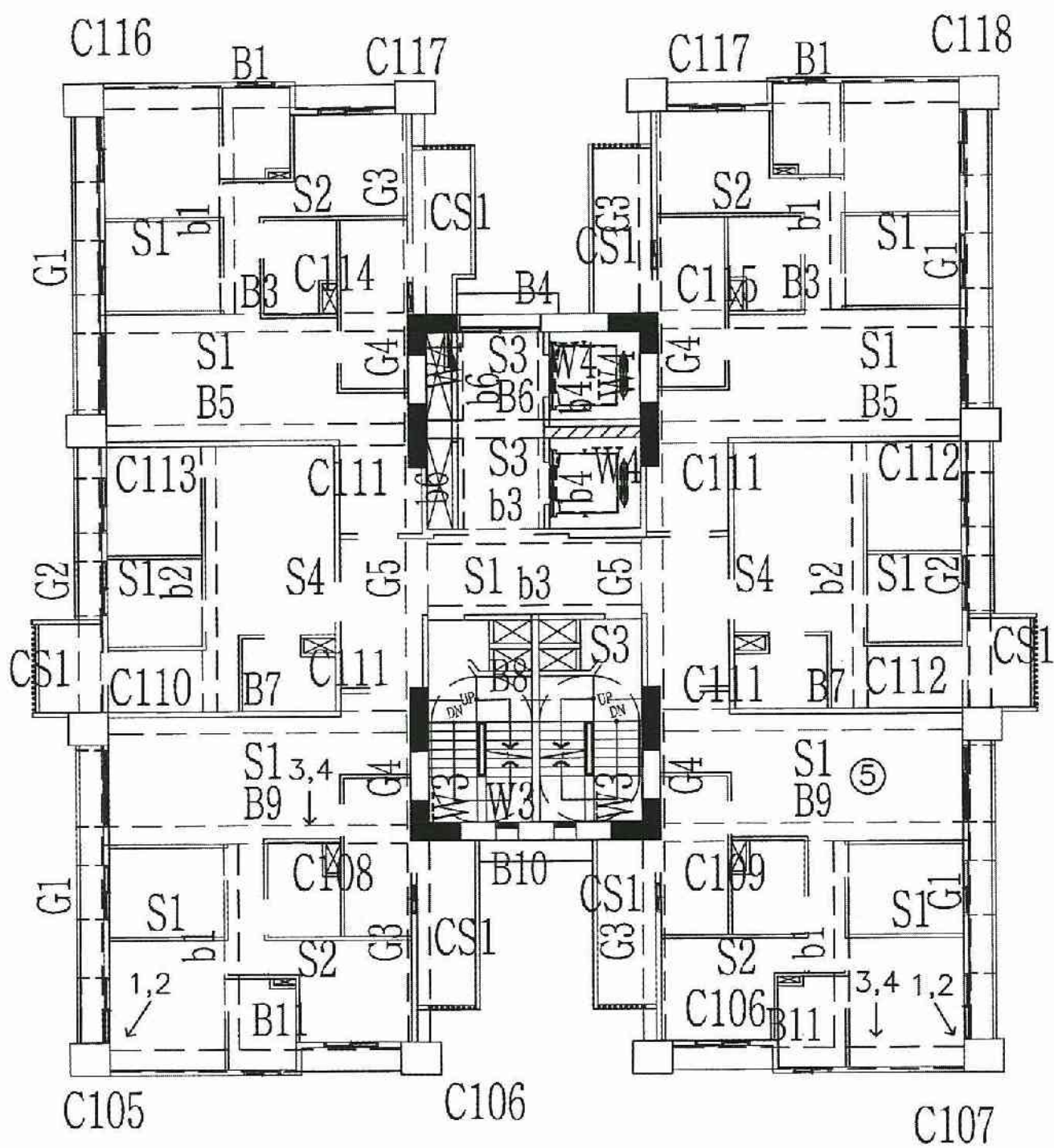
A6區A棟20層照片平面位置示意圖
