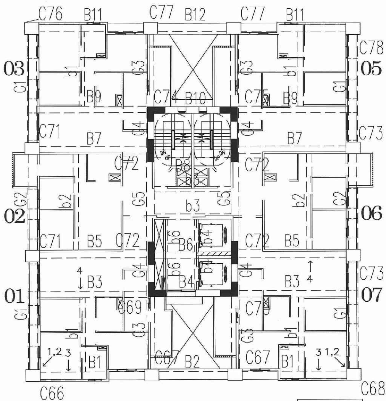
A6區B棟3層照片平面位置示意圖
