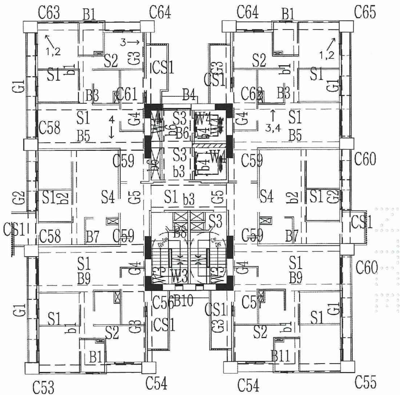
A6區C棟7層照片平面位置示意圖
