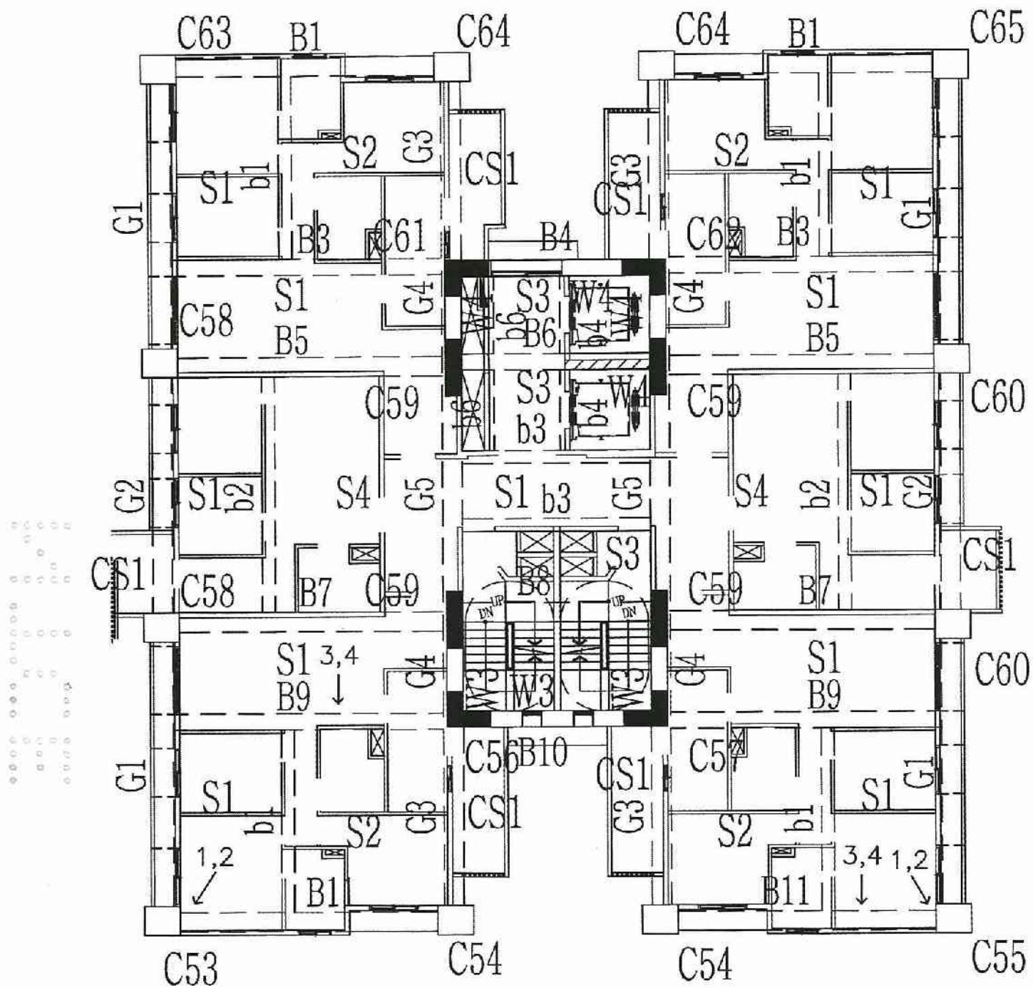
A6區C棟14層照片平面位置示意圖
