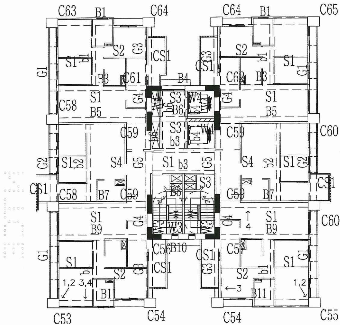
A6區C棟18層照片平面位置示意圖
