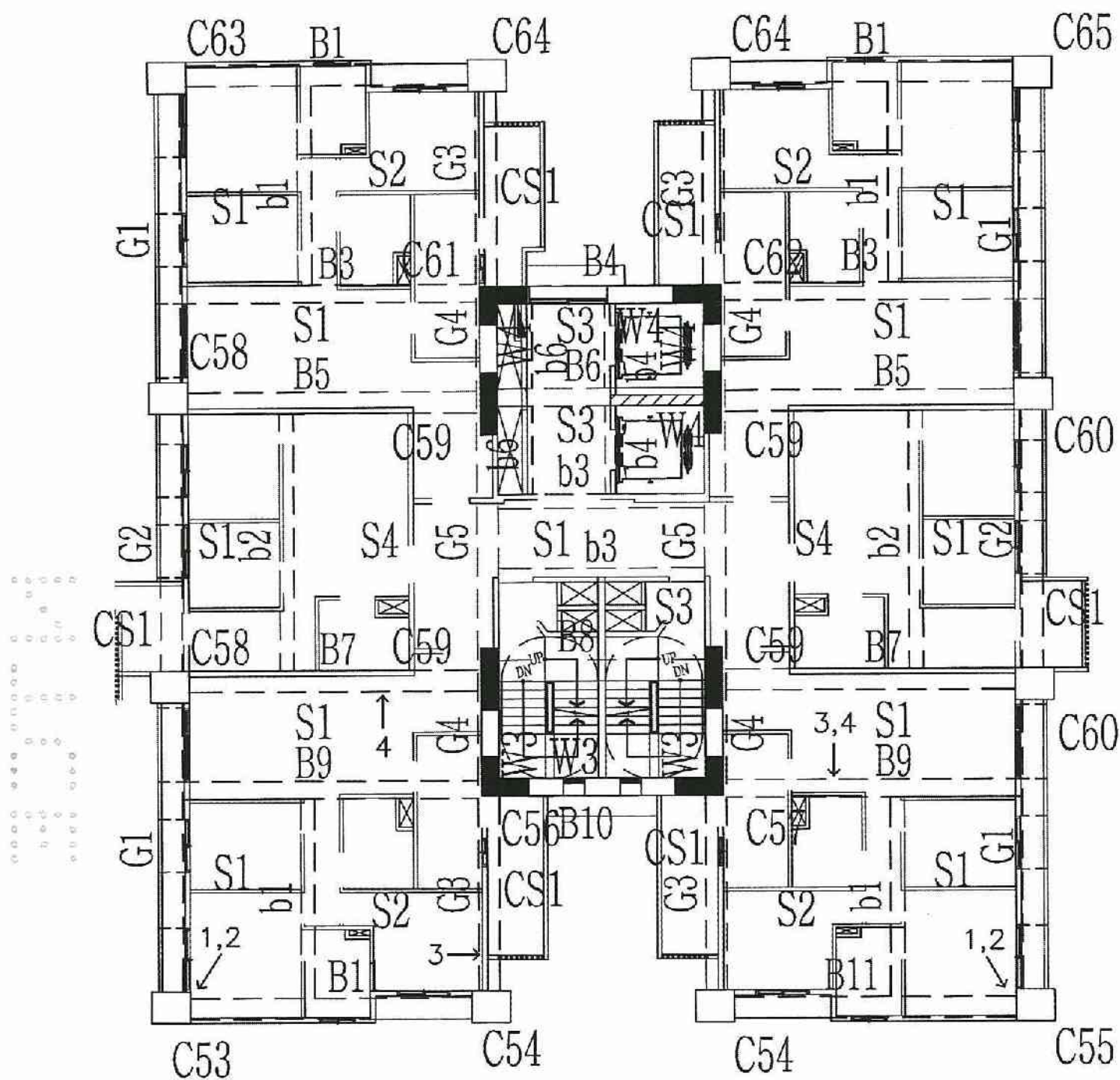
A6區C棟4層照片平面位置示意圖
