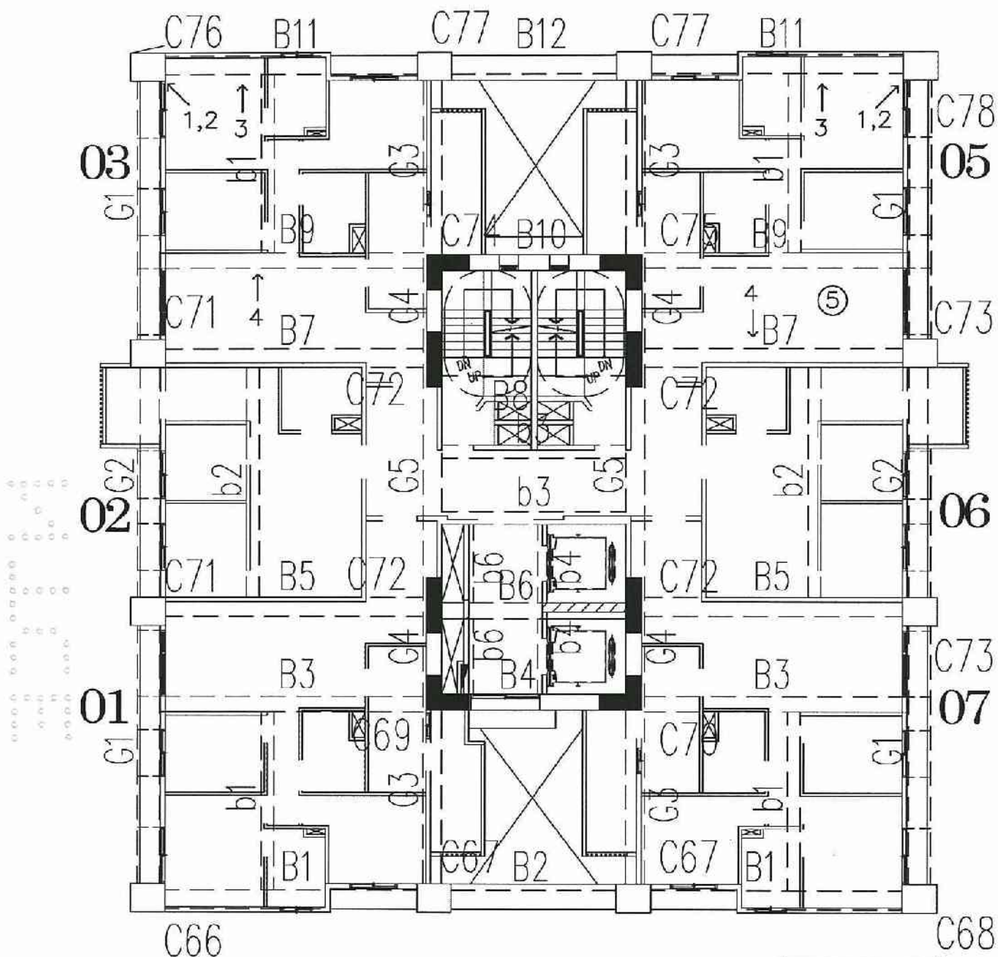
A6區B棟10層照片平面位置示意圖
