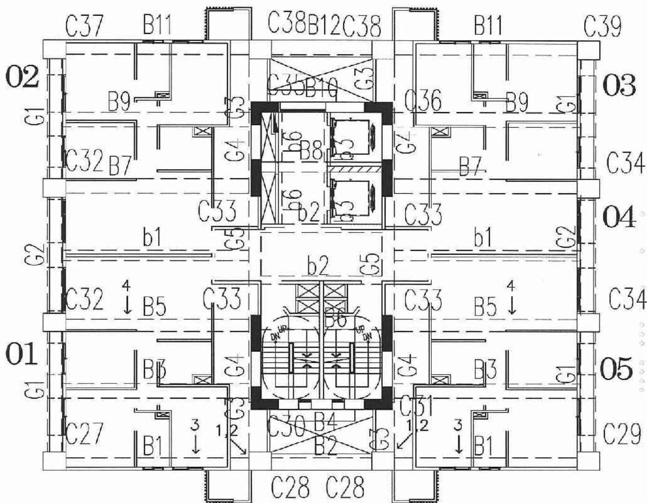
A6區D棟17層照片平面位置示意圖
