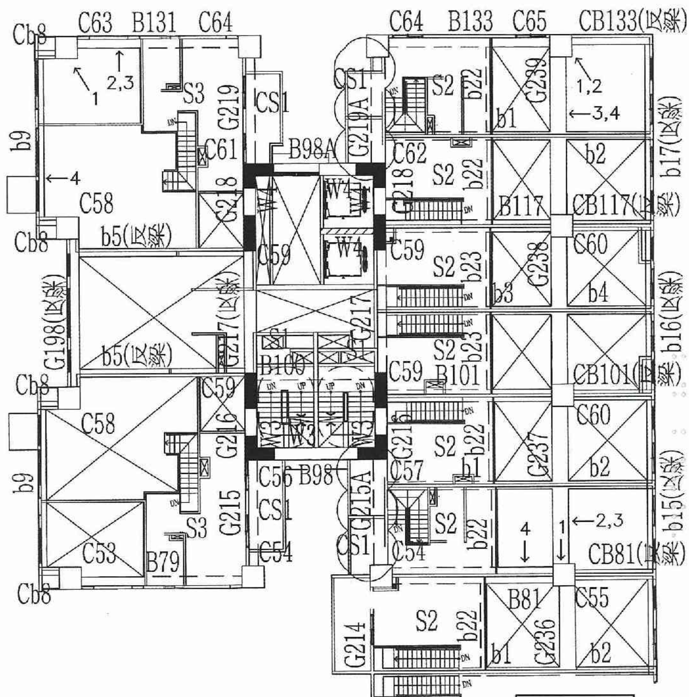
A6區C棟1層照片平面位置示意圖
