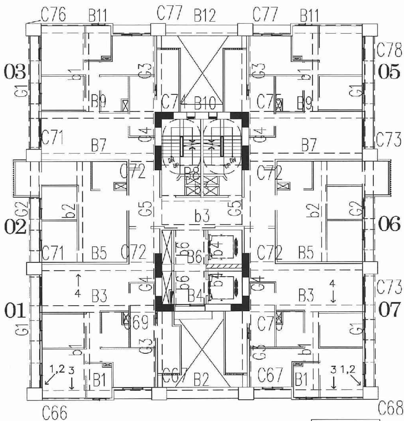
A區B棟7層照片平面位置示意圖
