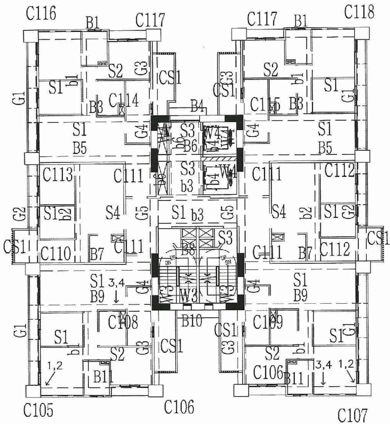
A6區A棟8層照片平面位置示意圖
