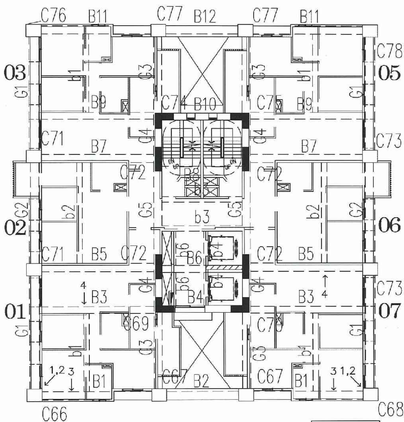
A6區B棟5層照片平面位置示意圖
