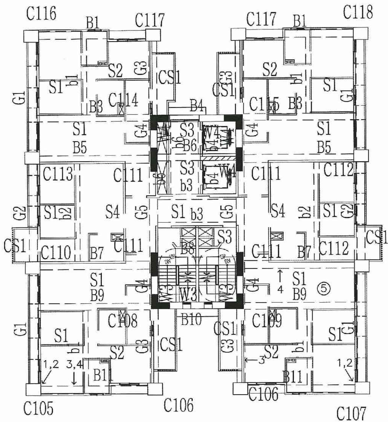
A6區A棟6層照片平面位置示意圖
