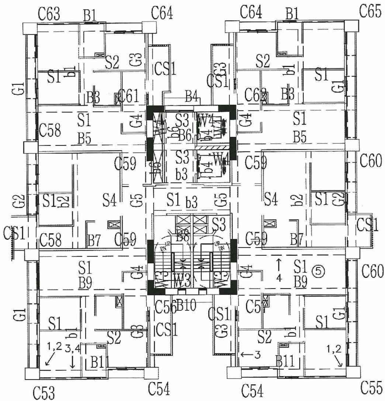
A6區C棟12層照片平面位置示意圖
