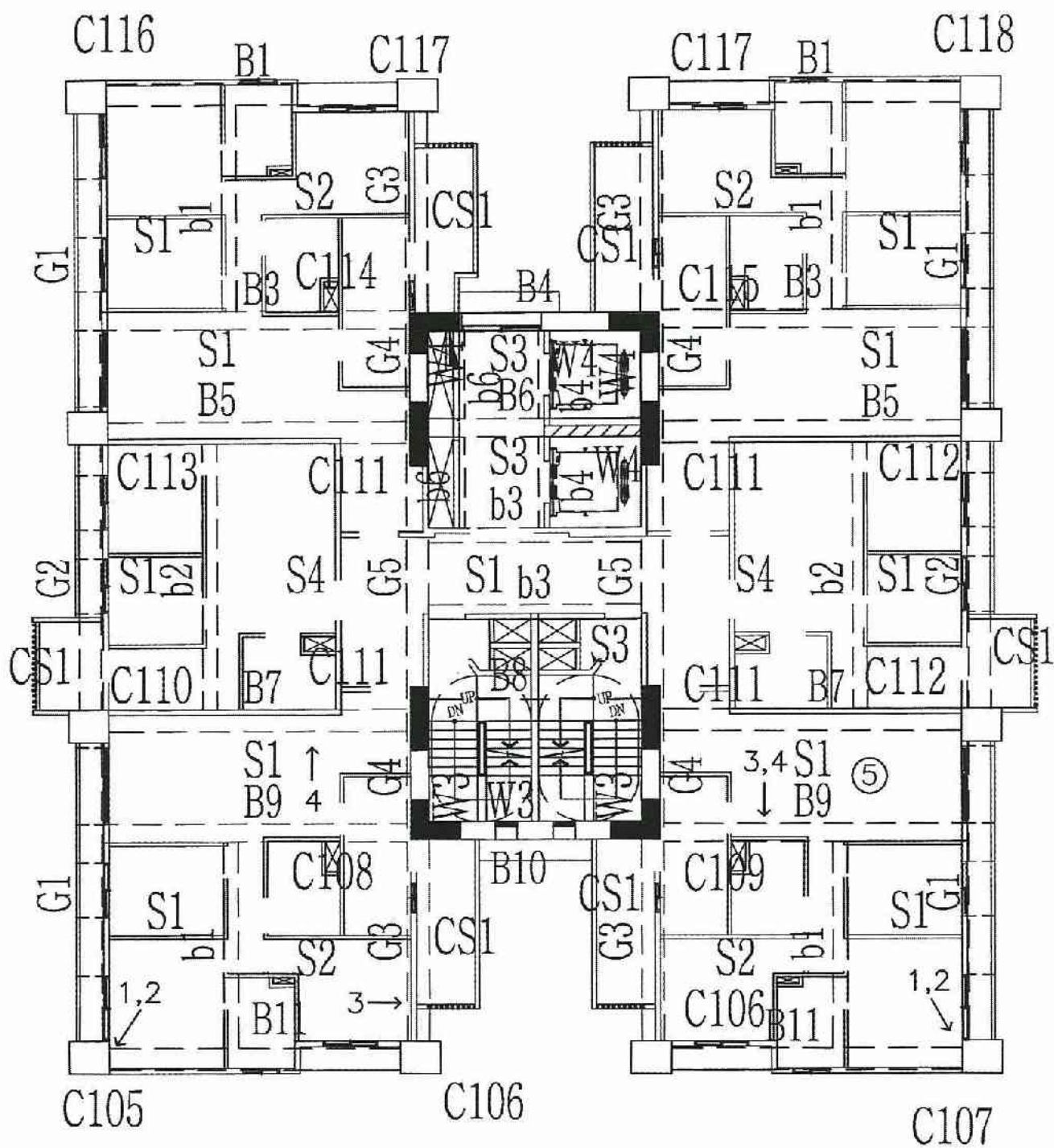
A6區A棟10層照片平面位置示意圖
