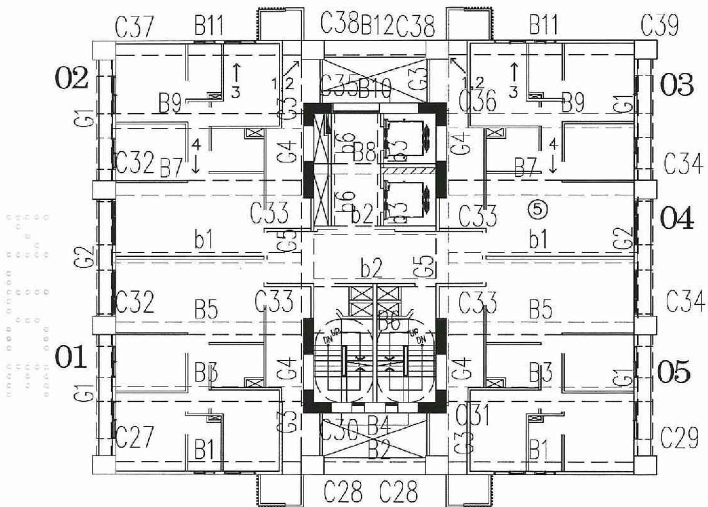
A6區D棟20層照片平面位置示意圖
