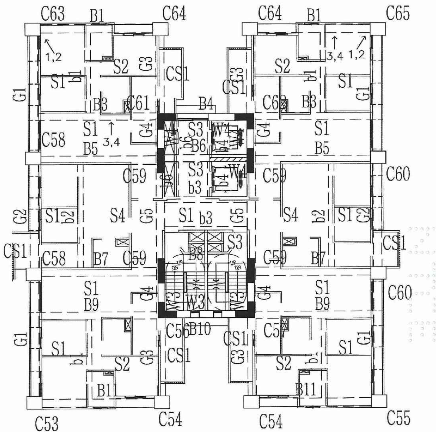
A6區C棟17層照片平面位置示意圖
