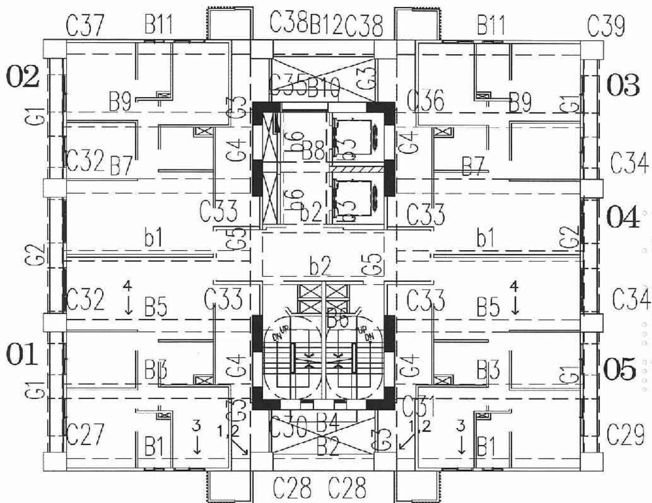
A6區D棟19層照片平面位置示意圖
