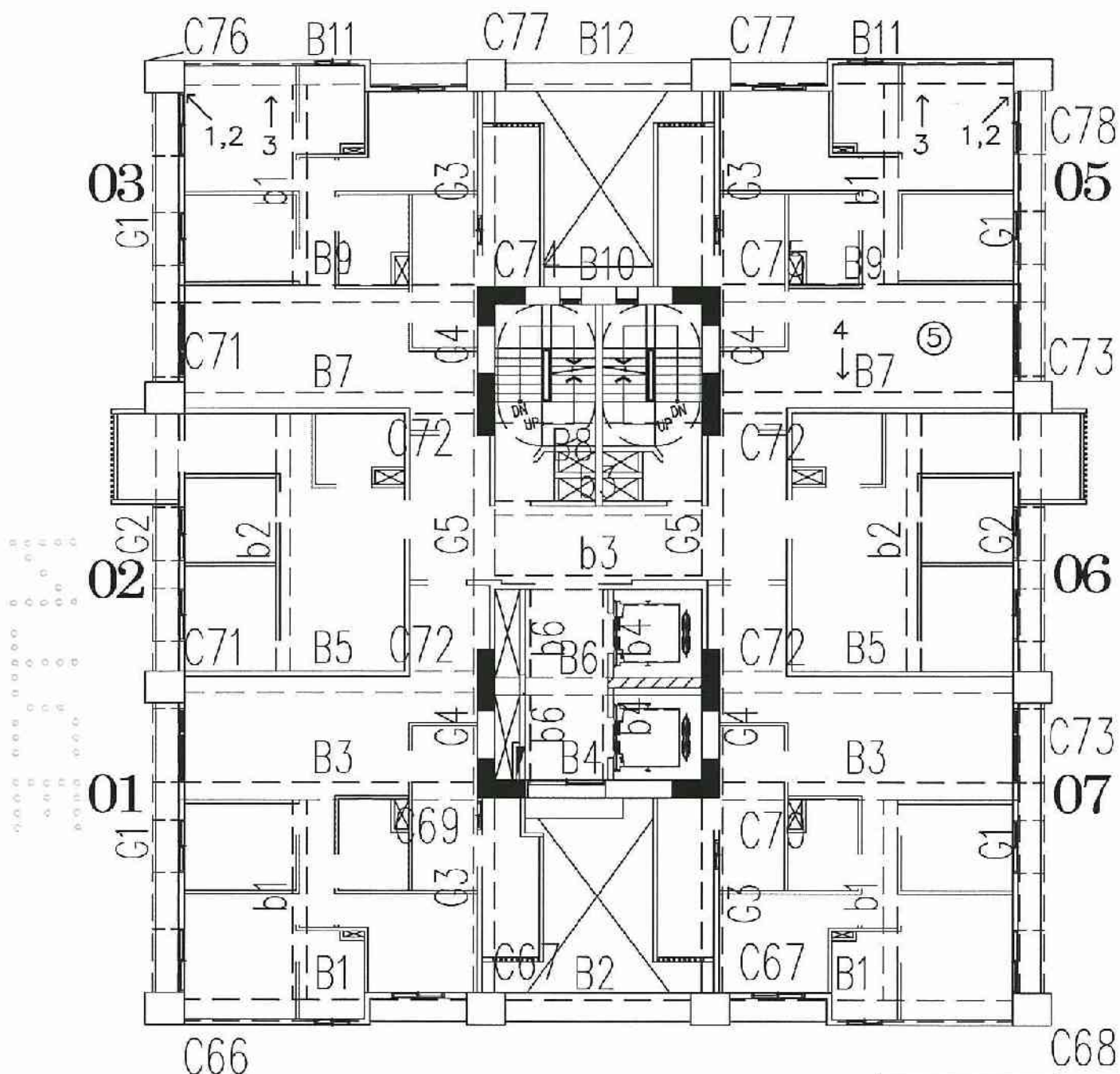
A6區B棟8層照片平面位置示意圖
