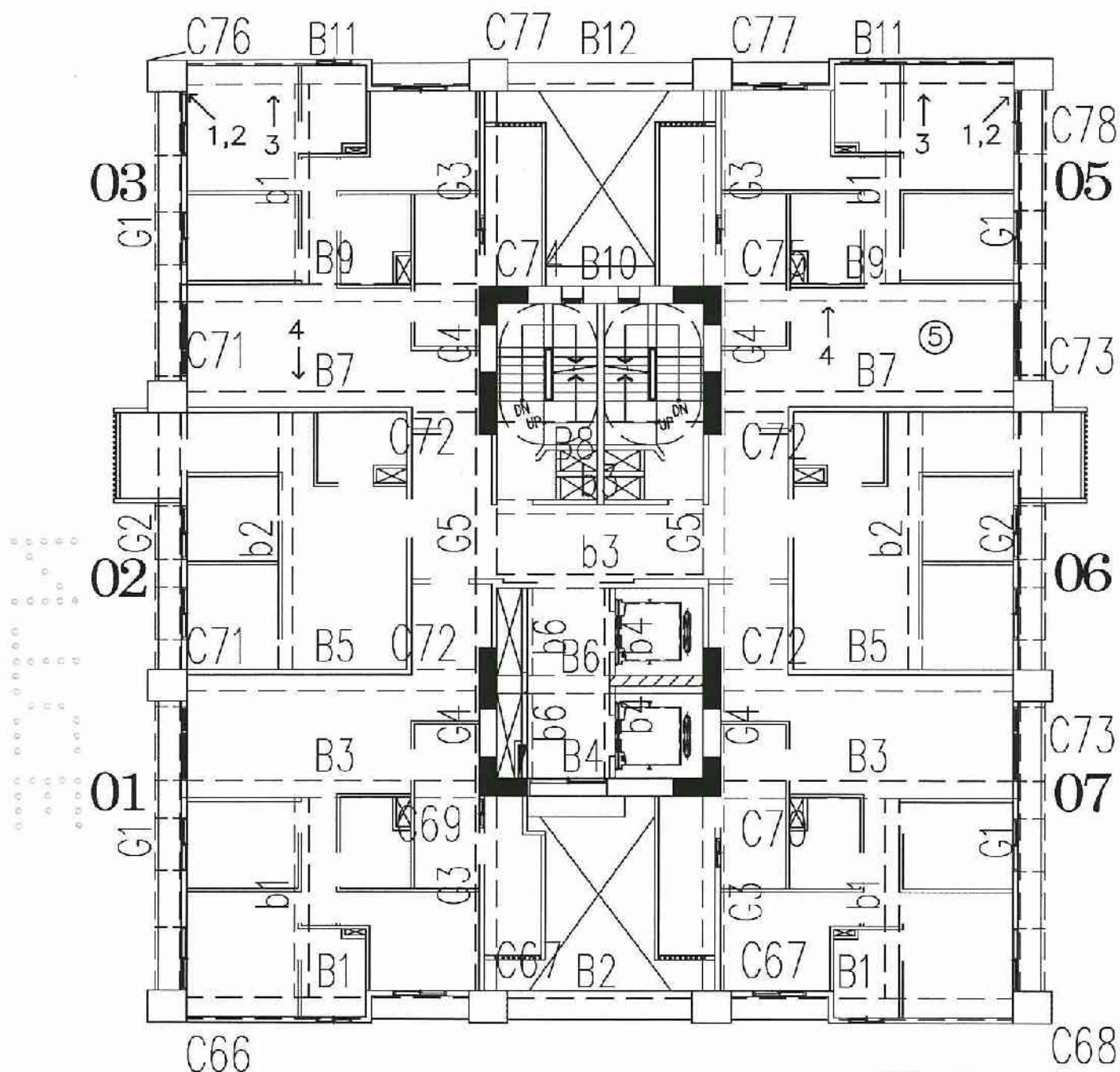
A6區B棟6層照片平面位置示意圖
