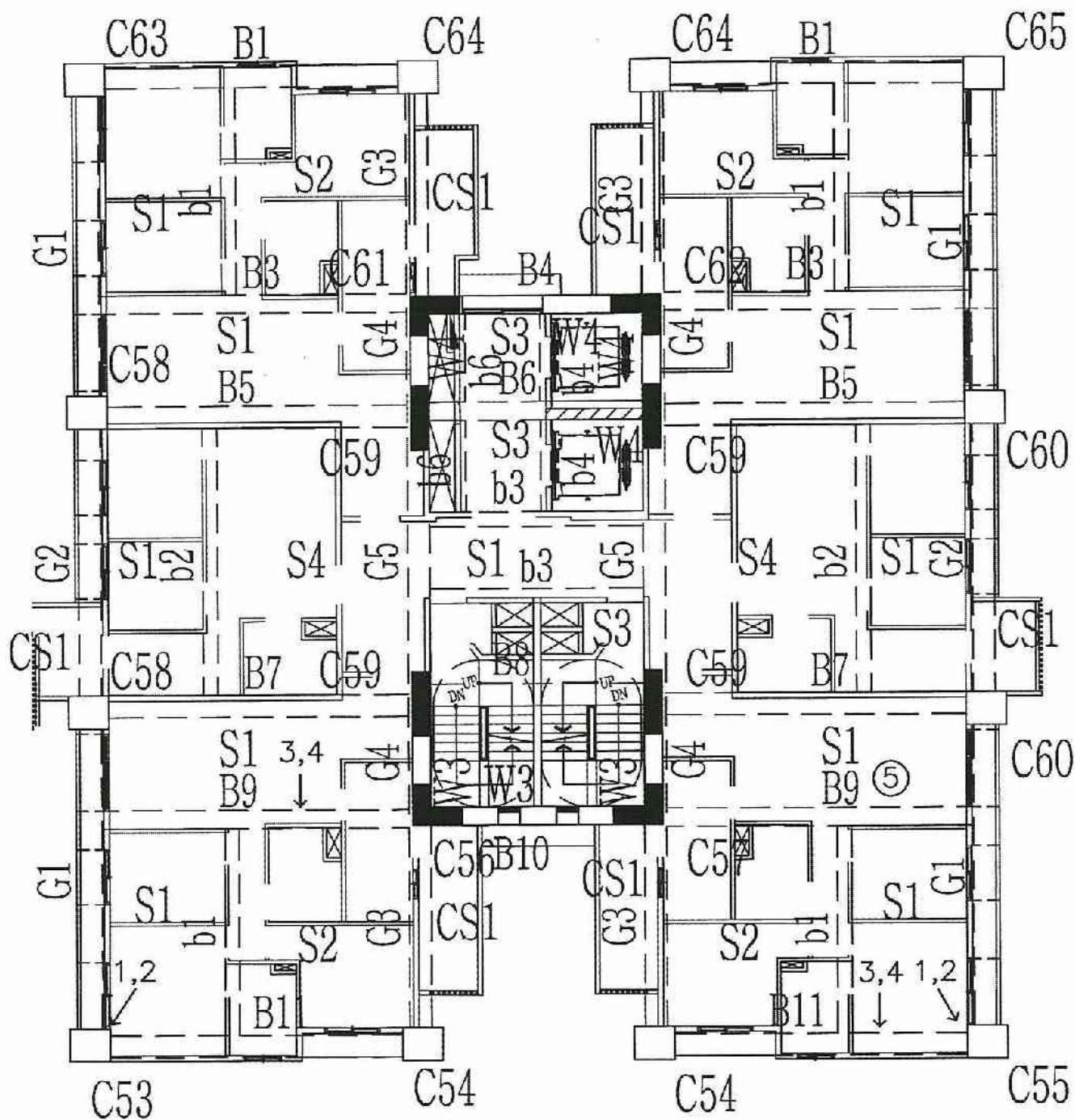
A6區C棟20層照片平面位置示意圖
