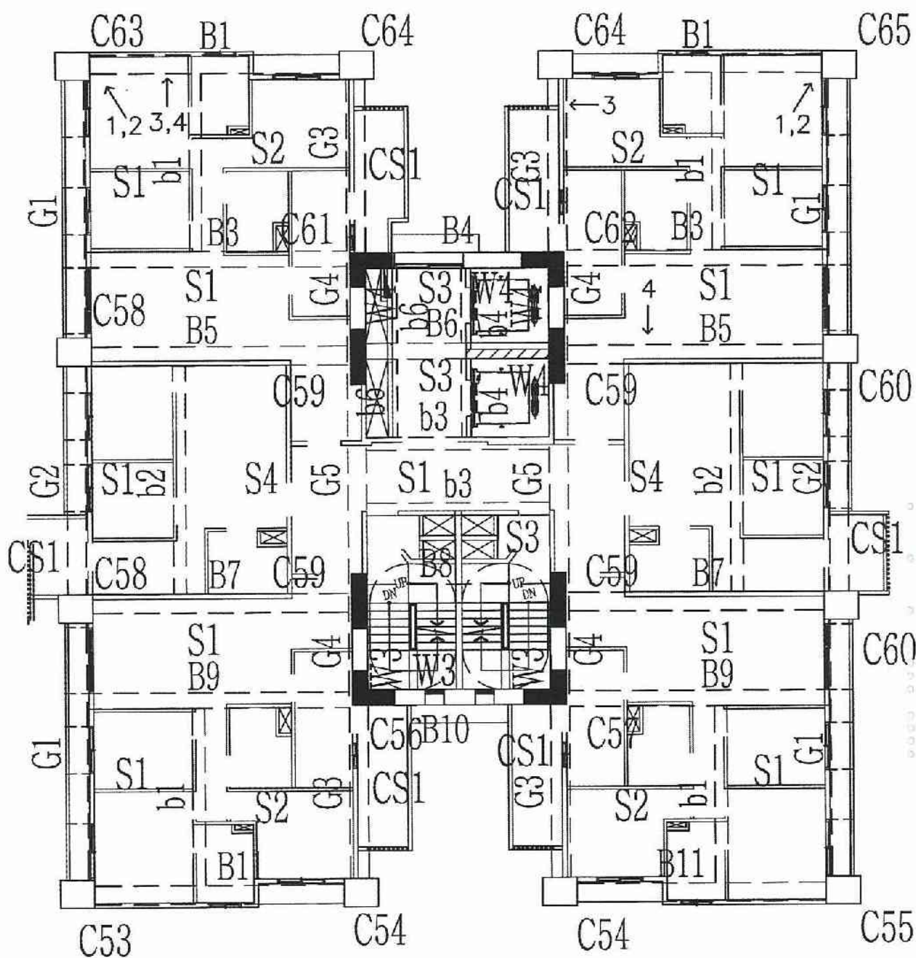
A6區C棟21層照片平面位置示意圖
