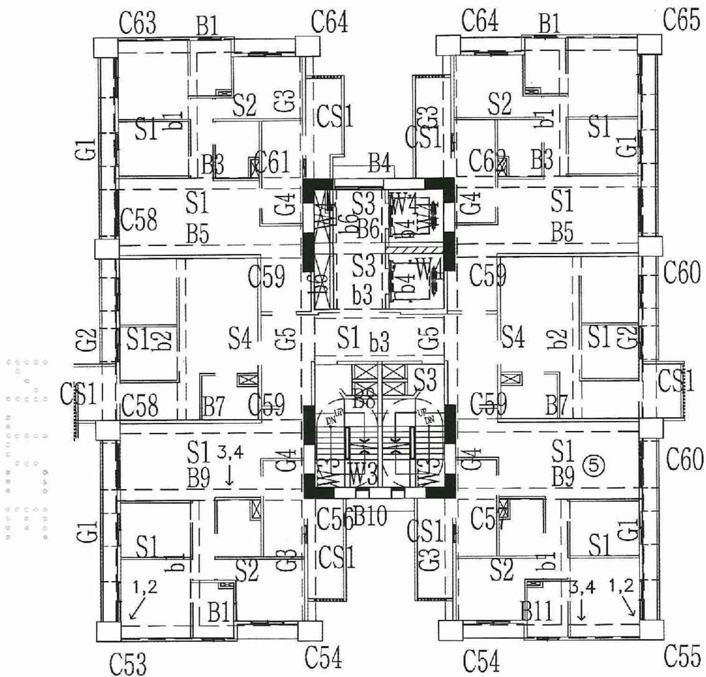
A6區C棟8層照片平面位置示意圖
