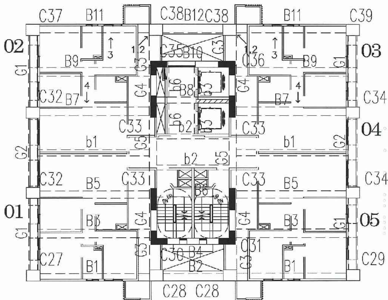
A6區D棟21層照片平面位置示意圖
