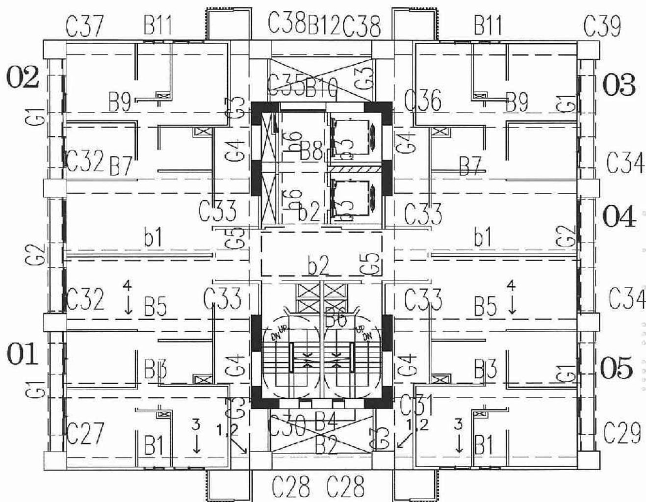
A6區D棟7層照片平面位置示意圖
