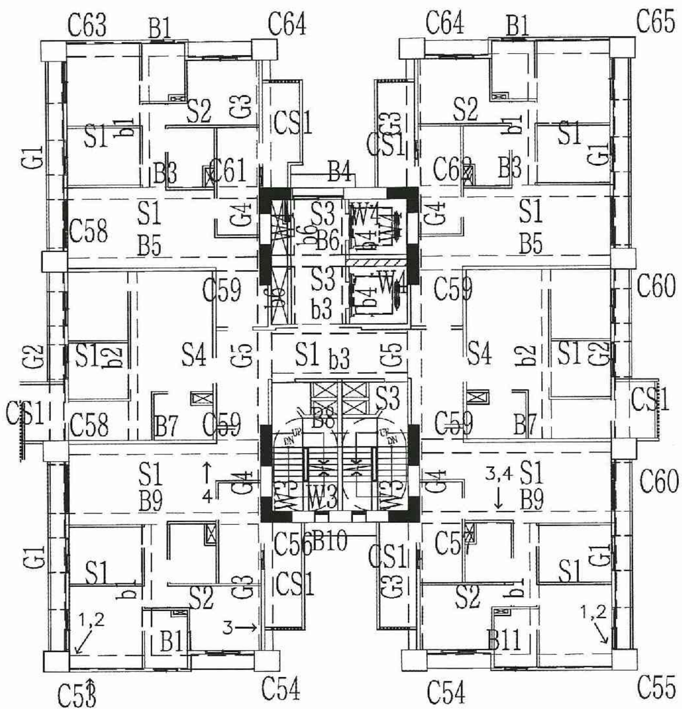
A6區C棟22層照片平面位置示意圖
