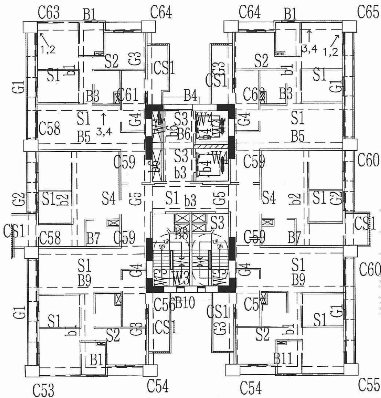
A6區C棟5層照片平面位置示意圖
