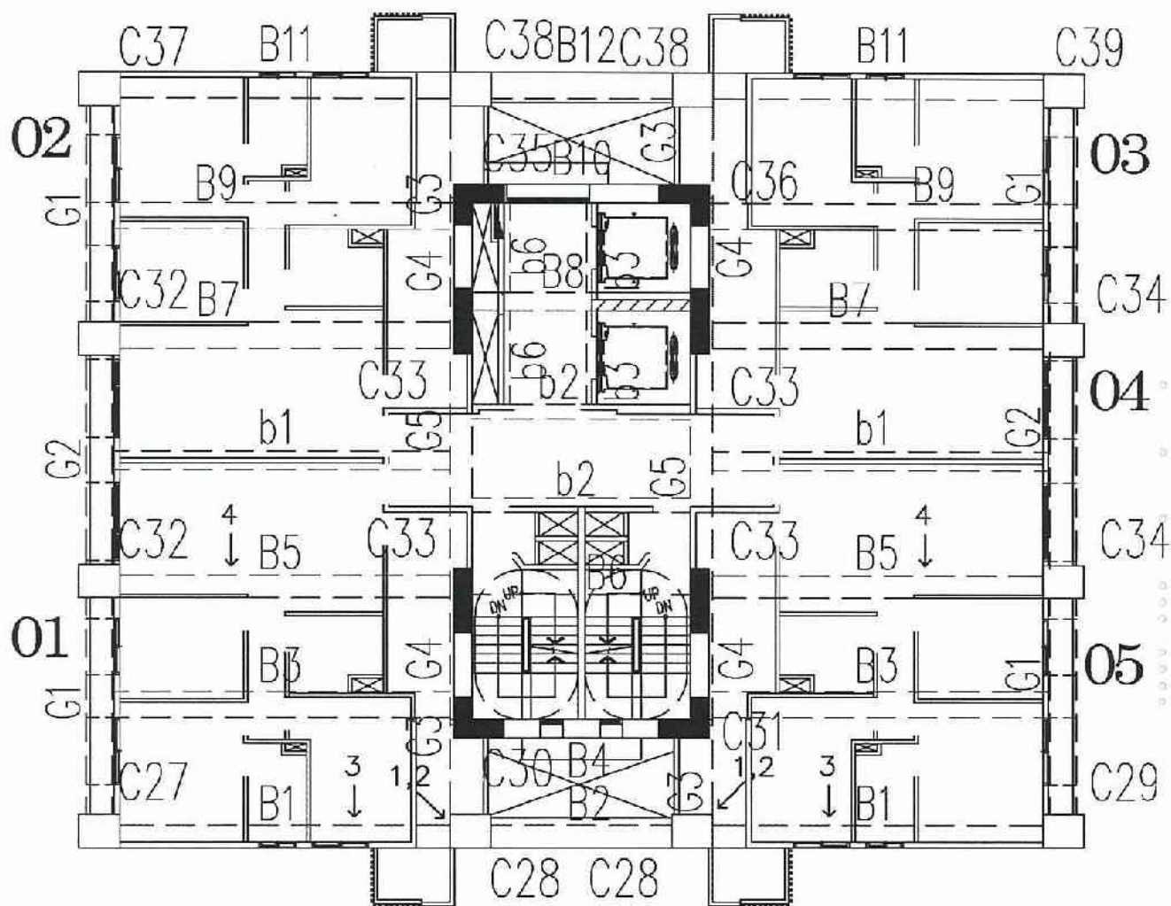
A6區D棟11層照片平面位置示意圖
