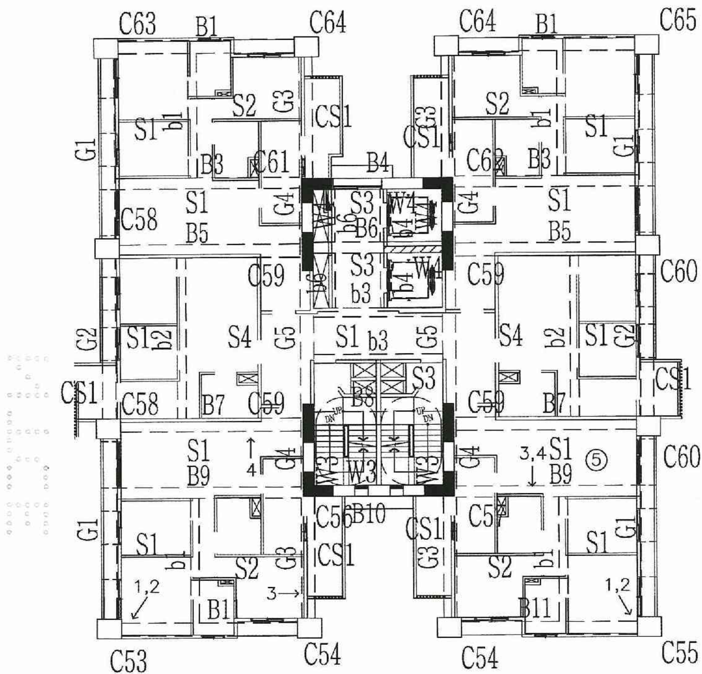
A6區C棟16層照片平面位置示意圖
