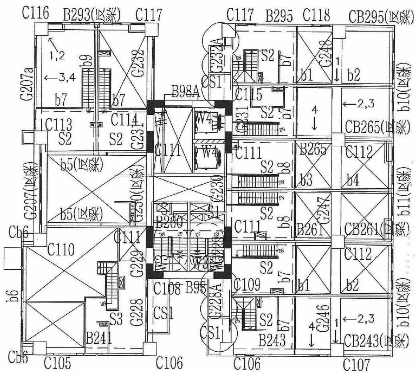
A6區A棟1層照片平面位置示意圖
