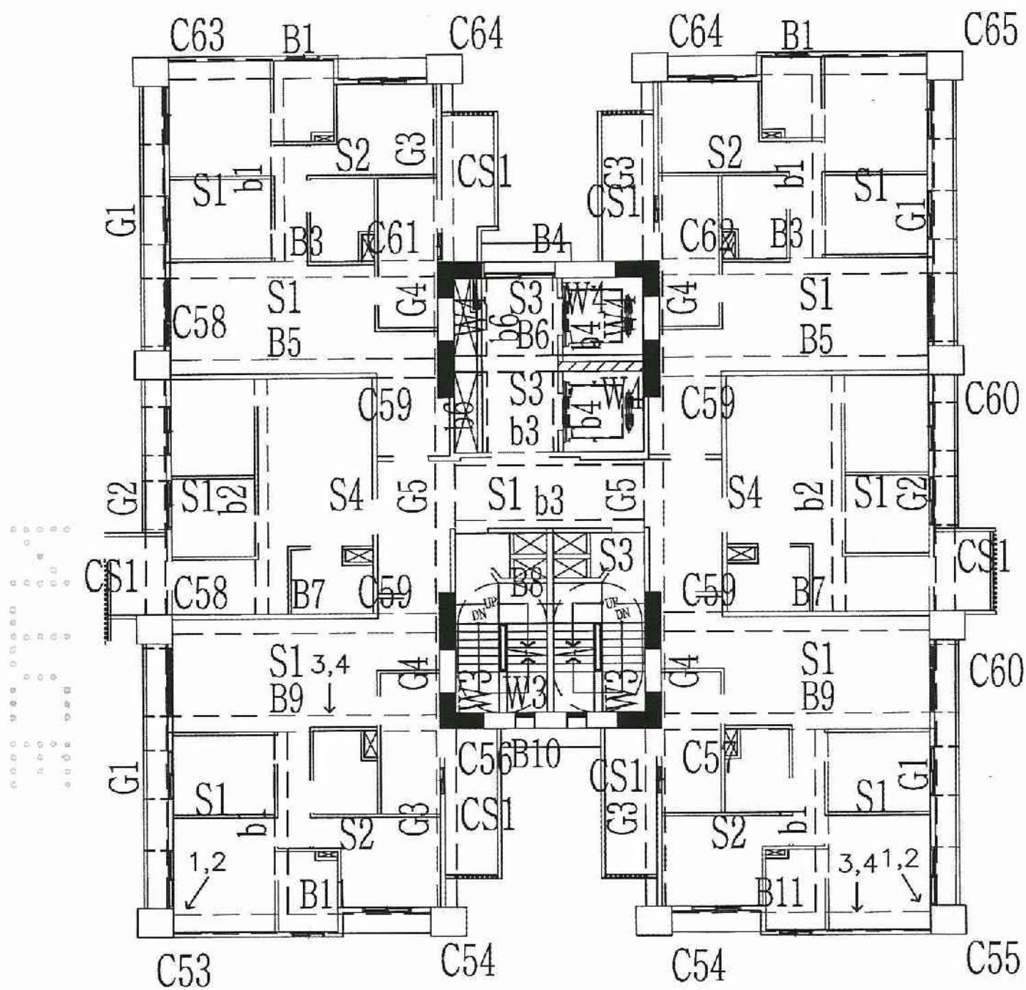
A6區C棟2層照片平面位置示意圖
