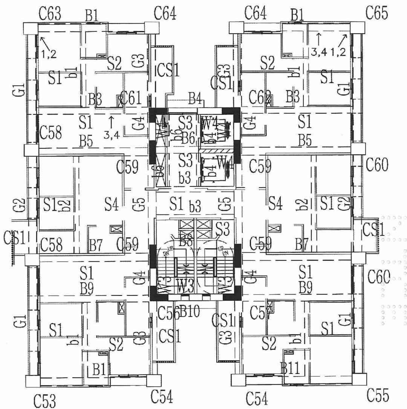
A6區C棟23層照片平面位置示意圖
