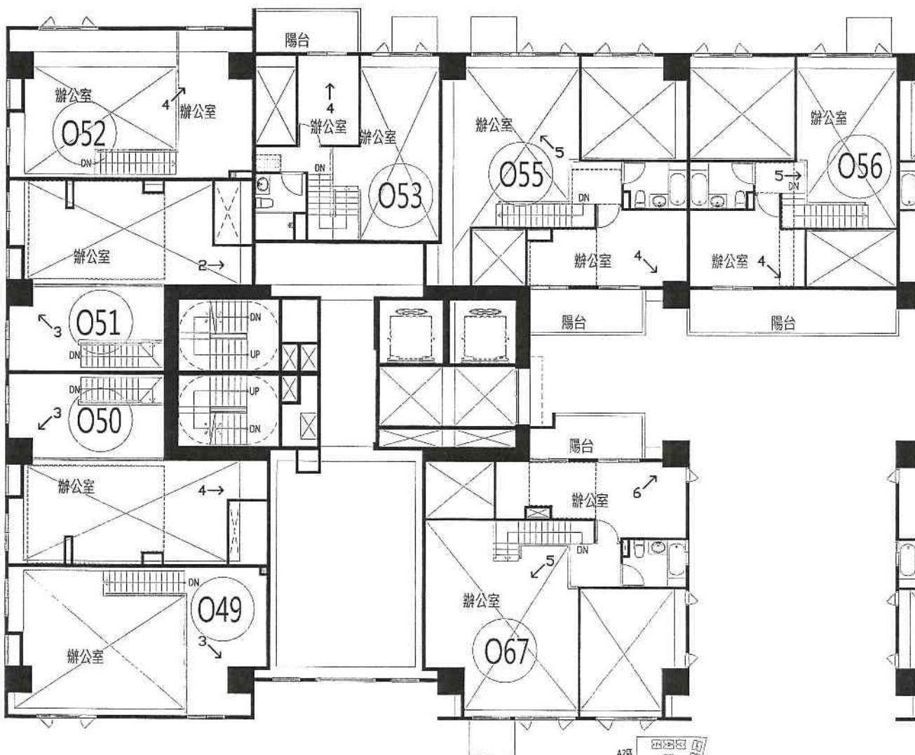
A6區S棟1層夾層照片平面位置示意圖
