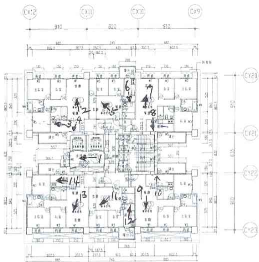
(Q棟) 3 層平面圖
