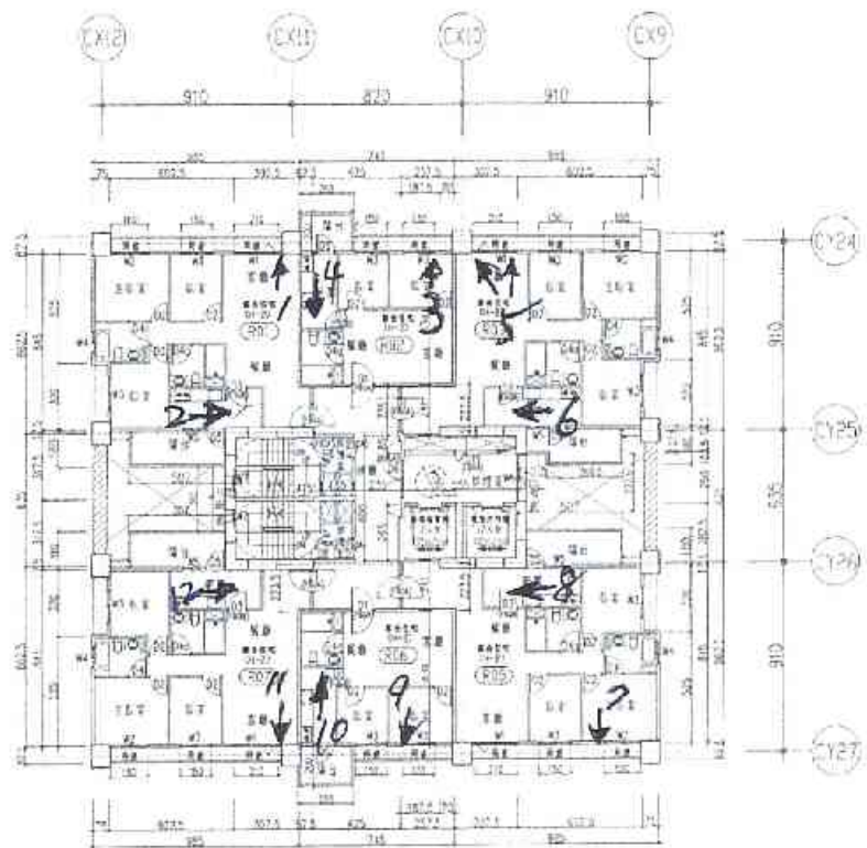
建築設計人建築面積(建築面積外計十七・二十・二十三層・詳註釋圖) (R棟) 18 層平面圖 A1 S=1/200 A3 S=1/400
