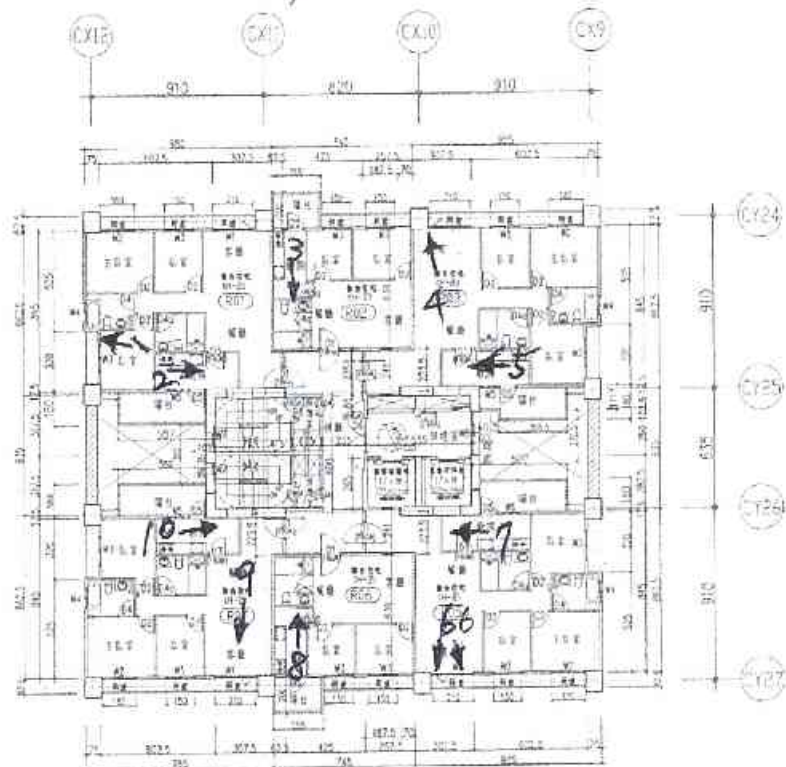
建築士事務所(建築士事務所) (R棟) 20 層平面圖 A1 S=1/200 A3 S=1/400
