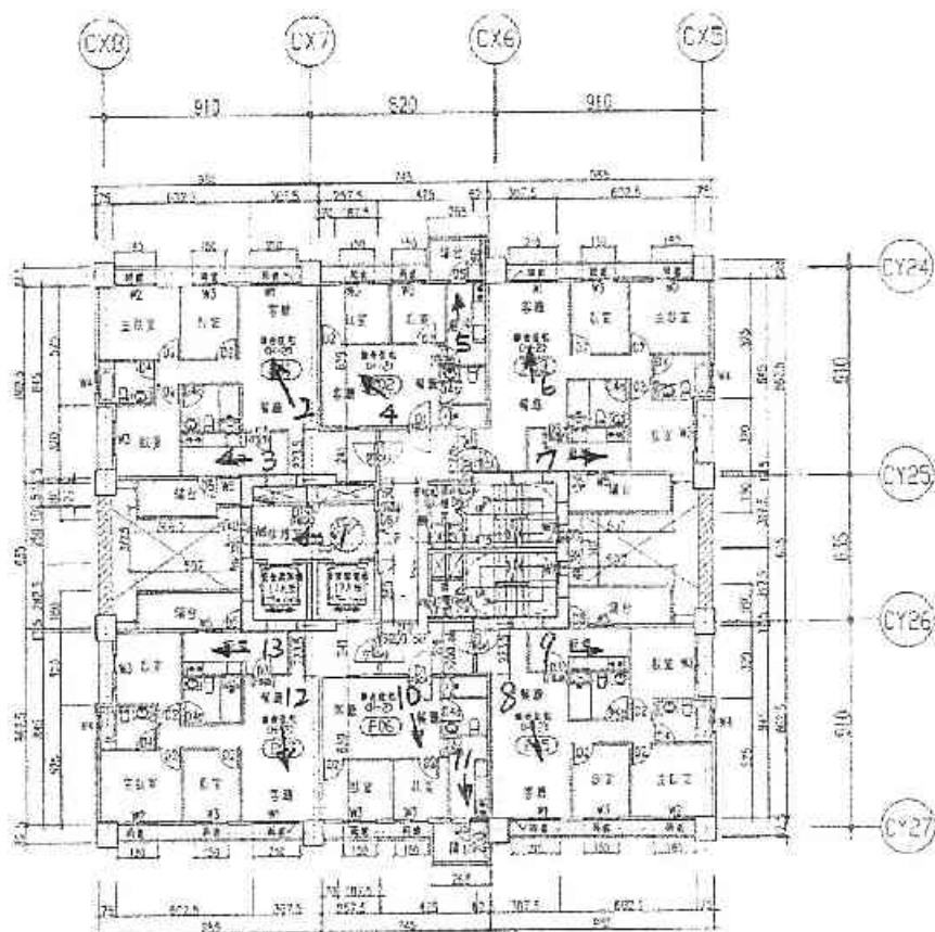
(P棟) 17 層平面圖 A1 S=1/200 A3 S=1/400
