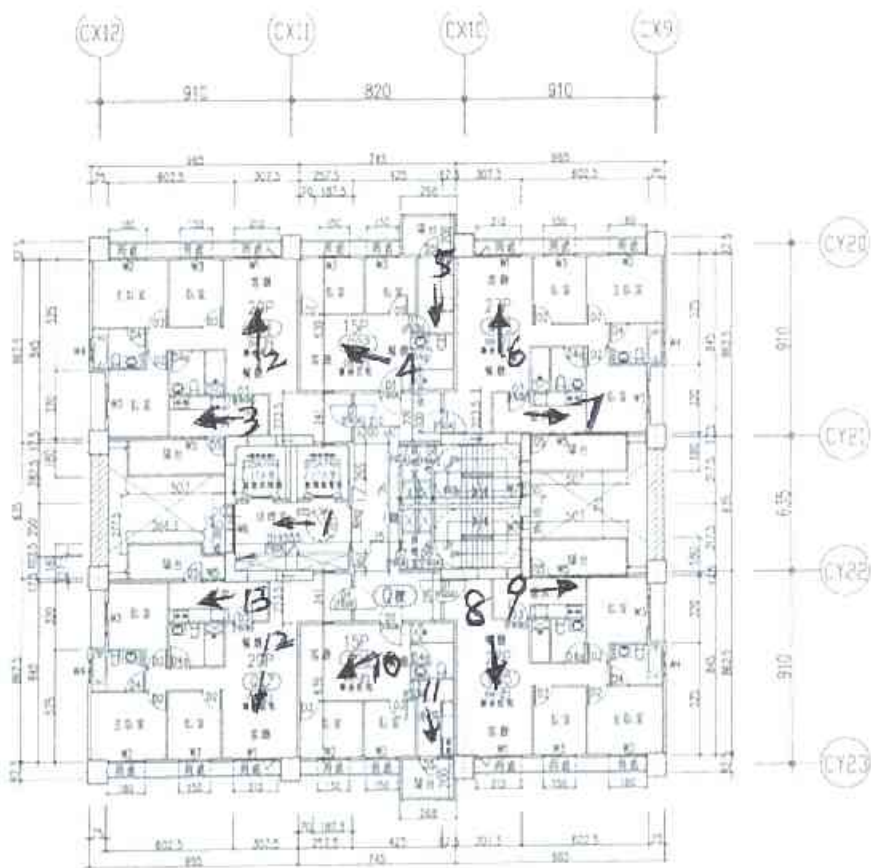
(Q棟) 4 層平面圖
