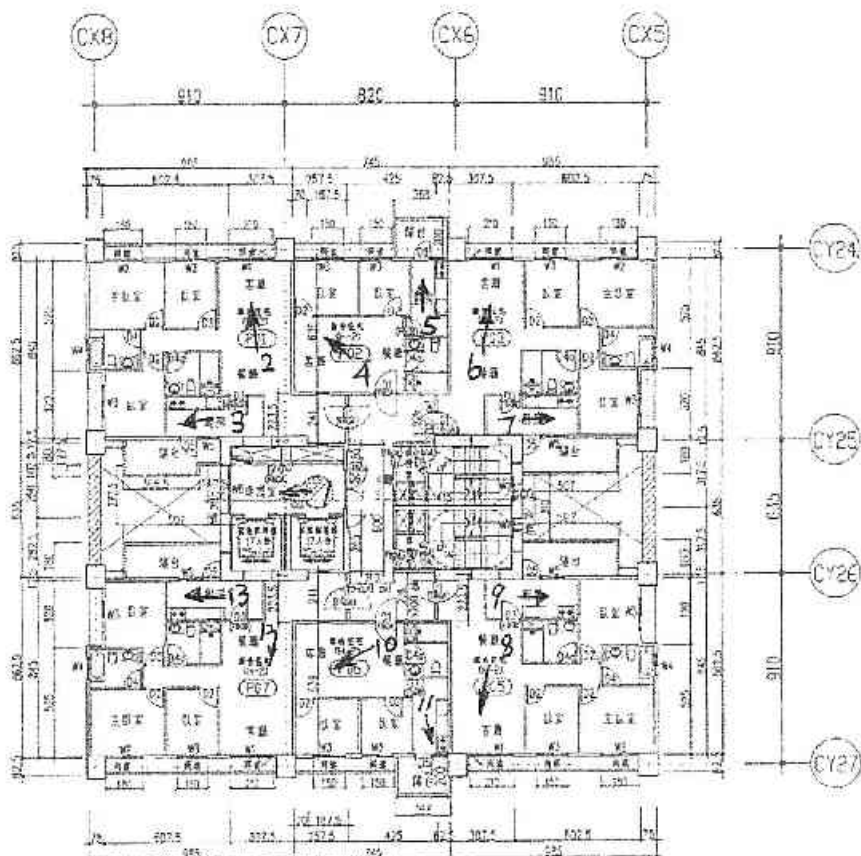
(P棟) 19 層平面圖 A1 S=1/200 A3 S=1/400
