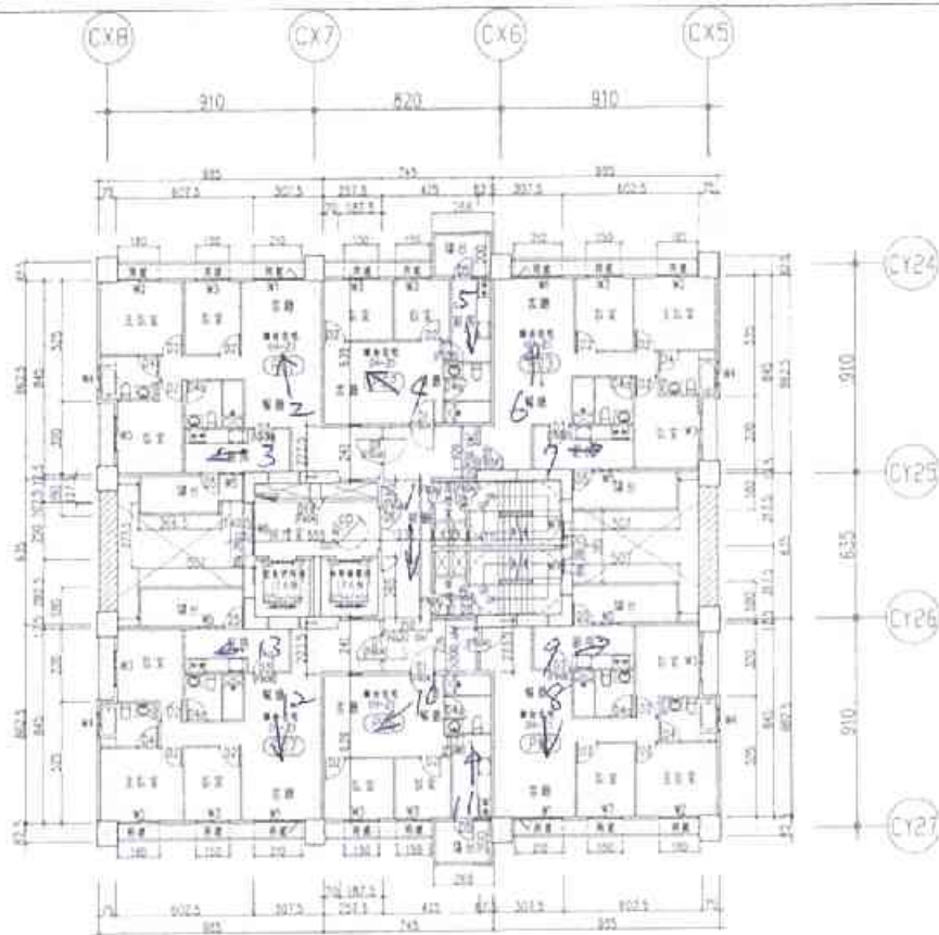
(P棟)3 層平面圖
