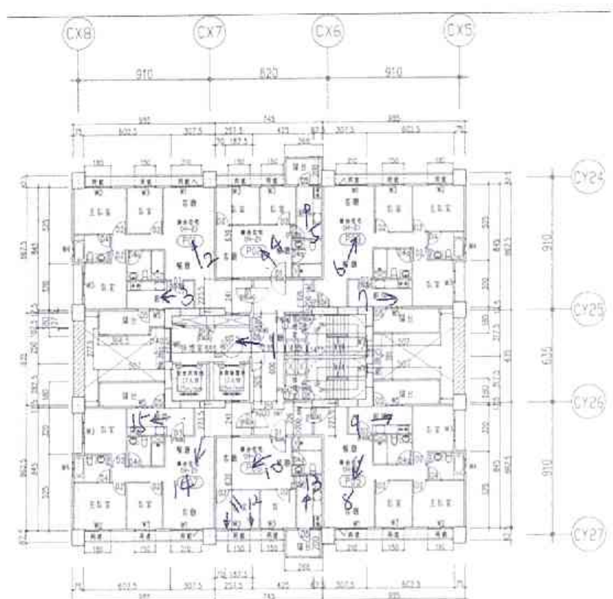
(P棟) 9 層平面圖 A1 S=1/200 A3 S=1/400
