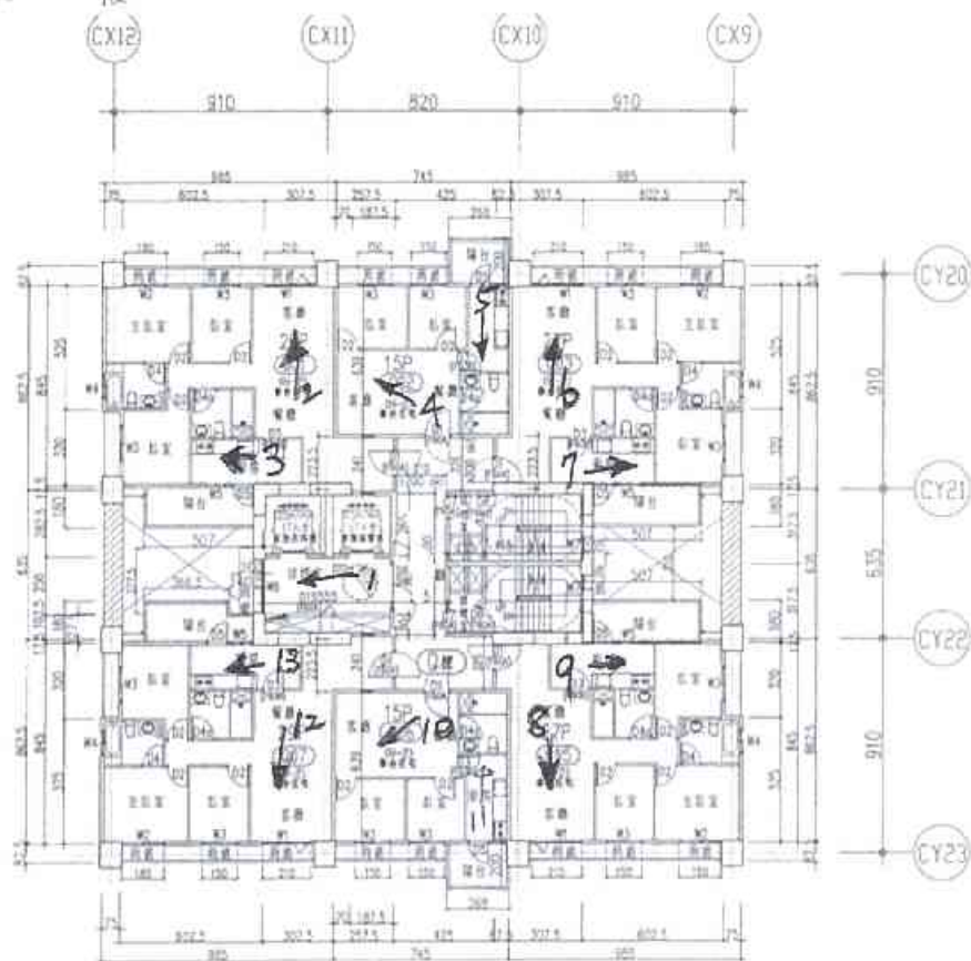
(Q棟) 13 層平面圖
