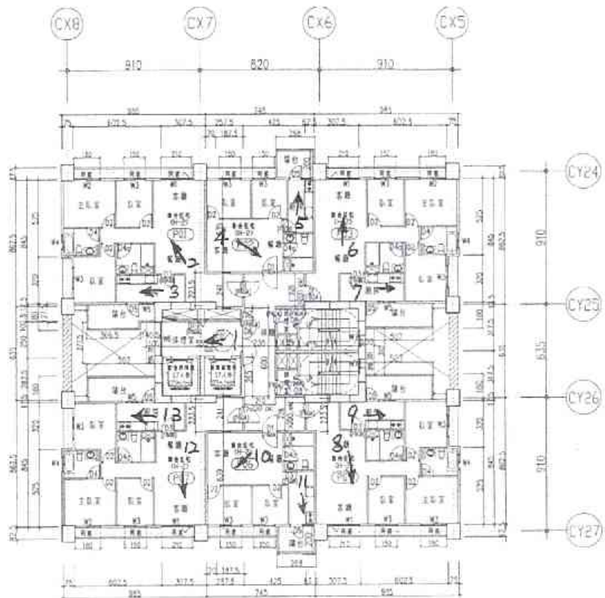
(P棟) 21 層平面圖 A1 S=1/200 A3 S=1/400
