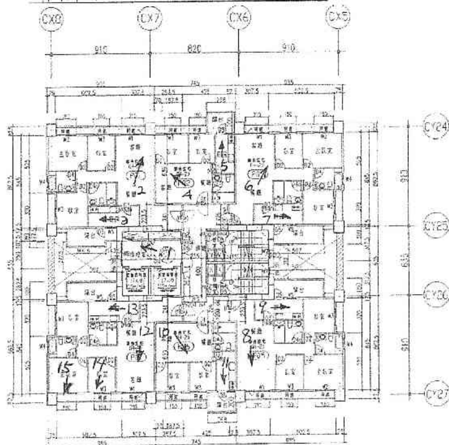
(P棟) 17 層平面圖 A1 S=1/200 A3 S=1/400
