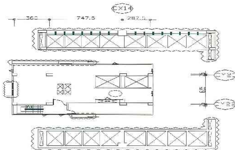
(S棟) 屋頂一層平面圖
