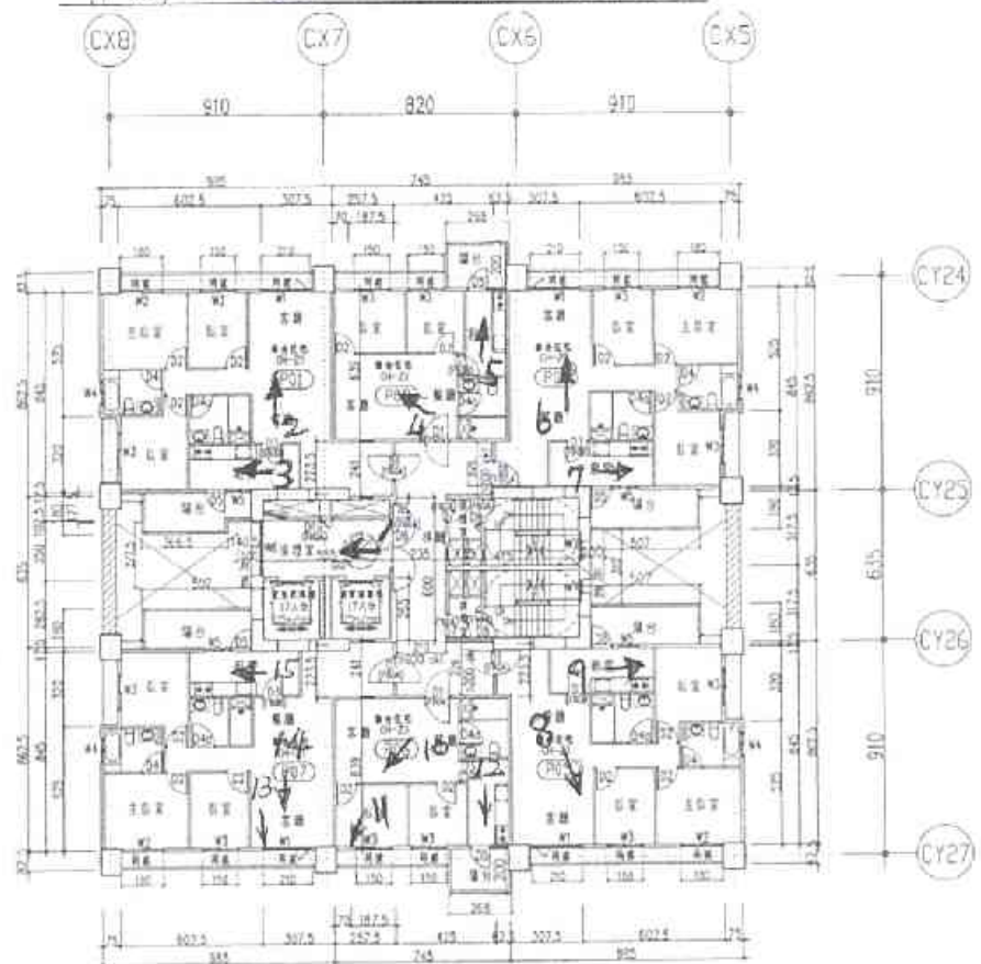
(P棟) 22 層平面圖 A1 S=1/200 A3 S=1/400
