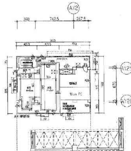
(F) 屋頂三層平面圖
