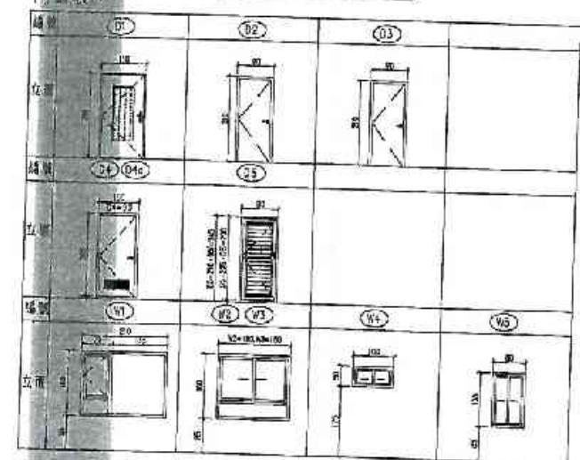
結構尺寸表：
