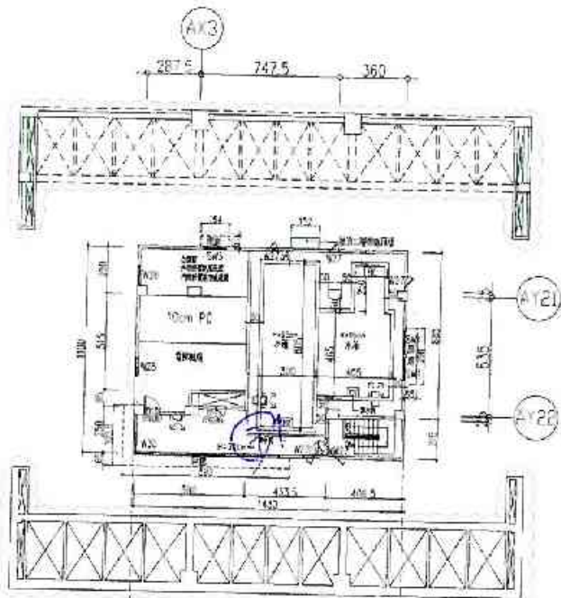
(E棟) 屋頂三層平面圖
