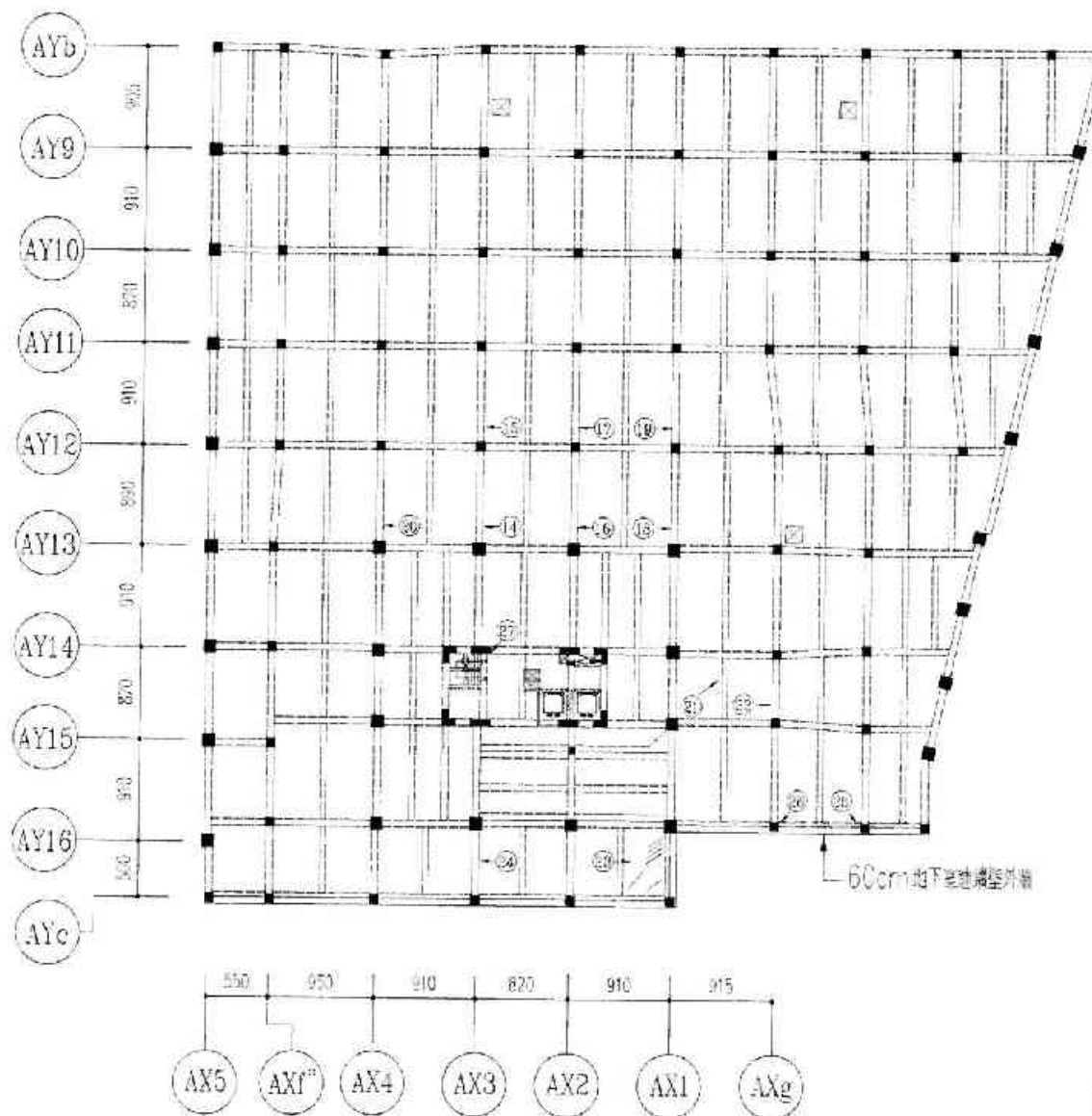
地下二層裂損照片編號平面圖 A6-2(圖F棟)
