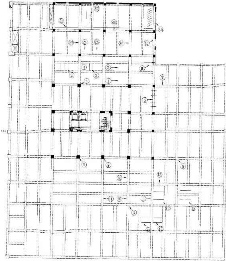
一層裂損照片編號平面圖
