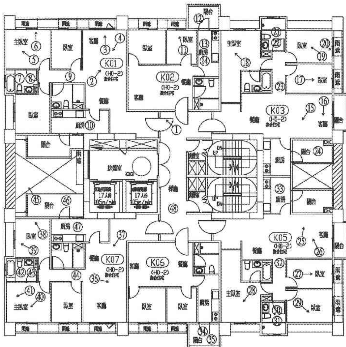
四層平面圖
