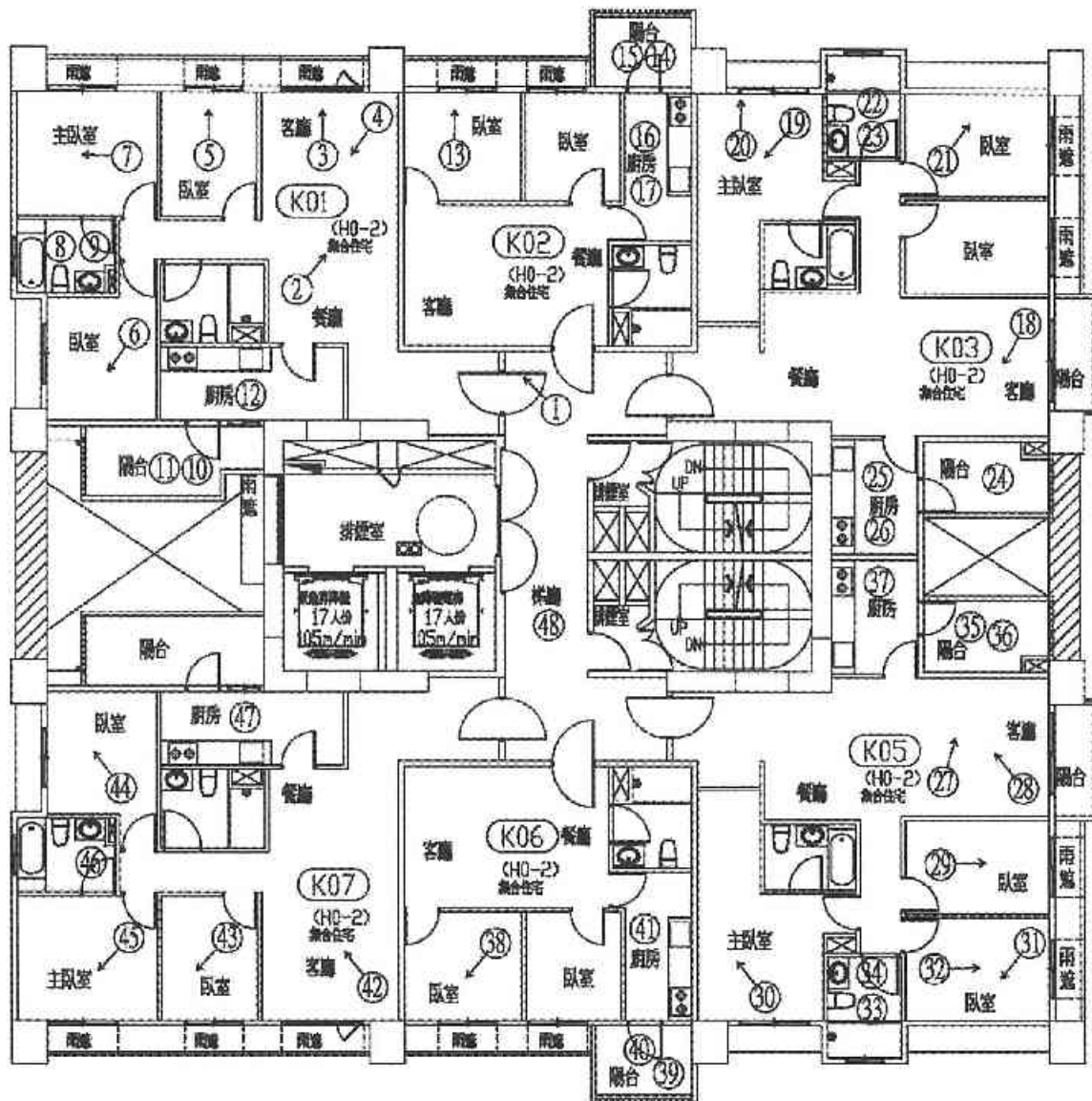
五層平面圖 照片編號：○ A6區K棟
