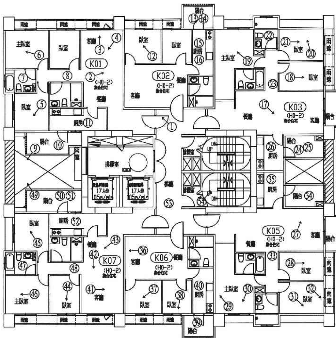
七層平面圖 照片編號：○ A6區K棟
