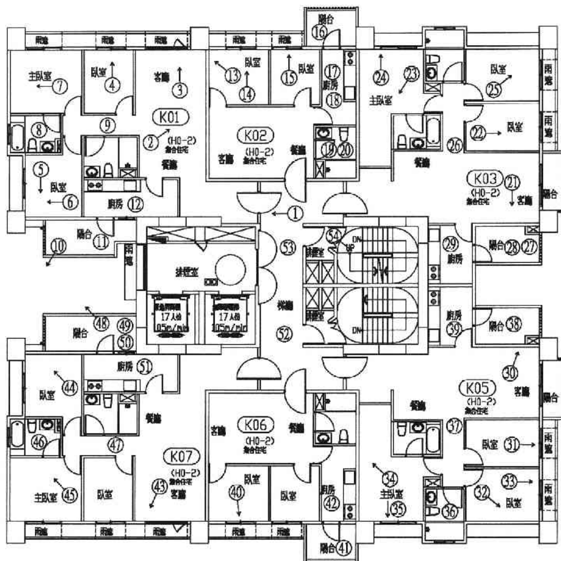
二十一層平面圖 照片編號：○ A6區K棟
