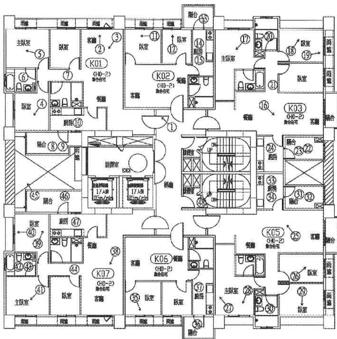
六層平面圖 照片編號：○ A6區K棟
