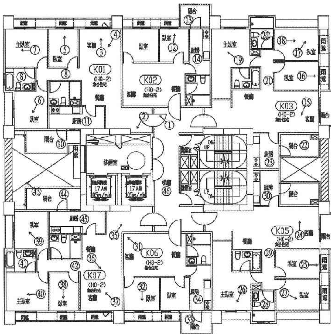
二十層平面圖 照片編號：○ A6區K棟
