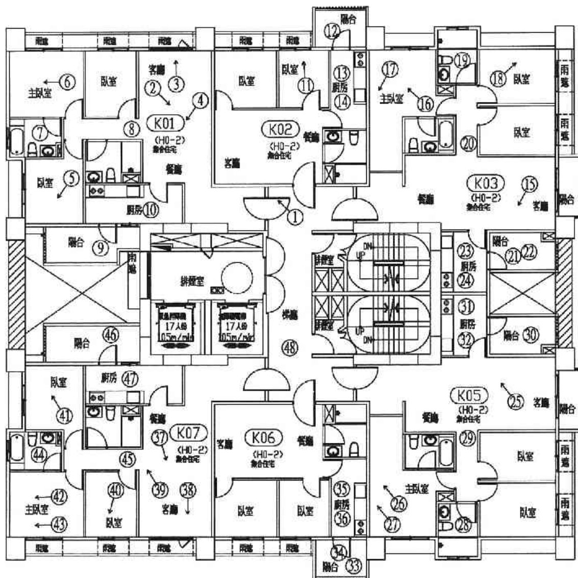
八層平面圖 照片編號：○ A6區K棟
