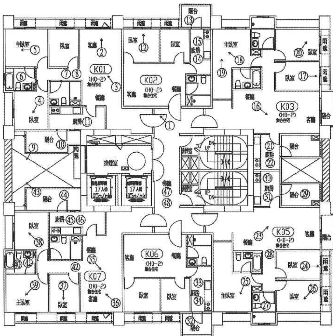
十八層平面圖 照片編號：○ A6區K棟
