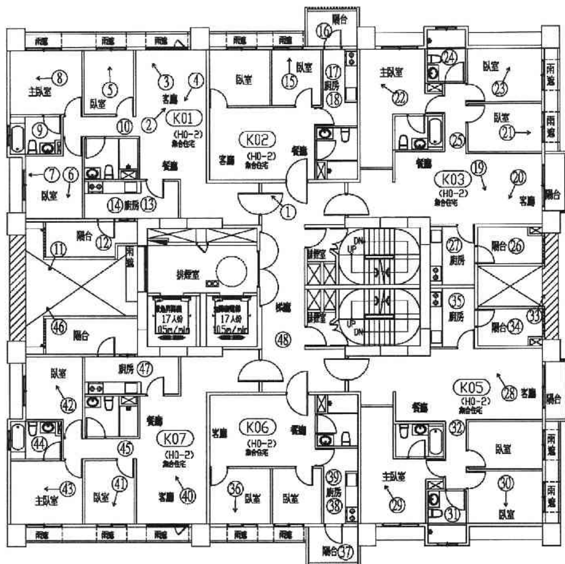
十三層平面圖 照片編號：○ A6區K棟
