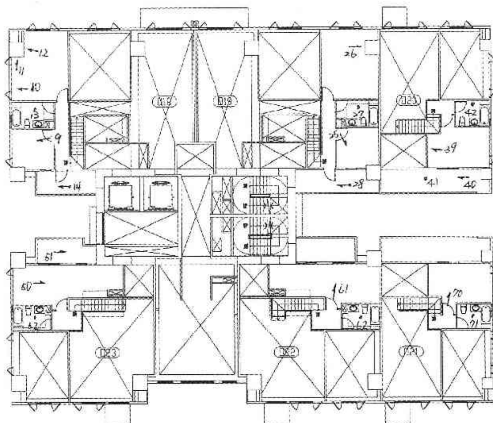
(E棟) 夾層平面圖
