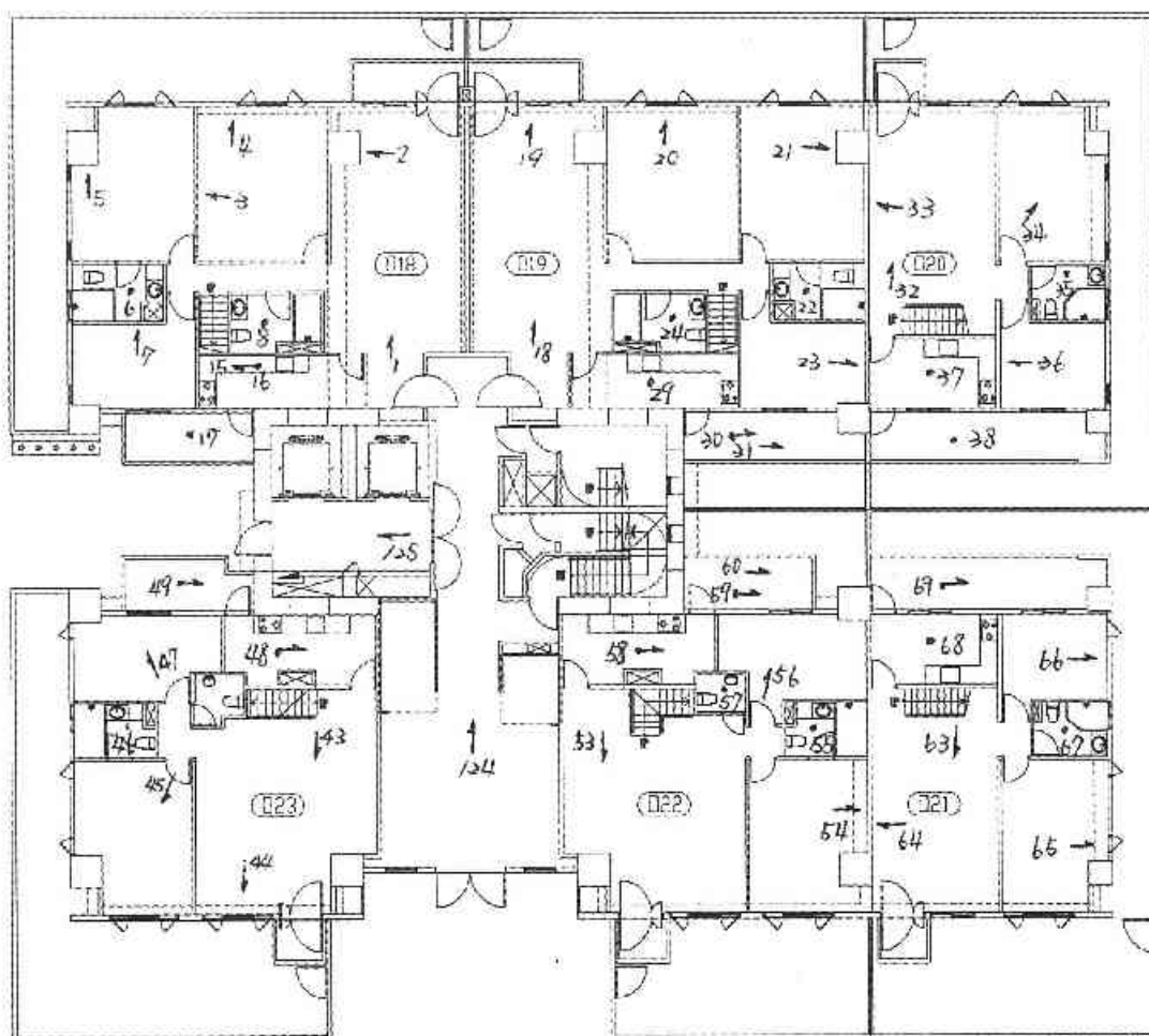
(E棟) 一層平面圖
