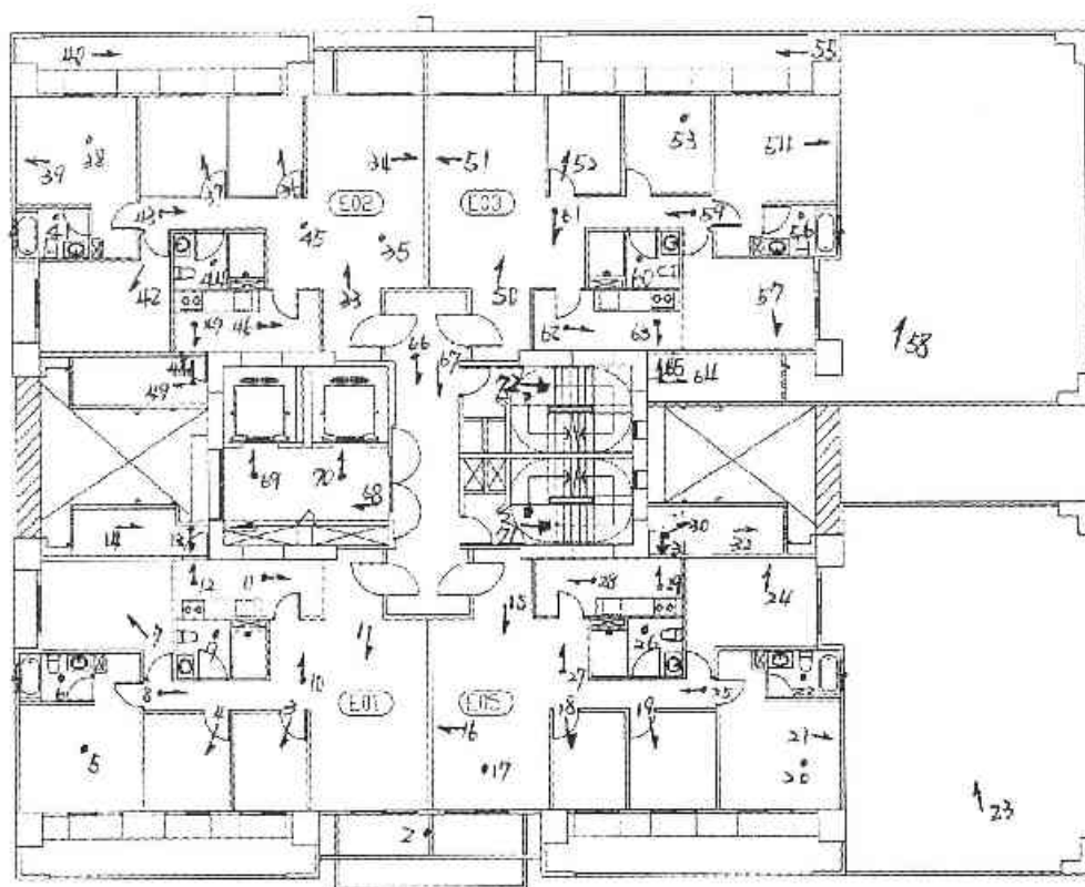
(E棟) 二層平面圖
