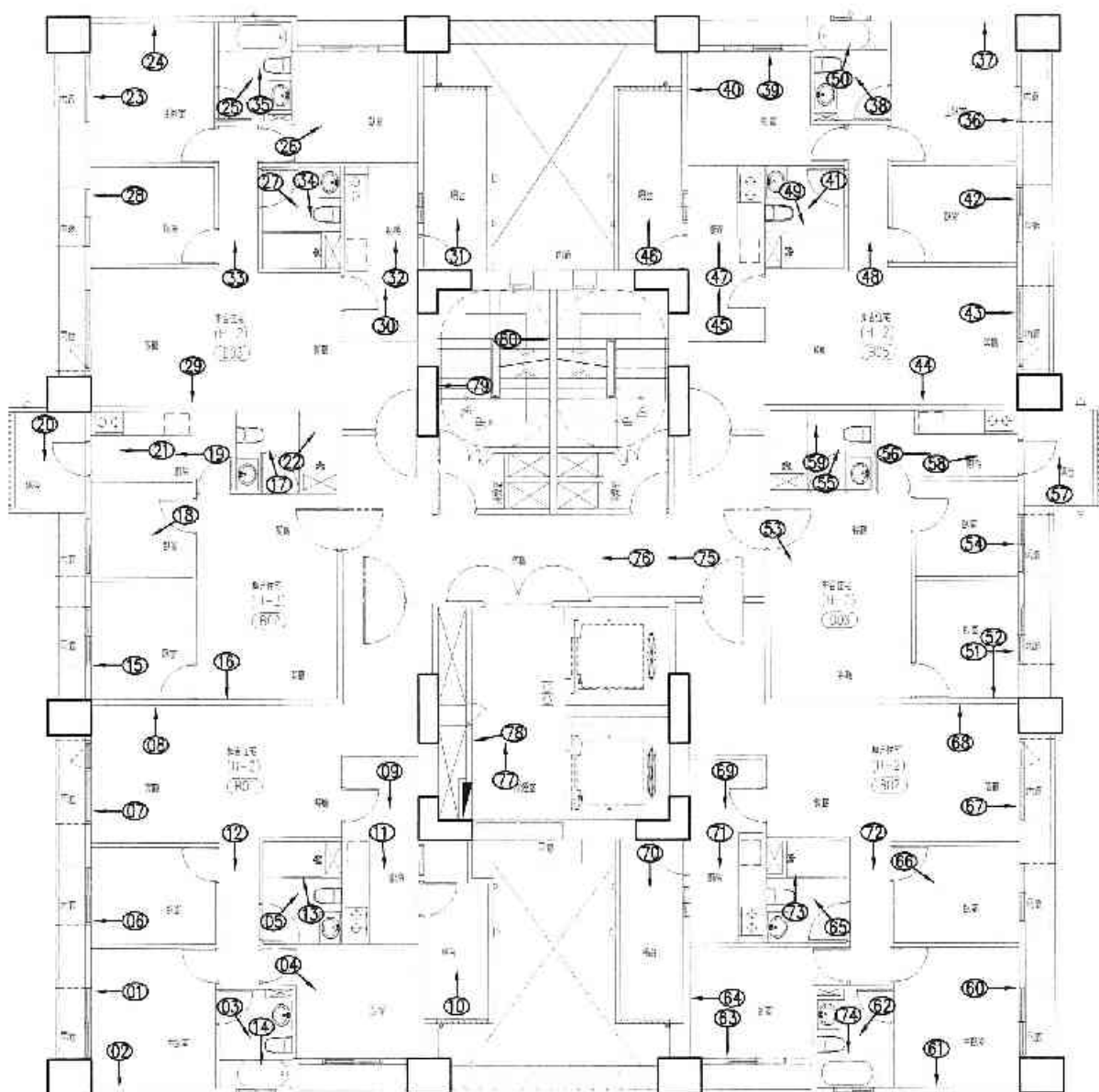
B棟 十五層平面圖(十六層結構)
