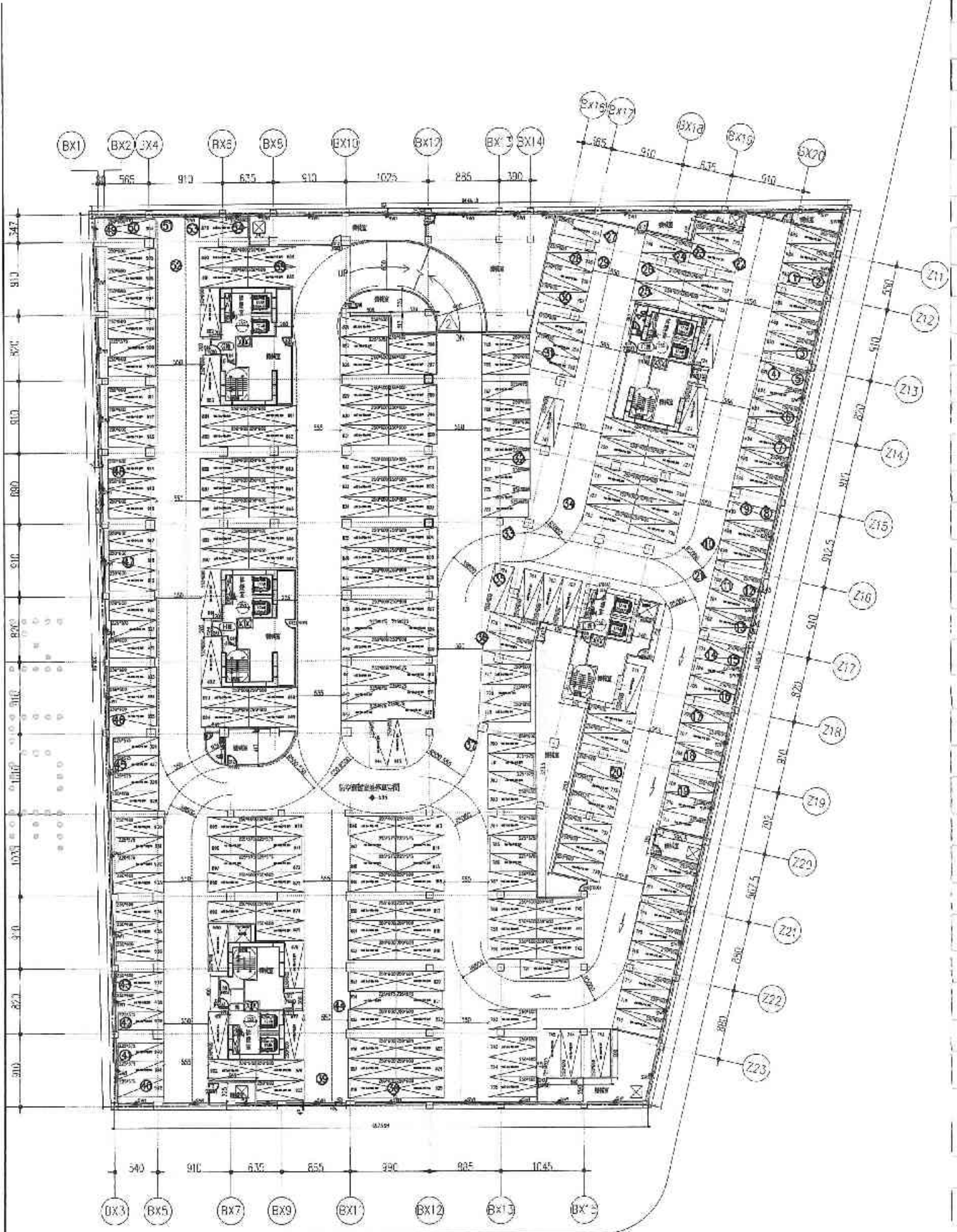
A3 II 地下二層現況位置示意圖
